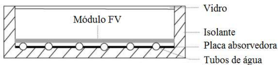
Figura 16. Corte transversal de um coletor solar híbrido PVT básico
