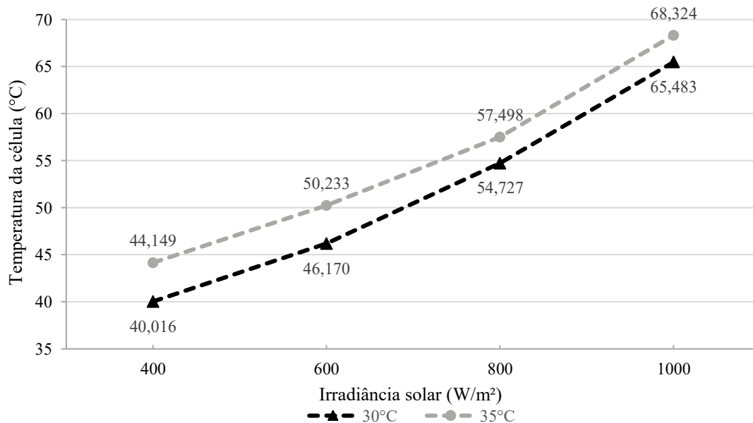
Figura 63. Temperatura da célula fotovoltaica em função da irradiância solar Fonte: Elaboração própria
