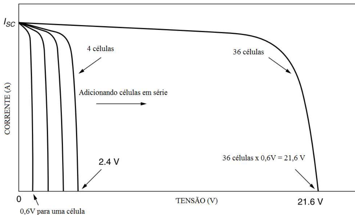
Figura 10. Células ligadas em série, suas tensões para determinados níveis de corrente Fonte: Adaptado de MASTERS (2004)
