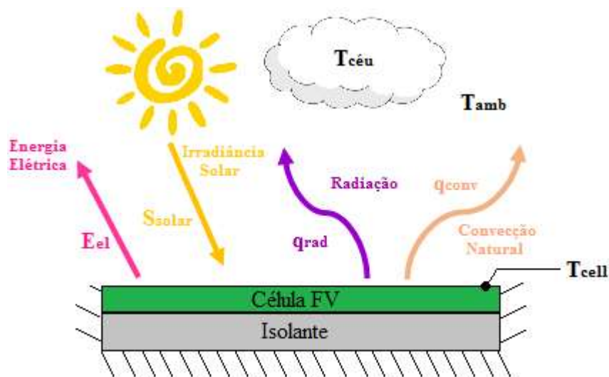
Figura 35. Esquema do Modelo Térmico 1
