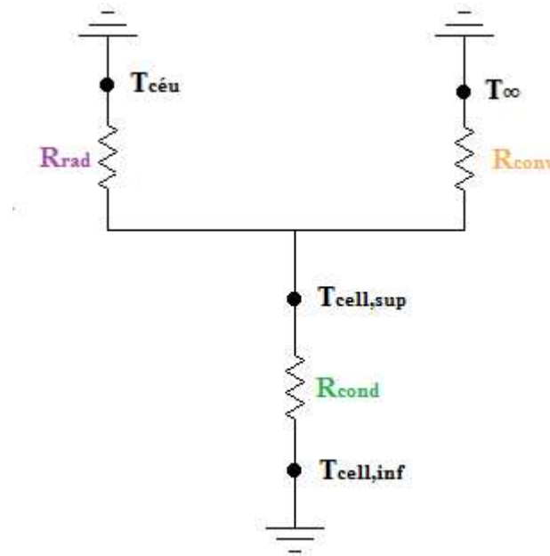
Figura 36. Diagrama de resistências do Modelo Térmico 1 Fonte: Autoria própria
