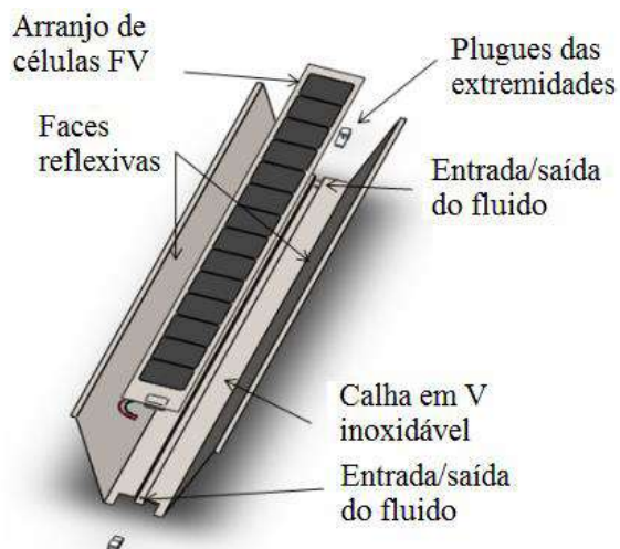
Figura 27. Detalhe de uma calha em V de um BIPVTC Fonte: Adaptada de Künnemeyer et al. (2011)
