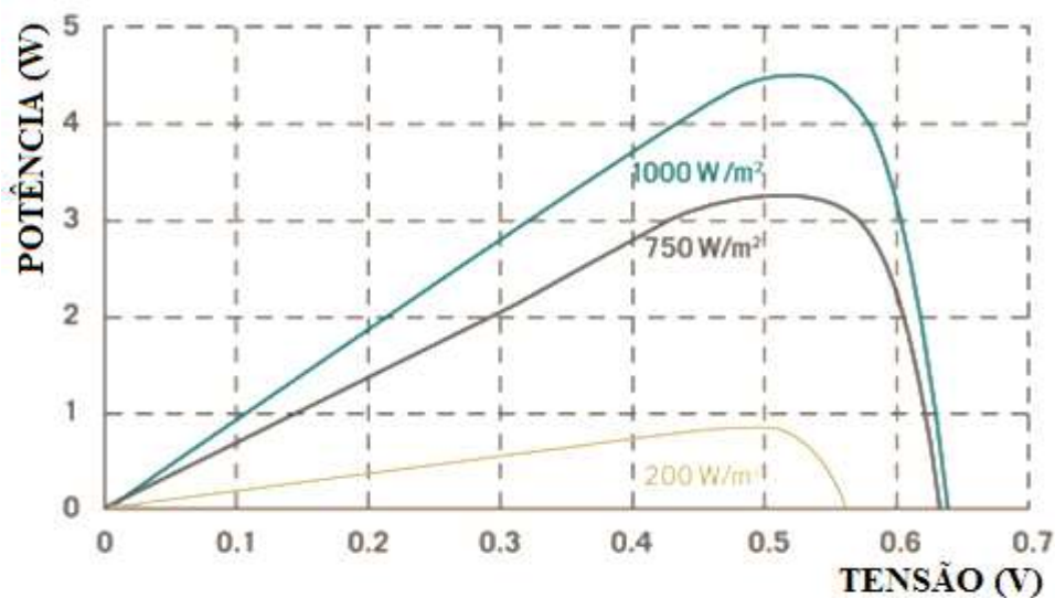
Figura 32. Curva característica P-V da célula em estudo Fonte: Adaptado de Q CELLS (2013)
