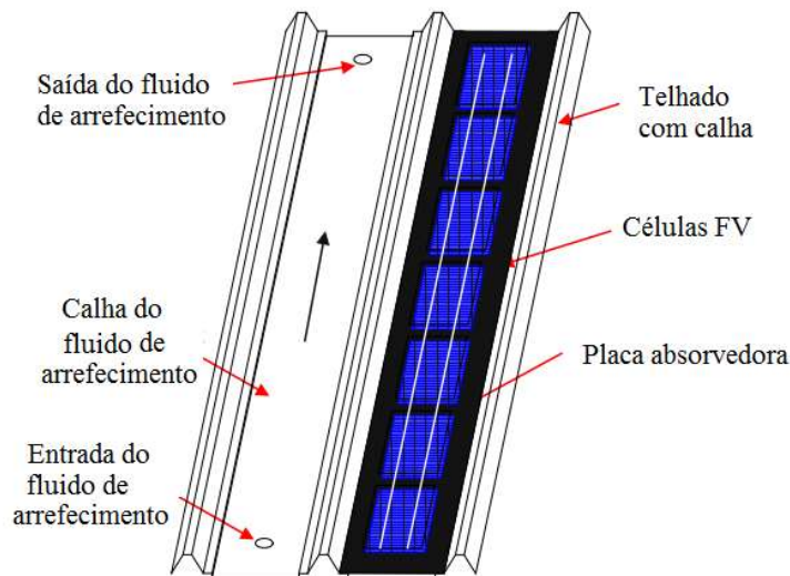
Figura 26. Coletor BIPVT Fonte: Adaptada de ANDERSON et al. (2009)
