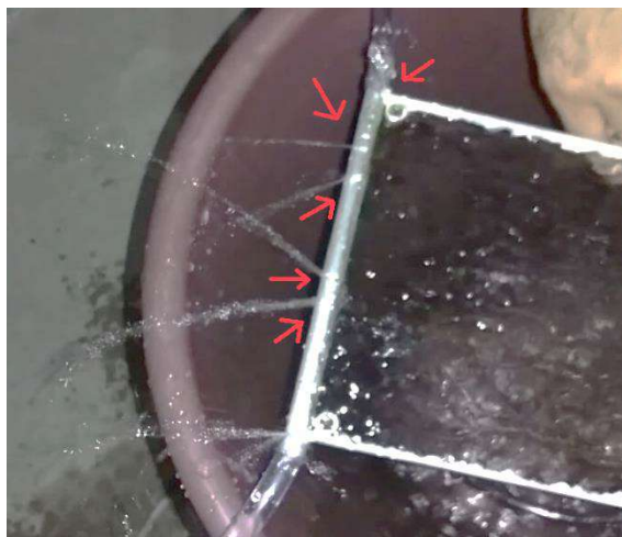
Figura 44. Pontos de vazamento da camada vidro-vidro
