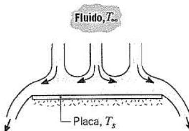
Figura 73. Escoamentos movidos pelo empuxo em placas horizontais com face superior fria
