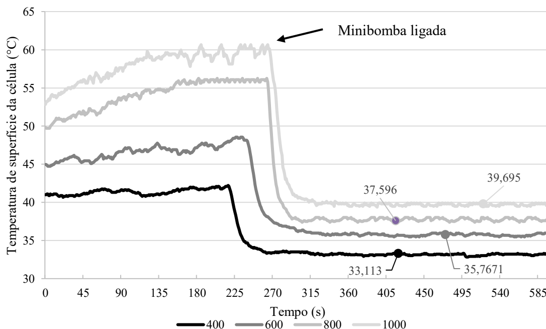
Figura 67. Comportamento da temperatura de superfície da célula FV com arrefecimento
