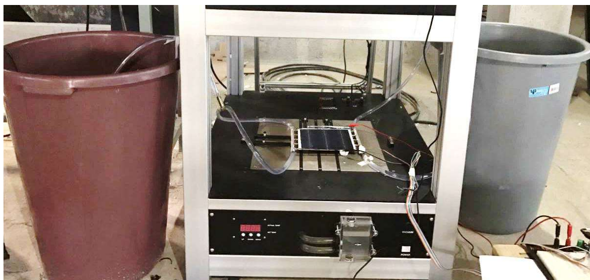
Figura 51. Protótipo 1 sem a camada vidro/vidro Fonte: Autoria própria
