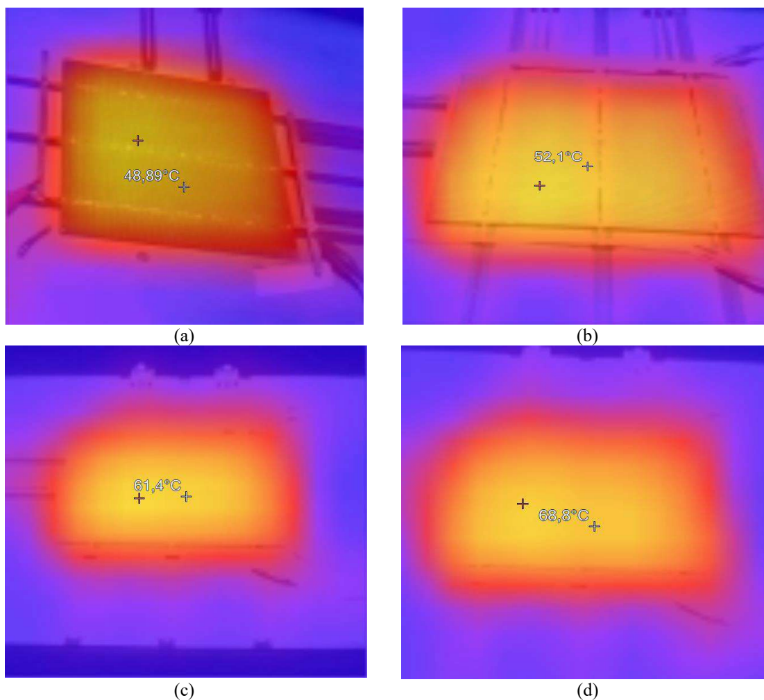
Figura 65. Mapa de calor da célula FV para temperatura ambiente de 35°C e irradiância de (a) 400W/m², (b) 600W/m², (c) 800W/m² e (d) 1000W/m² Fonte: Autoria própria
