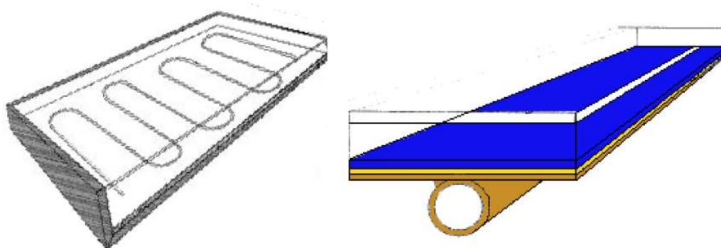
Figura 25. Coletor PVT real com tubos em serpentinas (esquerda) e coletor PVT com tubos retilíneos utilizado nos modelos numéricos (direita)
