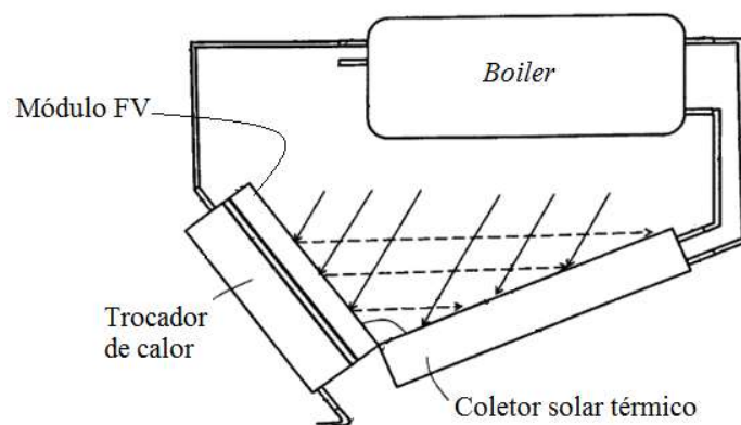
Figura 28. Visão global do sistema híbrido com destaque nos quatro principais elementos
