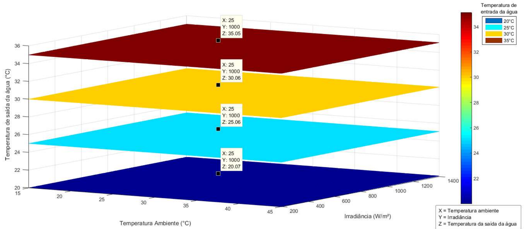
Figura 62. Temperatura de saída da água em função da radiação solar e temperatura ambiente à uma temperatura de entrada de (a) 20°C e (b) 25°C
