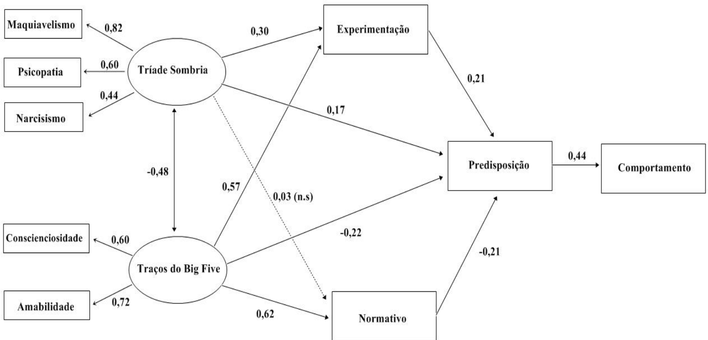
Figure 1. Modelo explicativo da infidelidade
