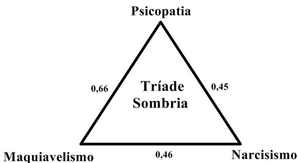
Figura 2. Correlações entre os membros da Tríade Sombria
