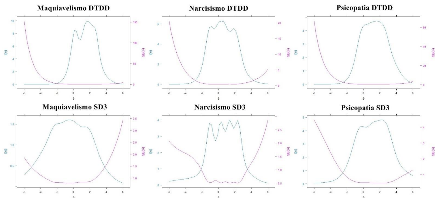
Figura 1. Informação psicométrica das subescalas
