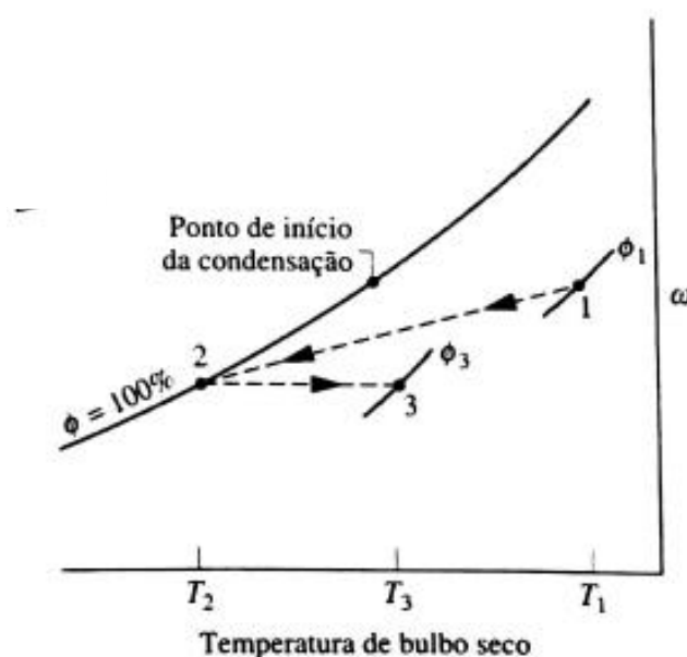
Figura 1.3 Esboço do processo de desumidificação
