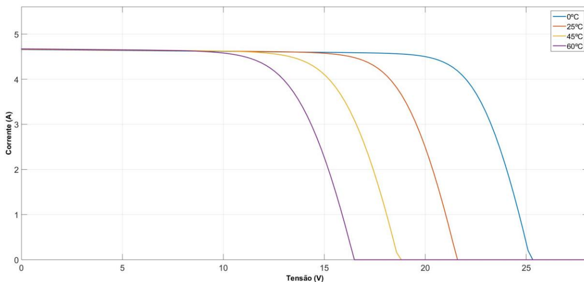
Figura 73. Curvas características I \times V da célula fotovoltaica IS-70/12 obtidas nas condições de G=1000 \text{ W/m}^2 e temperatura variando, T=0^\circ \text{C} , T=25^\circ \text{C} , T=45^\circ \text{C} e T=60^\circ \text{C} . Fonte: Elaborada pelo autor.
