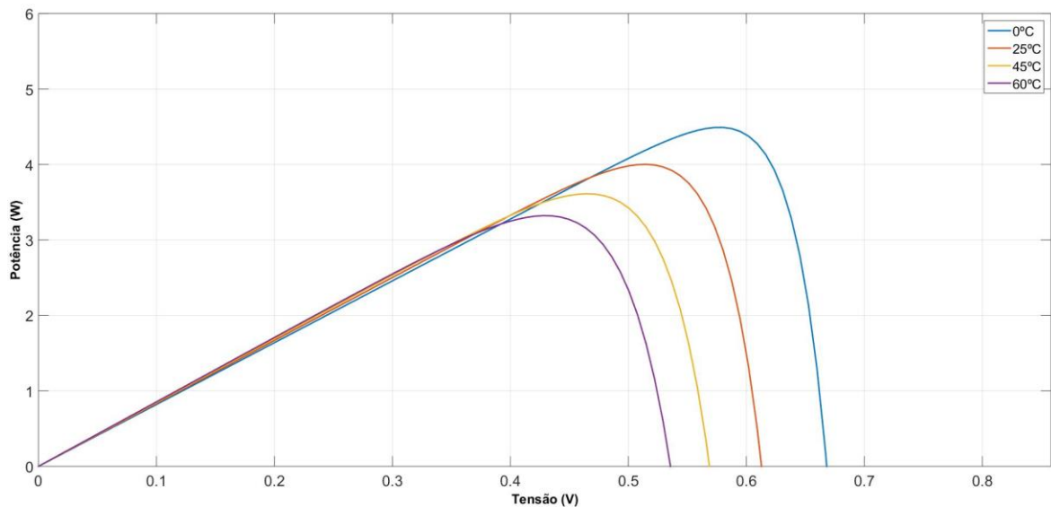
Figura 24. Curvas características P \times V da célula fotovoltaica Q6LPT3-G2 obtidas nas condições de G=1000 \text{ W/m}^2 e temperatura variando, T=0^\circ \text{C} , T=25^\circ \text{C} , T=45^\circ \text{C} e T=60^\circ \text{C} . Fonte: Elaborada pelo autor.
