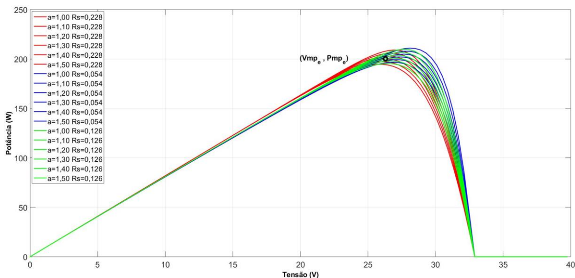
Figura 50. Curvas P \times V para diferentes fatores de idealidade e diferentes valores de resistências. Fonte: Elaborada pelo autor.
