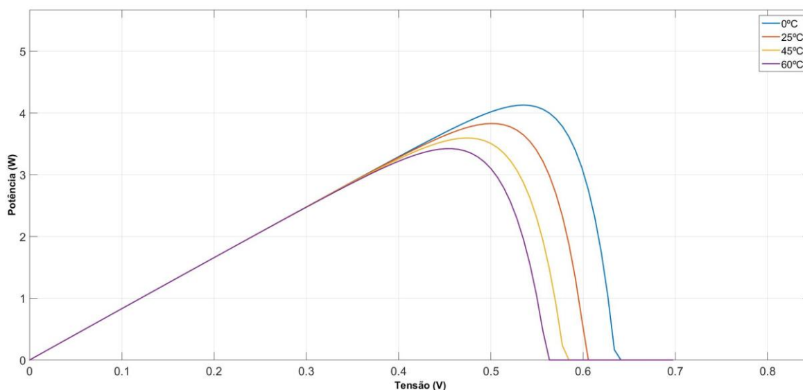
Figura 46. Curvas características P \times V da célula fotovoltaica Q6LM obtidas nas condições de G=1000\text{W/m}^2 e temperatura variando, T=0^\circ\text{C} , T=25^\circ\text{C} , T=45^\circ\text{C} e T=60^\circ\text{C} . Fonte: Elaborada pelo autor.
