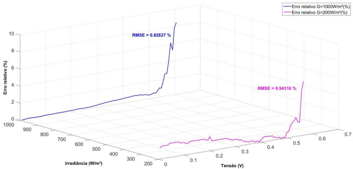
Figura 23. Curvas do erro relativo entre as curvas de potência, apresentada na folha de dados do fabricante e as curvas estimadas pelo modelo, nas condições STC e ( T=25\text{ }^{\circ}\text{C} , G=200\text{ W/m}^2 ) para a célula fotovoltaica Q6LPT3-G2. Fonte: Elaborada pelo autor.
