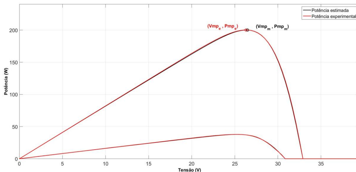
Figura 32. Curvas características P \times V , estimadas pela simulação e retiradas do datasheet, para o módulo fotovoltaico KC200GT nas condições STC e ( T=25^\circ\text{C} , G=200\text{ W/m}^2 ). Fonte: Elaborada pelo autor.
