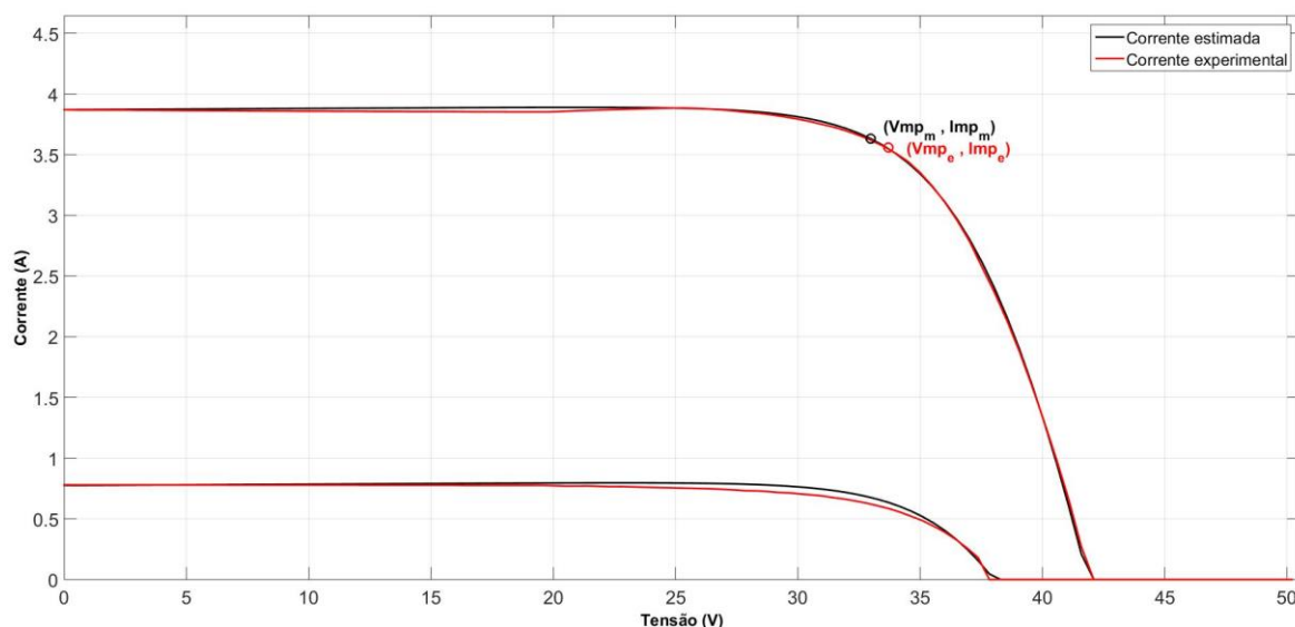
Figura 37. Curvas características I \times V , estimadas pela simulação e retiradas do datasheet, para o módulo fotovoltaico BP-MSZ 120 nas condições STC e ( T=25\text{ }^{\circ}\text{C} , G=200\text{ W/m}^2 ). Fonte: Elaborada pelo autor.
