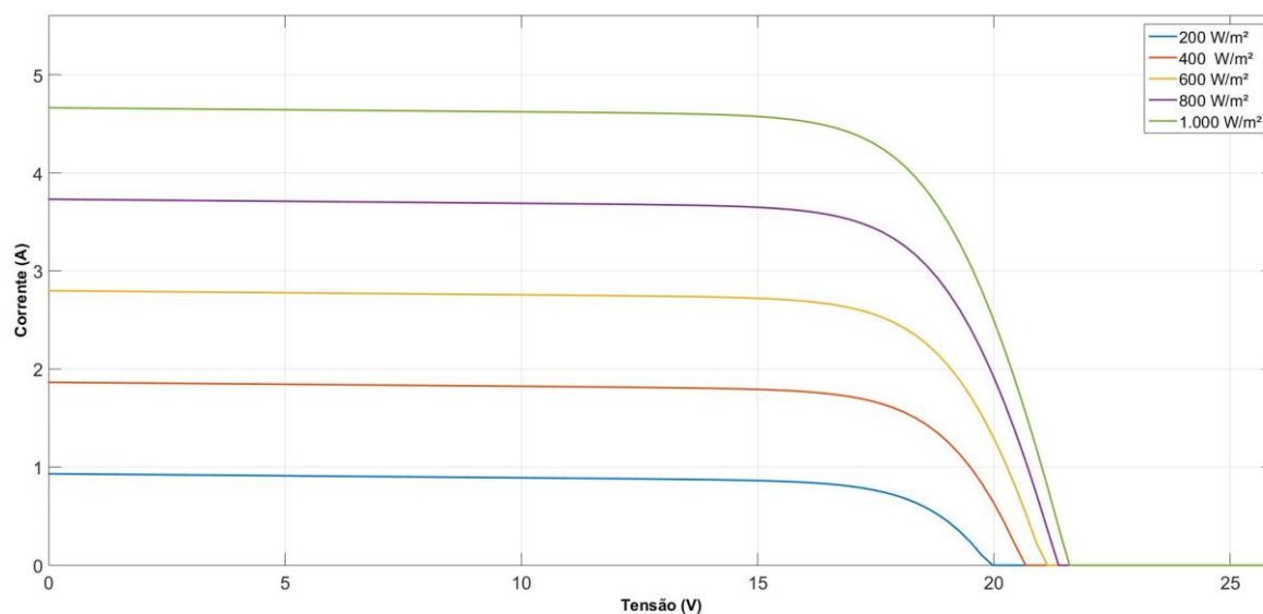
Figura 74. Curvas características I \times V do módulo fotovoltaico IS-70/12 obtidas nas condições de T=25\text{ }^{\circ}\text{C} , e irradiância variando, G=1000\text{ W/m}^2 , G=800\text{ W/m}^2 , G=600\text{ W/m}^2 , G=400\text{ W/m}^2 , G=200\text{ W/m}^2 . Fonte: Elaborada pelo autor.
