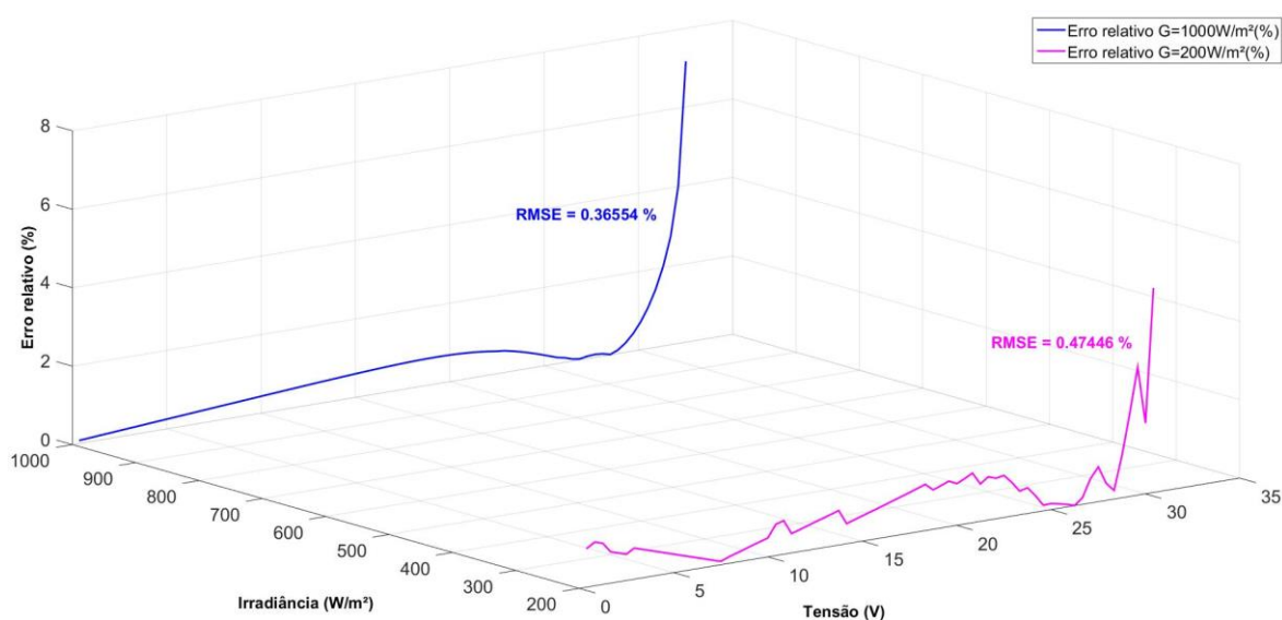
Figura 33. Curvas do erro relativo entre as curvas de potência, apresentada na folha de dados do fabricante e as curvas estimadas pelo modelo, nas condições STC e ( T=25^\circ\text{C} , G=200\text{ W/m}^2 ) para o módulo fotovoltaico KC200GT. Fonte: Elaborada pelo autor.
