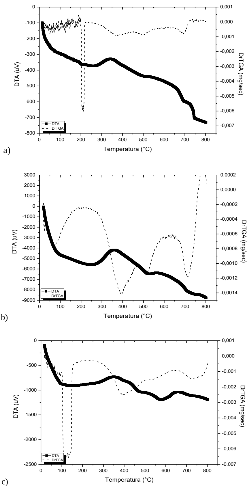
Figura 55: Gráficos de DTA-DrTGA versus Temperatura LaNiO 3 método Pechini , a) 05 °C.min -1 , b) 10 °C.min -1 e c) 15 °C.min -1 .
