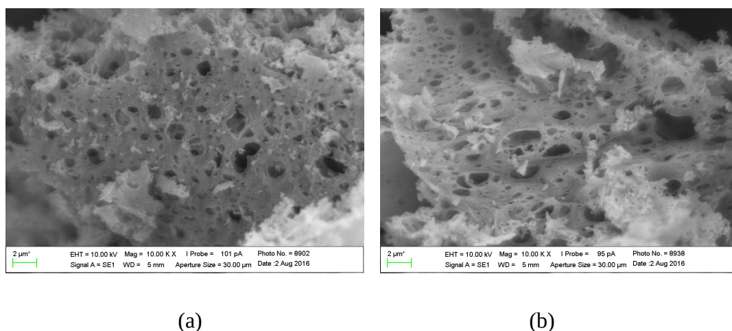
Figura 15: Micrografia dos compostos (a) \text{LaNiO}_3 e (b) \text{LaNi}_{0,8}\text{Co}_{0,2}\text{O}_3 pelo método da gelatina.
