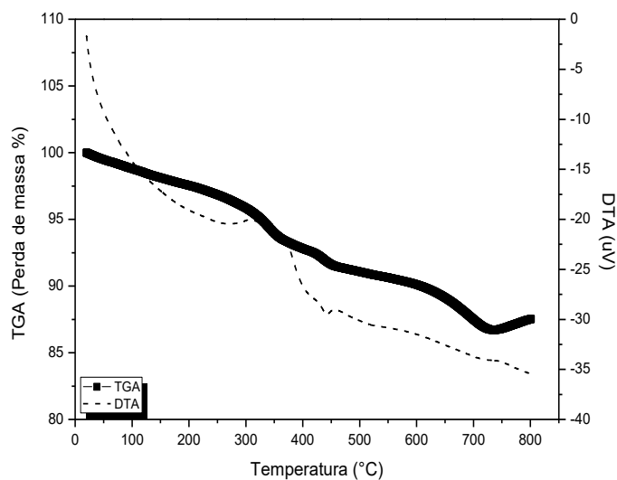
Figura 26: Gráficos de TGA-DTA versus Temperatura do \text{LaNi}_{0,8}\text{Co}_{0,2}\text{O}_3 , 10\text{ }^{\circ}\text{C}.\text{min}^{-1}
