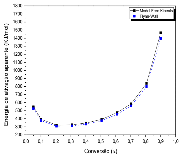
Figura 37: Energia de ativação aparente versus grau de conversão do \text{LaNiO}_3 .
