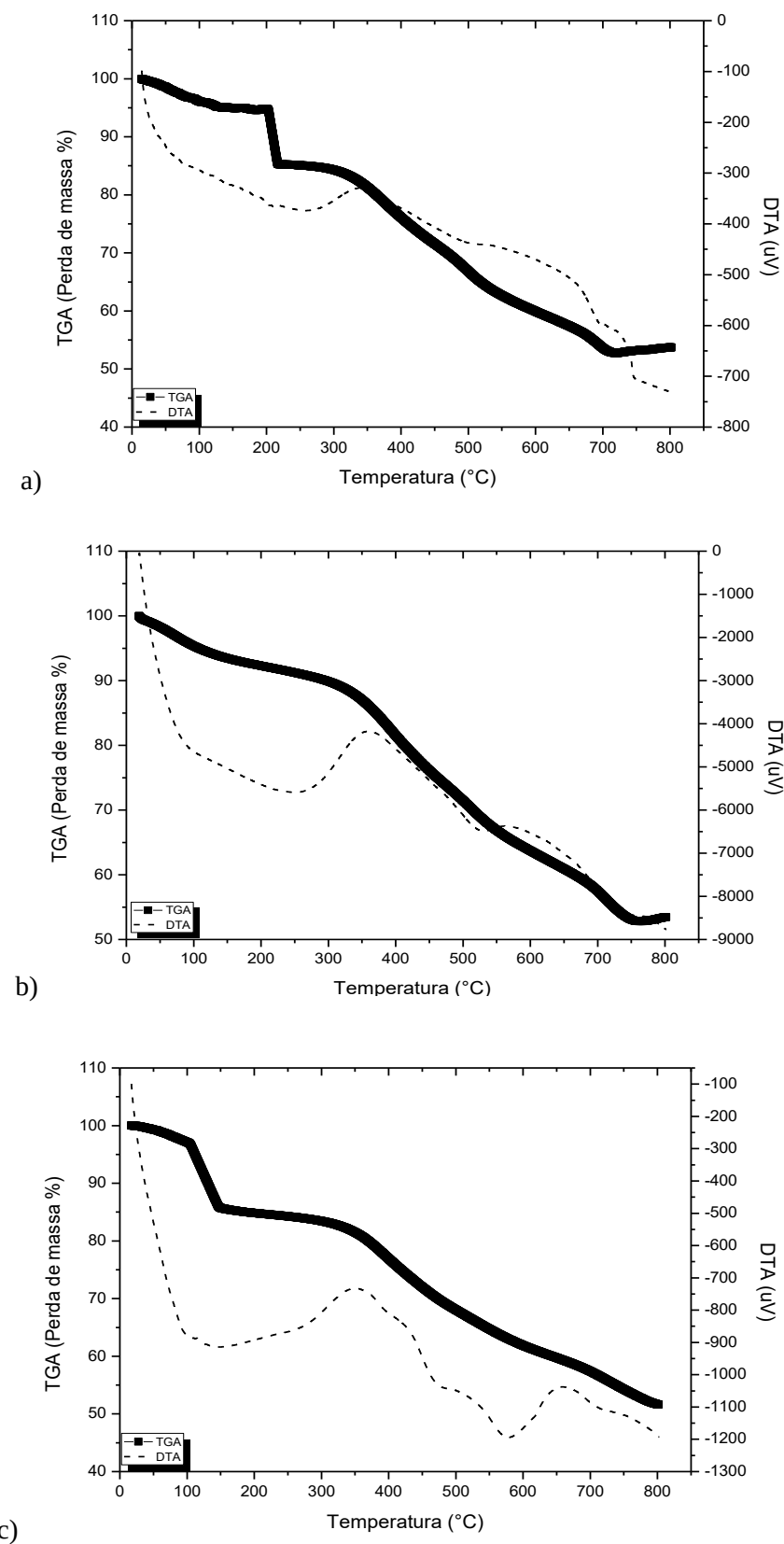
Figura 51: Gráficos de TGA-DTA versus Temperatura \text{LaNiO}_3 método Pechini, a) 05 °C.min -1 , b) 10 °C.min -1 e c) 15 °C.min -1 .
