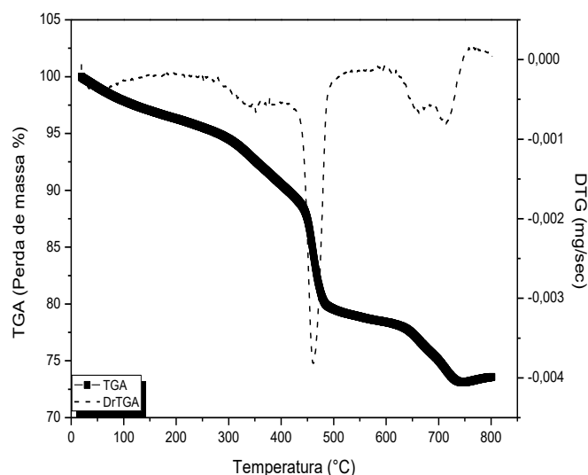
Figura 18: Gráficos da TGA-DTG versus Temperatura, 10\text{ }^{\circ}\text{C}.\text{min}^{-1} .
