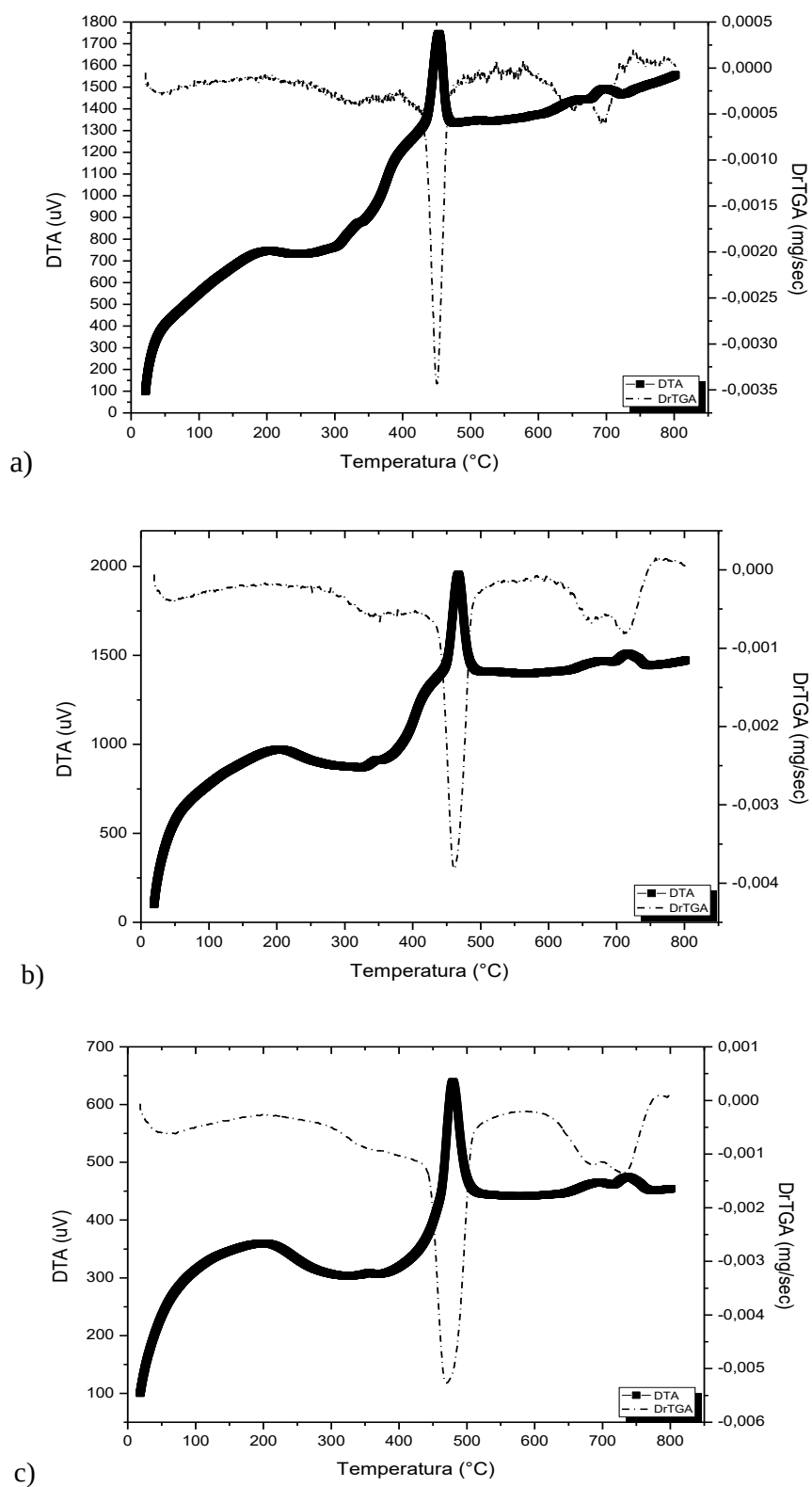
Figura 53: Gráficos de DTA-DrTGA versus Temperatura \text{LaNiO}_3 método da gelatina, a) 05\text{ }^\circ\text{C.min}^{-1} , b) 10\text{ }^\circ\text{C.min}^{-1} e c) 15\text{ }^\circ\text{C.min}^{-1} .
