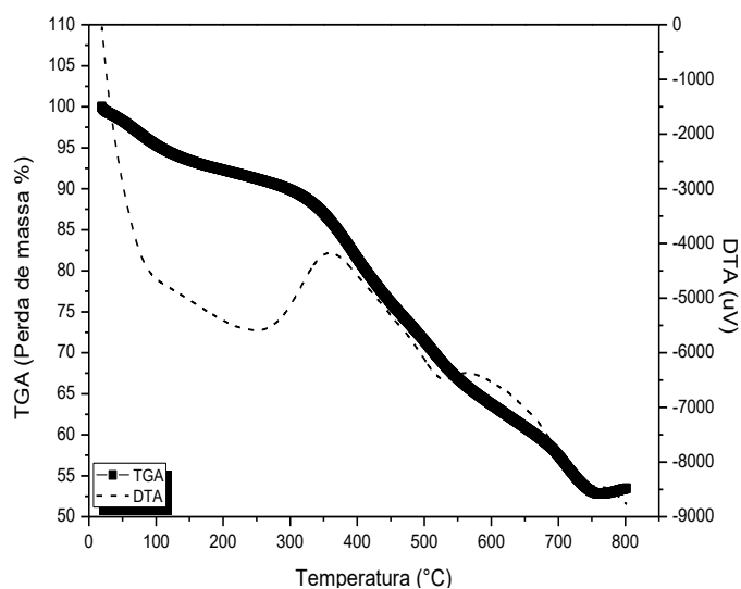
Figura 33: Gráficos de TGA-DTA versus Temperatura do \text{LaNiO}_3 , 10 ^{\circ}\text{C}.\text{min}^{-1} .
