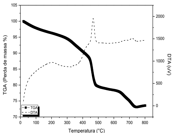
Figura 19: Gráficos de TGA-DTA versus Temperatura, 10 °C.min -1 .
