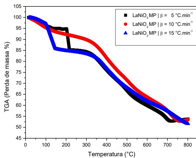
Figura 31: Curvas termogravimétricas do \text{LaNiO}_3 com três diferentes razões de aquecimento ( \beta ).
