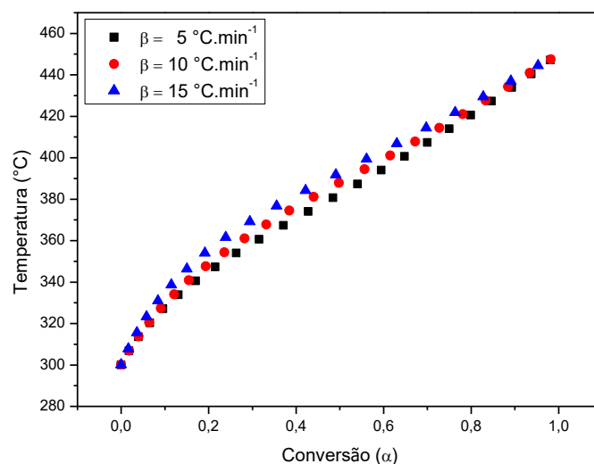
Figura 34: Gráfico conversão versus temperatura do \text{LaNiO}_3 .
