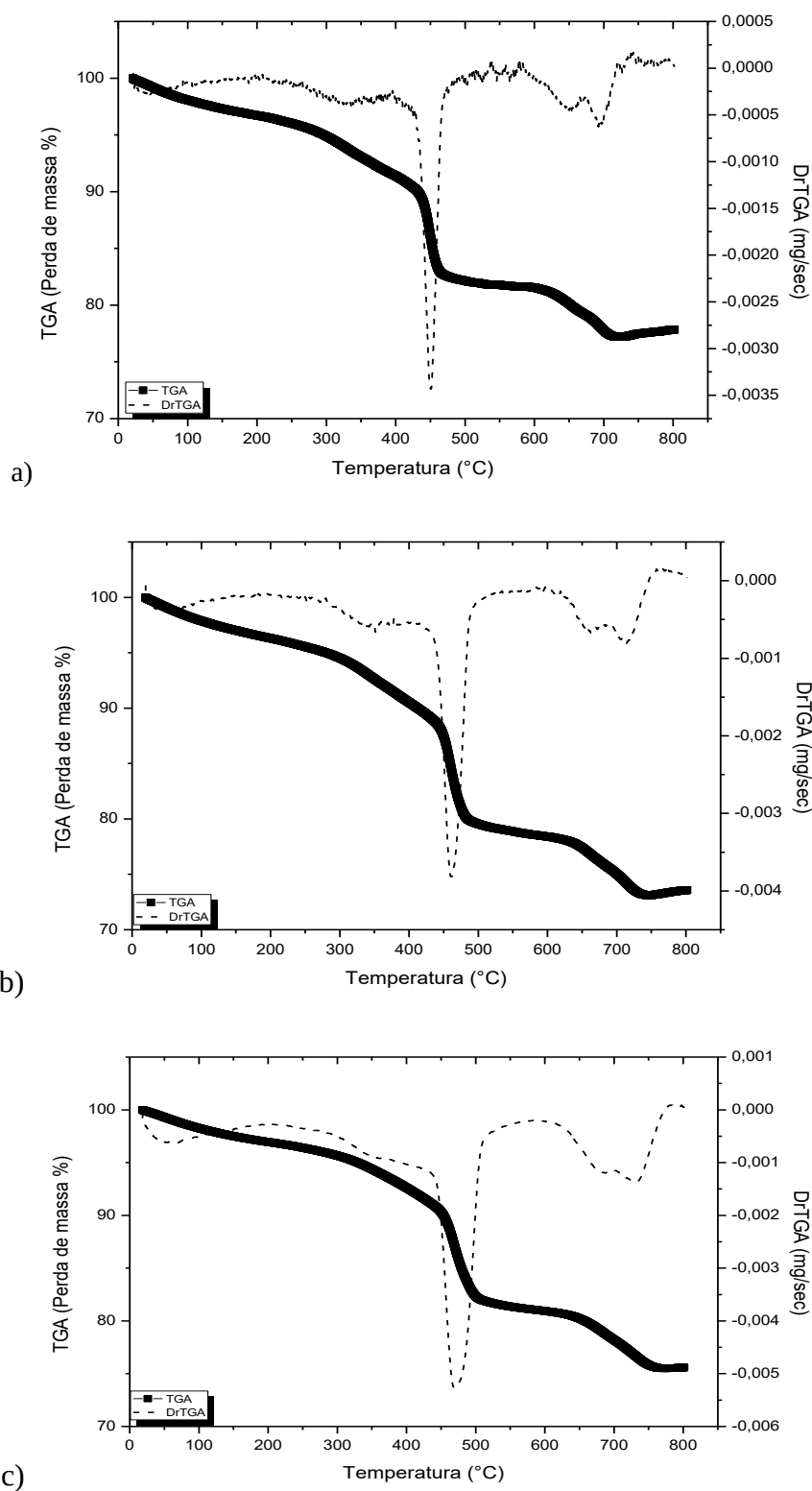
Figura 45: Gráficos da TGA-DrTGA versus Temperatura do \text{LaNiO}_3 Método da gelatina, a) 05 °C.min -1 , b) 10 °C.min -1 e c) 15 °C.min -1 .
