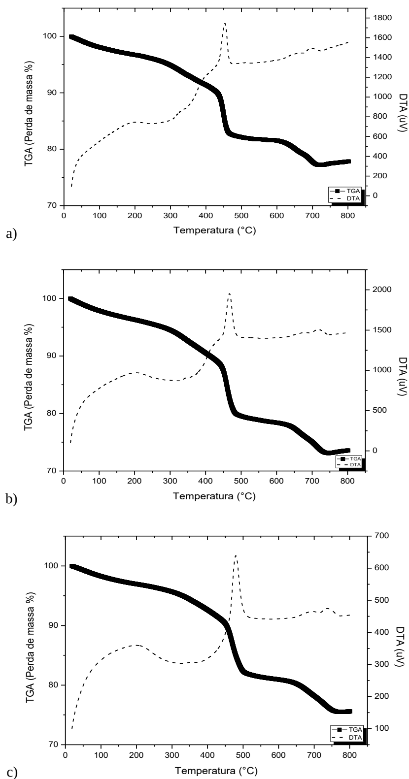
Figura 49: Gráficos de TGA-DTA versus Temperatura \text{LaNiO}_3 método da gelatina, a) 05\text{ }^\circ\text{C}\cdot\text{min}^{-1} , b) 10\text{ }^\circ\text{C}\cdot\text{min}^{-1} e c) 15\text{ }^\circ\text{C}\cdot\text{min}^{-1} .
