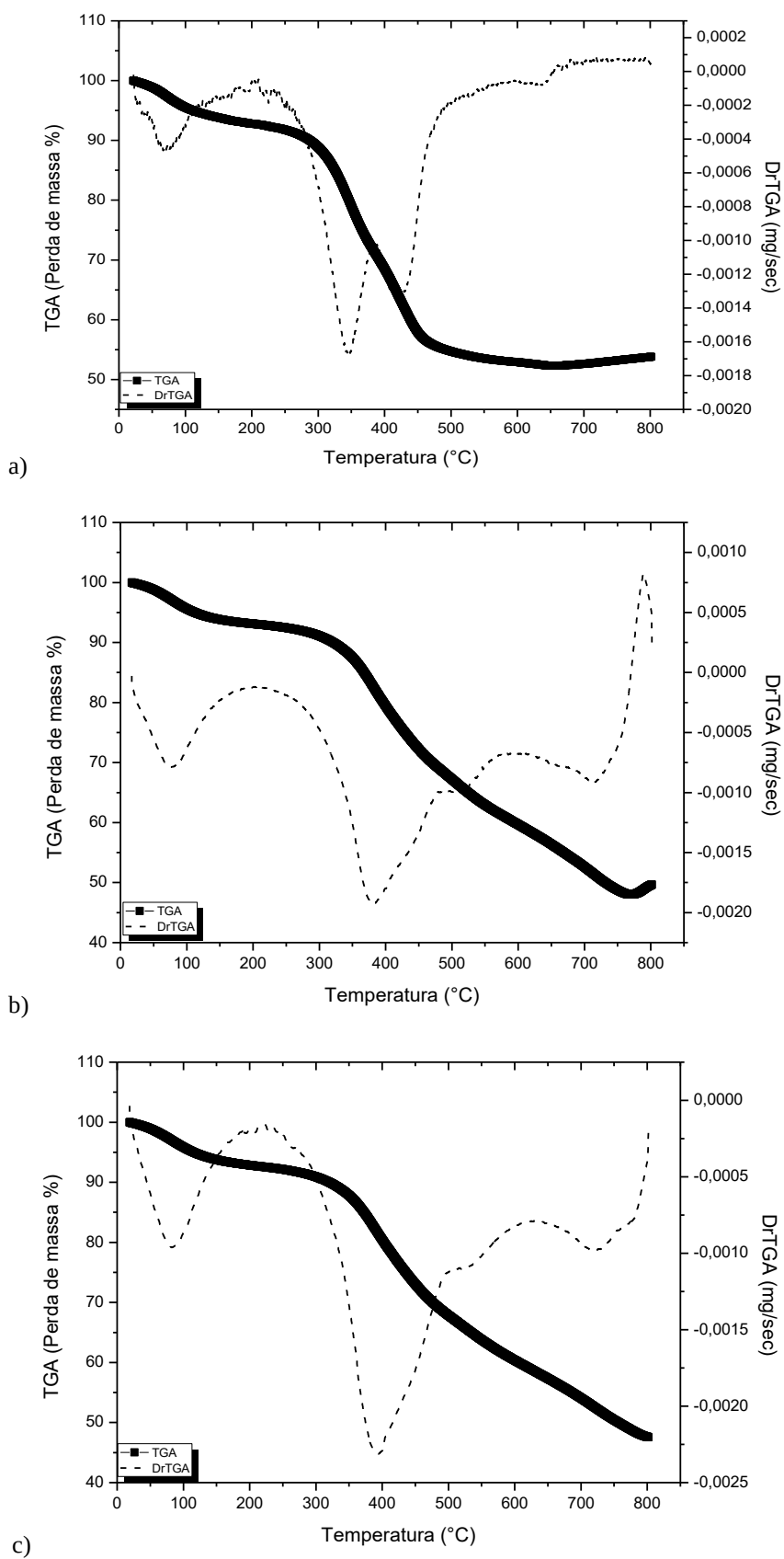
Figura 48: Gráficos da TGA-DrTGA versus Temperatura do \text{LaNi}_{0.8}\text{Co}_{0.2}\text{O}_3 método Pechini, a) 05 °C.min -1 , b) 10 °C.min -1 e c) 15 °C.min -1 .
