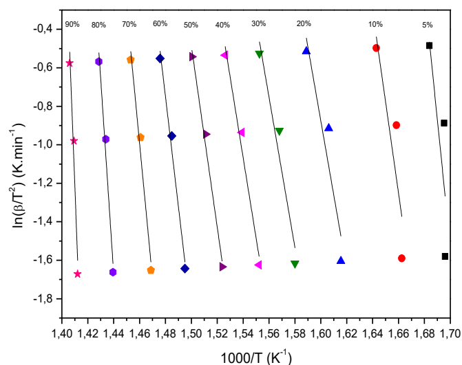
Figura 36: Logaritmo natural da razão de aquecimento dividido pela temperatura ao quadrado versus 1000/T do \text{LaNiO}_3 , Model Free Kinetics.
