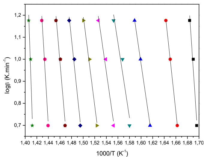
Figura 35: Logaritmo da razão de aquecimento versus 1000/T do \text{LaNiO}_3 , Flynn-Wall.
