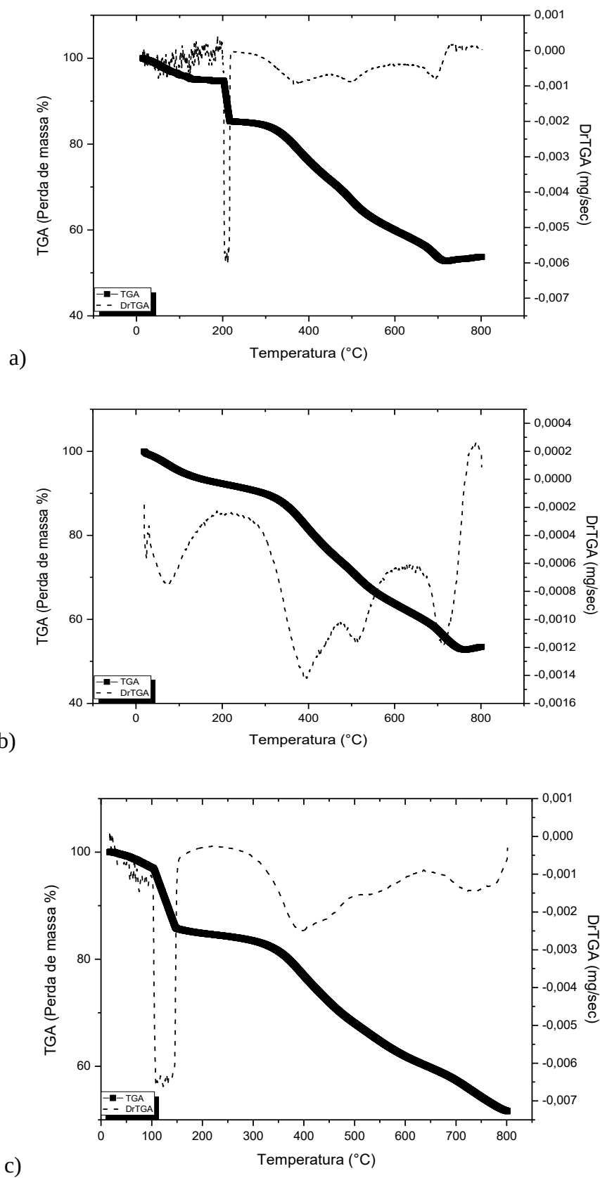
Figura 47: Gráficos da TGA-DrTGA versus Temperatura \text{LaNiO}_3 Método Pechini, a) 05 °C.min -1 , b) 10 °C.min -1 e c) 15 °C.min -1 .
