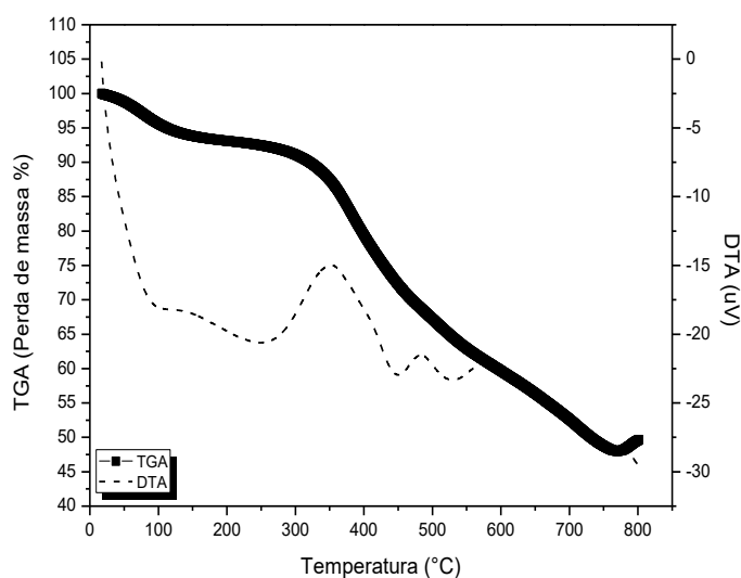
Figura 40: Gráficos de TGA-DTA versus Temperatura do \text{LaNi}_{0,8}\text{Co}_{0,2}\text{O}_3 , 10 ^{\circ}\text{C}.\text{min}^{-1} .
