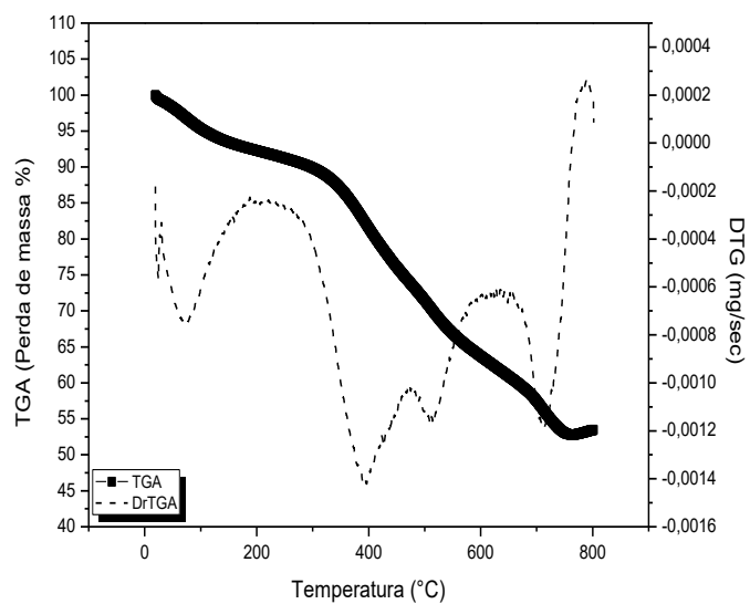
Figura 32: Gráficos da TGA-DTG versus Temperatura do \text{LaNiO}_3 , 10\text{ }^{\circ}\text{C.min}^{-1} .
