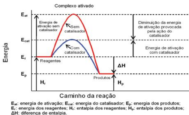
Figura 1: Reação não catalisada versus reação catalisada.
