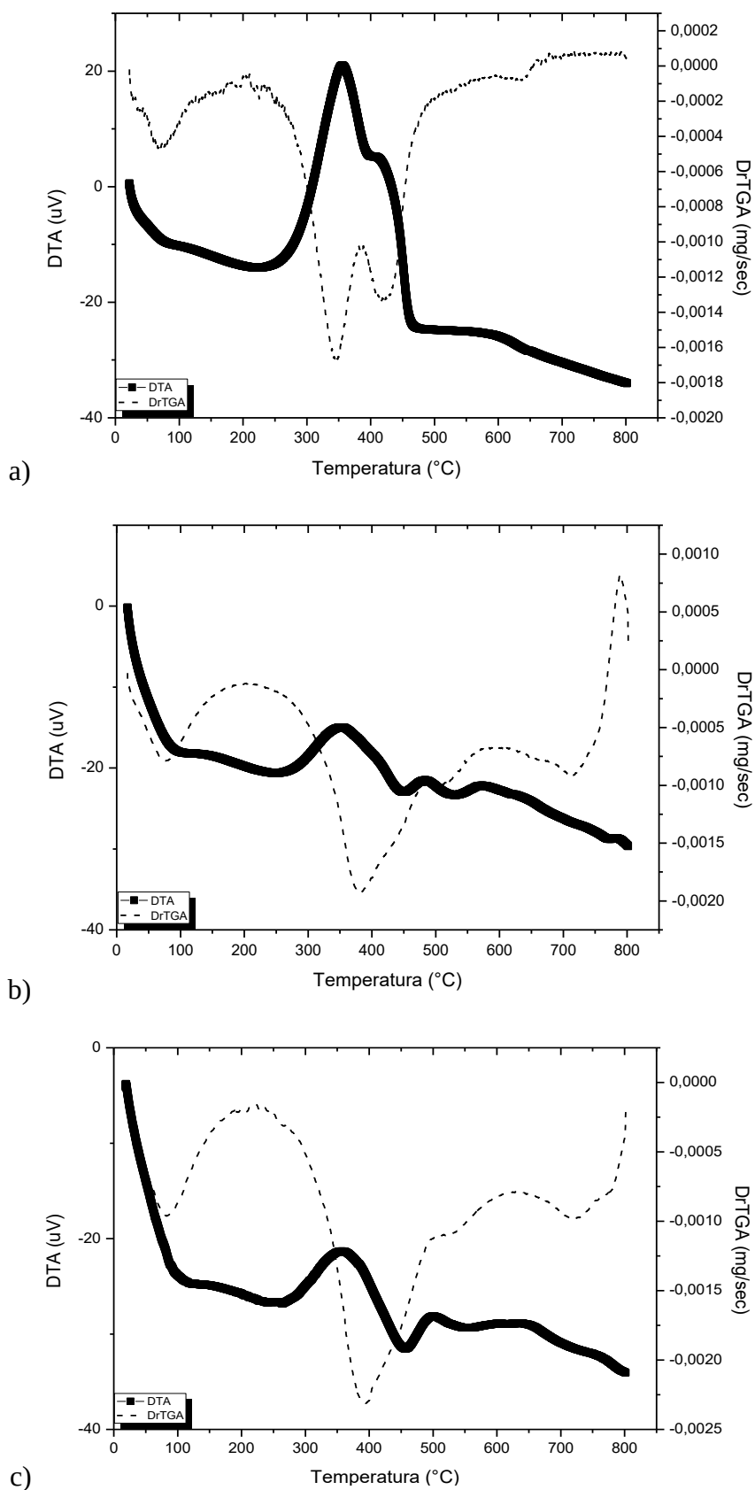
Figura 56: Gráficos de DTA-DrTGA versus Temperatura \text{LaNi}_{0.8}\text{Co}_{0.2}\text{O}_3 método Pechini, a) 05 °C.min -1 , b) 10 °C.min -1 e c) 15 °C.min -1 .
