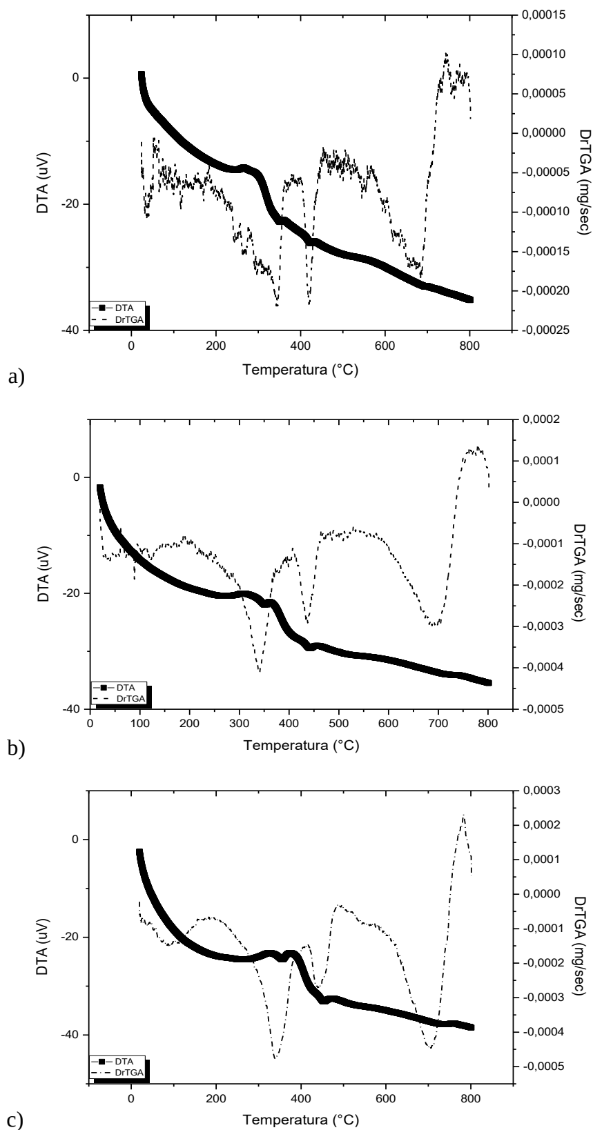
Figura 54: Gráficos de DTA-DrTGA versus Temperatura \text{LaNi}_{0.8}\text{Co}_{0.2}\text{O}_3 método da gelatina, a) 05 °C.min -1 , b) 10 °C.min -1 e c) 15 °C.min -1 .
