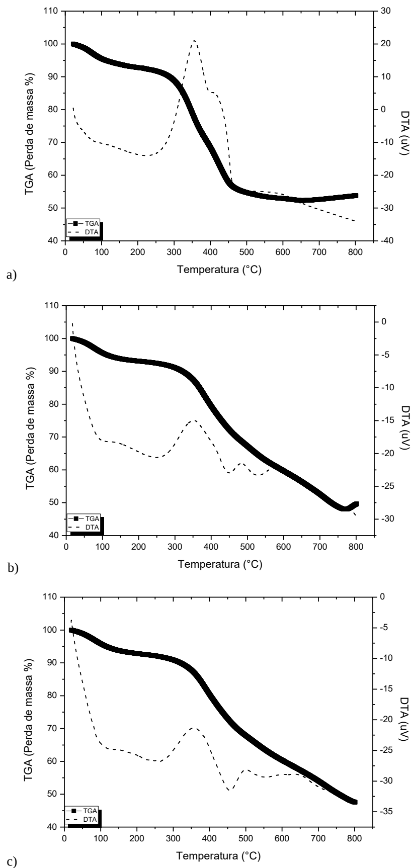
Figura 52: Gráficos de TGA-DTA versus Temperatura \text{LaNi}_{0.8}\text{Co}_{0.2}\text{O}_3 método Pechini, a) 05 °C.min -1 , b) 10 °C.min -1 e c) 15 °C.min -1 .
