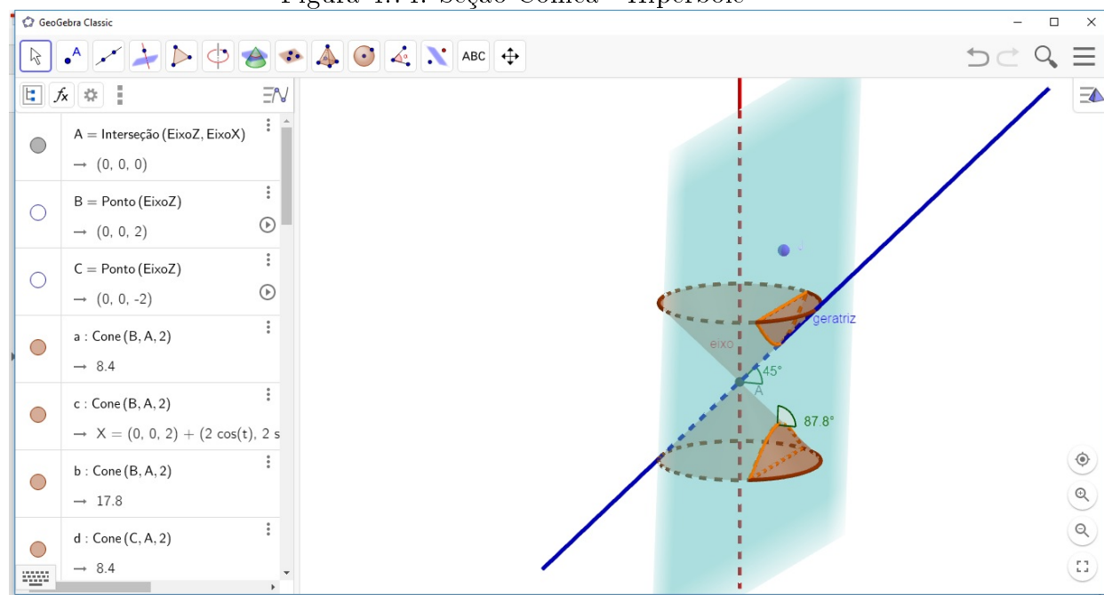
Figura 4.74: Seção Cônica - Hipérbole
