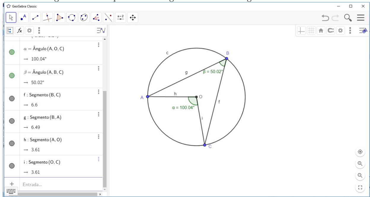
Figura 1.2: Relação entre o ângulo inscrito e o ângulo central
