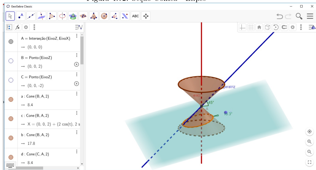
Figura 4.72: Seção Cônica - Elipse
