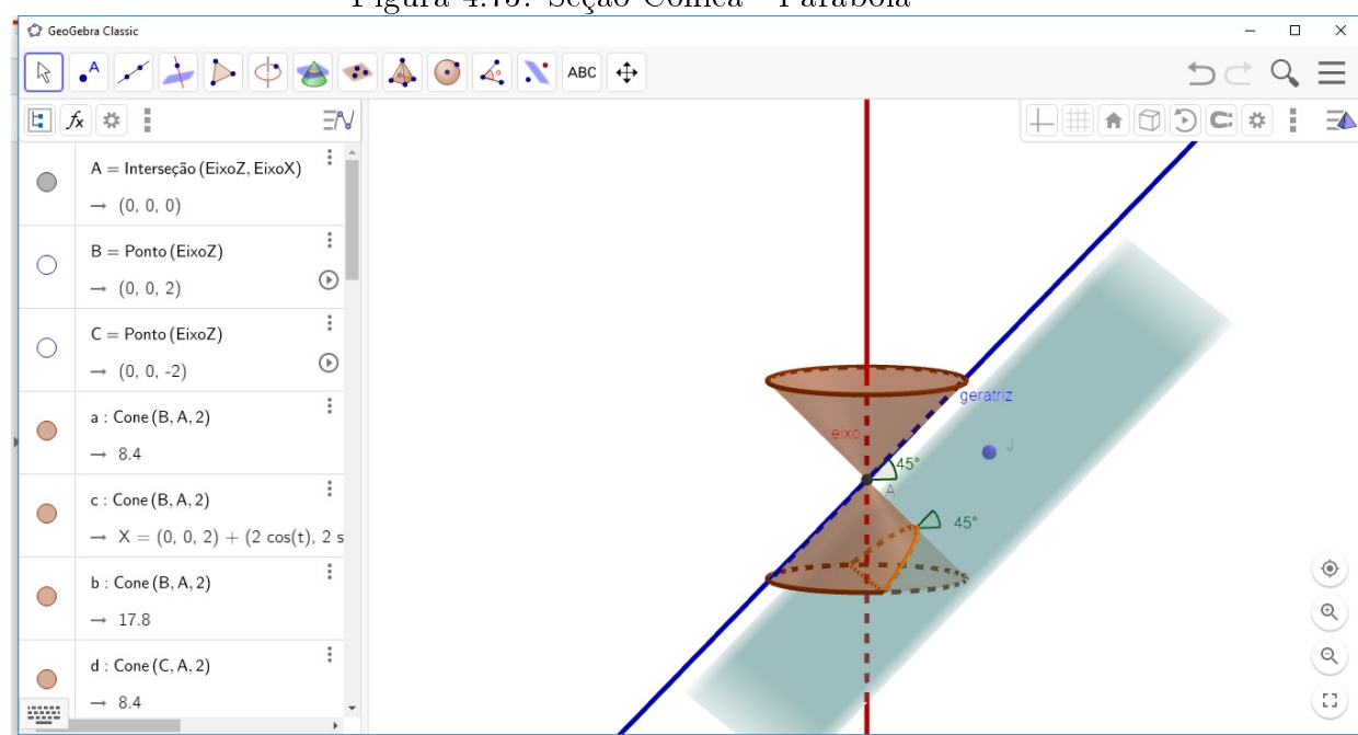
Figura 4.73: Seção Cônica - Parábola
