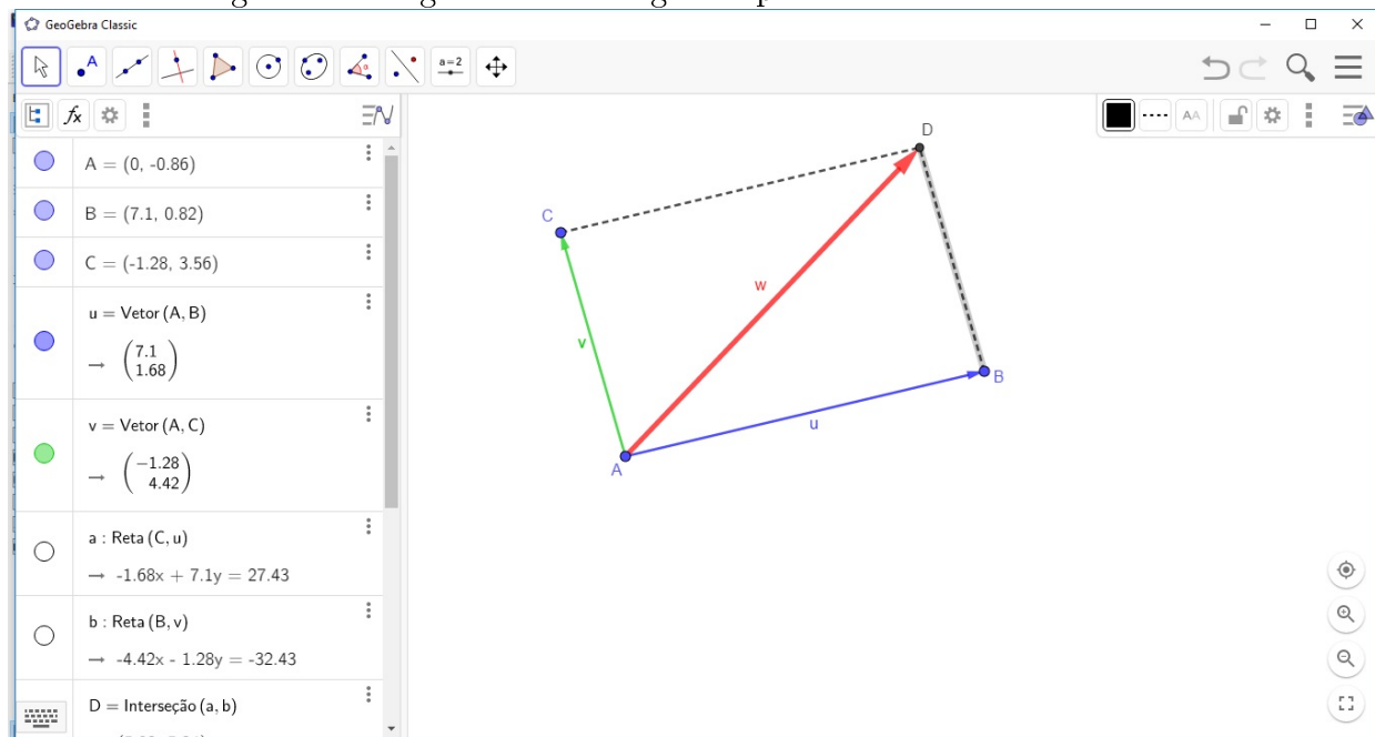
Figura 1.4: Regra do Paralelogramo para soma de vetores
