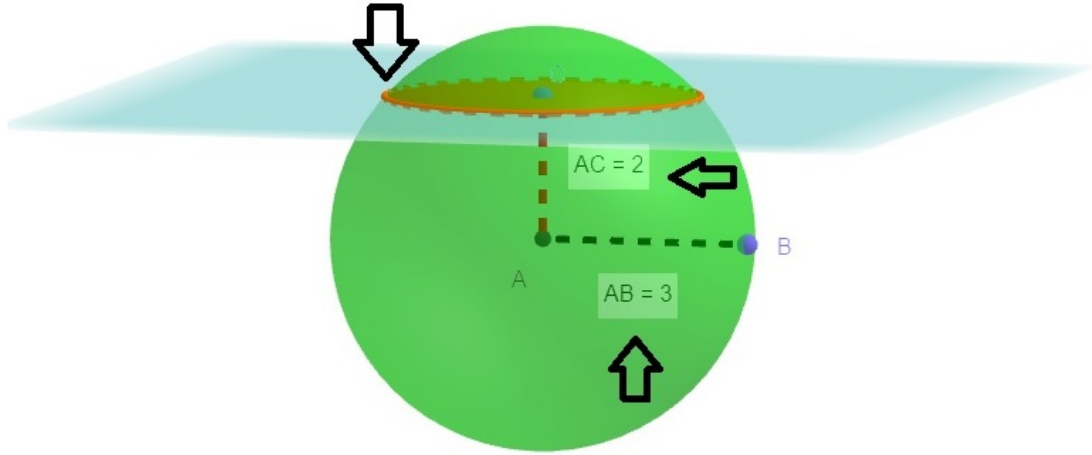
Figura 3.10: Interseção da esfera com o plano igual a um círculo
