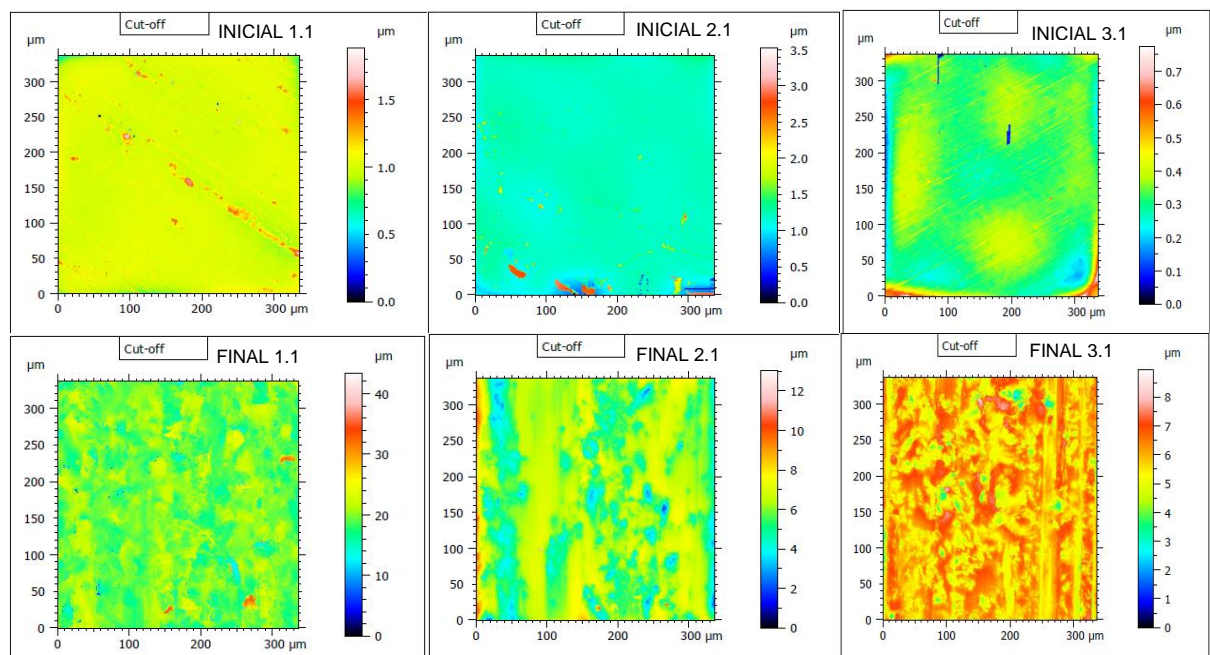
Figura 9: Imagens representativas da rugosidade de superfície das amostras obtidas nos relatórios de perfilometria
