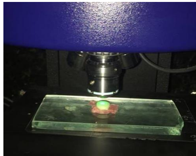
Figura 6: Análise da rugosidade inicial em perfilômetro Talysurf CCI MP
