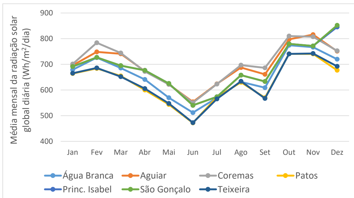
Figura 4.8 – Média mensal da radiação solar global diária (em Wh/m 2 /dia) para as localidades escolhidas da Mesorregião do Sertão Paraibano no horário de pico, entre 10h e 16h, fornecida pelo programa HelioClim.
