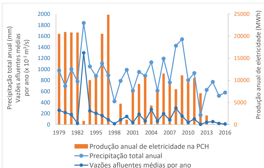
Figura 4.5 – Valores anuais para a precipitação total (em mm), vazões afluentes médias ( \times 10^{-1} \text{ m}^3/\text{s} ) e geração de eletricidade pela pequena central hidroelétrica (em MWh) em Coremas com dados de 1979 a 2016.
