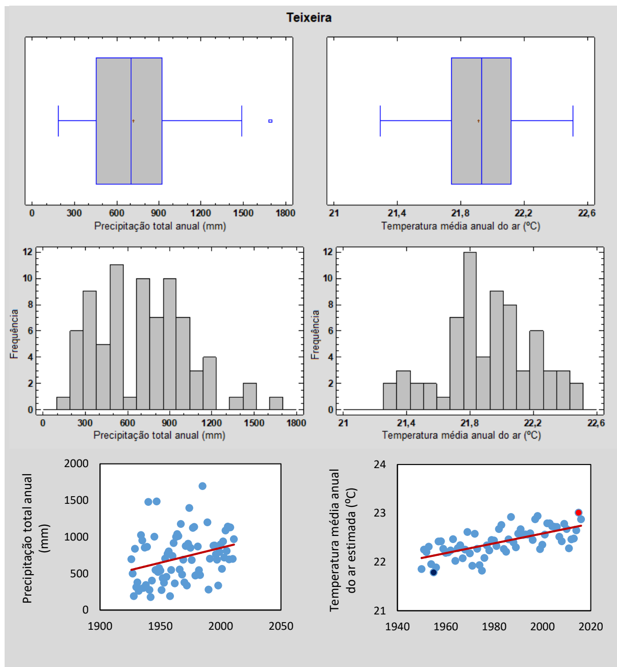
Figura 7 – Gráficos box-plot, de dispersão e histogramas para precipitação total anual (mm), com dados de 1926 a 2011, e temperatura média do ar estimada (°C), com dados de 1950 a 2016, para o município de Teixeira.
