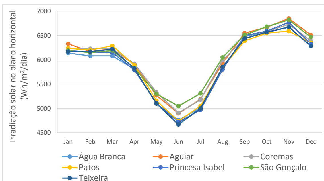
Figura 4.9 – Irradiação solar no plano horizontal (em Wh/m 2 /dia) para as localidades escolhidas da Mesorregião do Sertão Paraibano fornecida pelo programa SunData.
