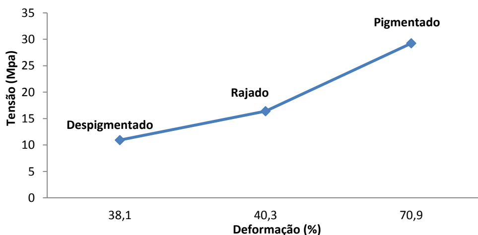
Figura 9. Médias do Módulo de Elasticidade para cascos brancos, rajados e pretos de ovinos Morada Nova.
