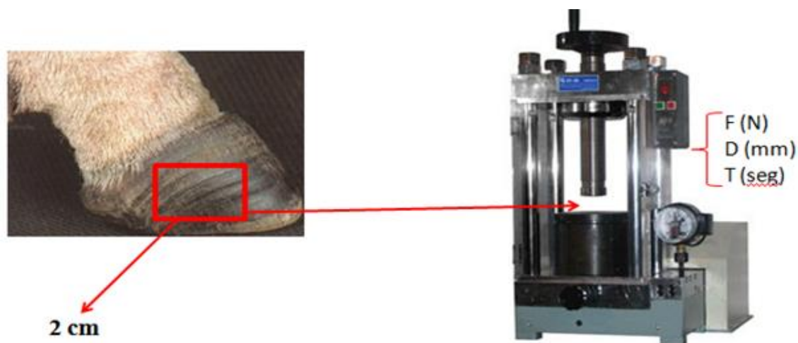
Figura 3. Metodologia aplicada nos testes de compressão dos cascos.
