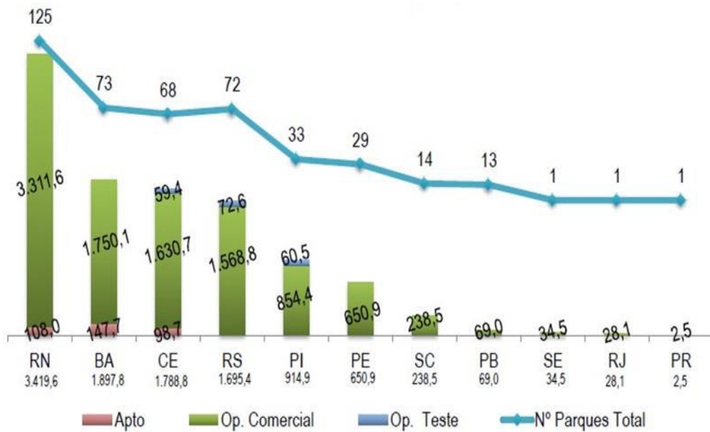
Figura 2- Potência instalada nos estados brasileiros, 2016 (MW)
