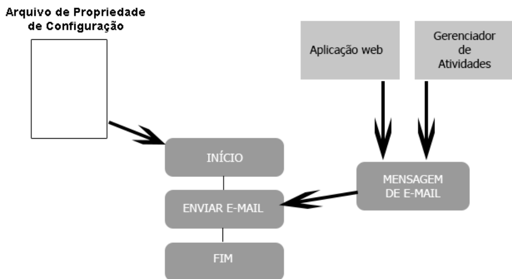
Figura 8 - Design de Alto Nível do Cliente de E-mail
