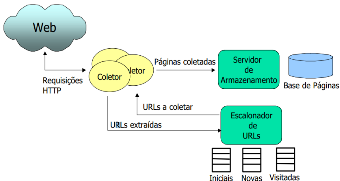
Figura 2 - Arquitetura Típica do Web Crawler
