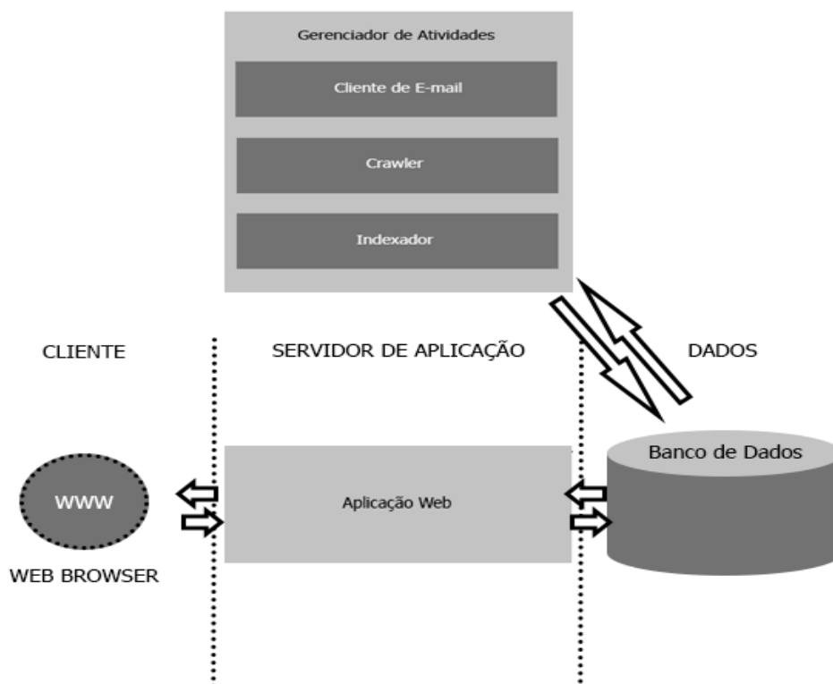
Figura 5 - Arquitetura Completa do Sistema
