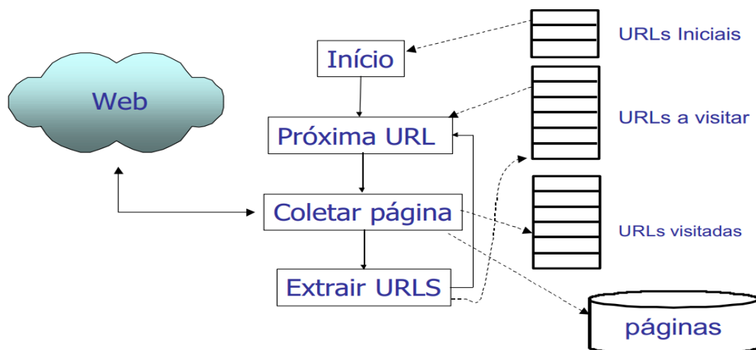
Figura 1 – Representação de um Web Crawler
