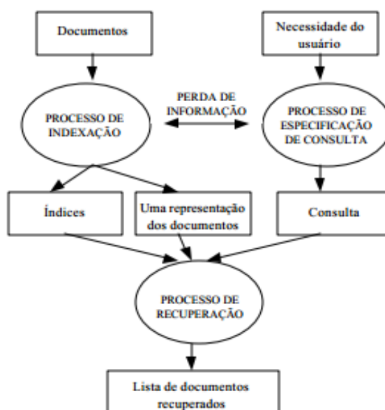
Figura 3 - Estrutura de um Sistema de Recuperação da Informação
