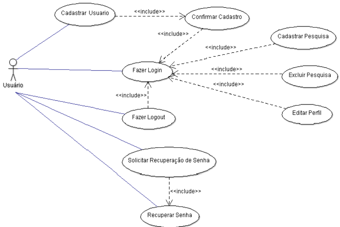
Figura 4 - Diagrama de Caso de Uso da Aplicação Web
