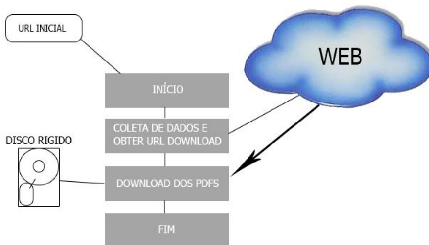
Figura 6 - Design de Alto Nível do Crawler
