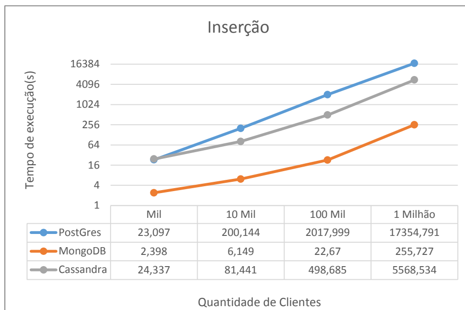
Figura 11 - Gráfico Insert
