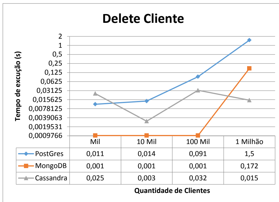
Figura 16 - Gráfico Delete
