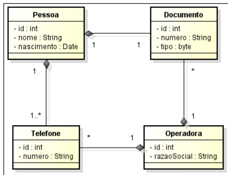
Figura 7- Diagrama classes
