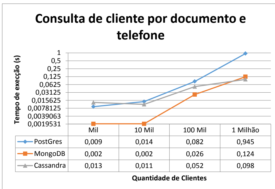
Figura 12- Gráfico Select
