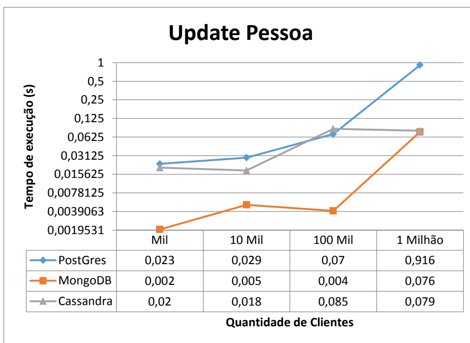
Figura 14 - Gráfico Update
