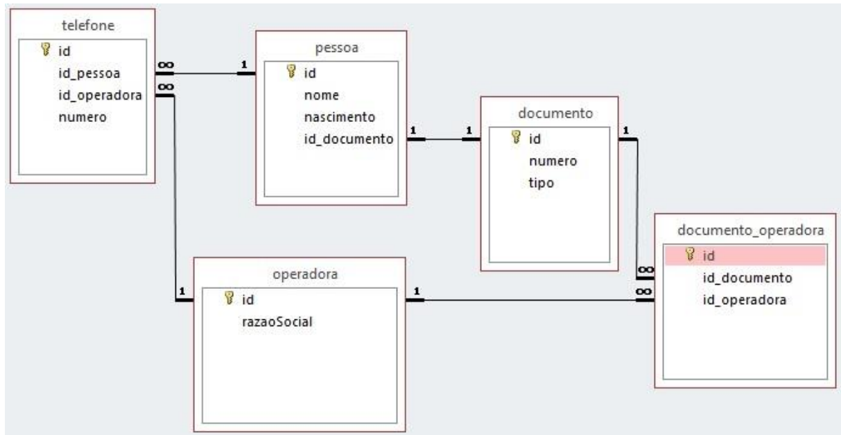
Figura 9 - Diagrama Lógico
