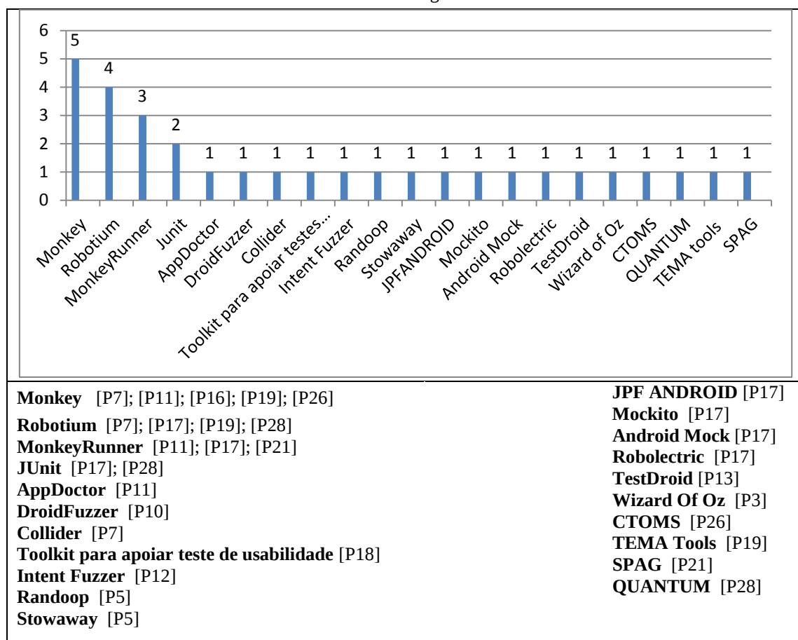
Gráfico 4: Ferramentas citadas nos artigos incluídos e relacionadas diretamente a eles..
