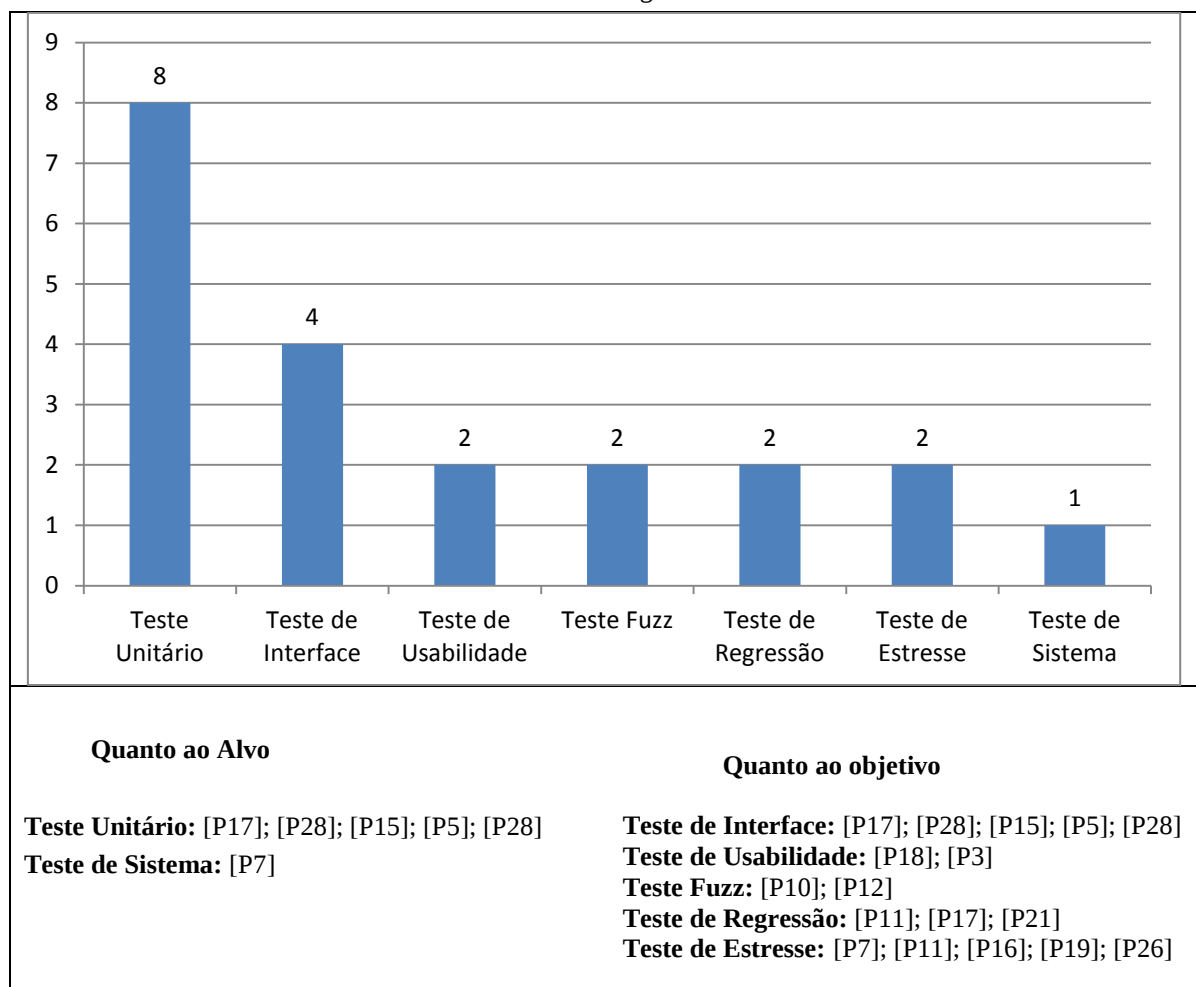
Gráfico 5: Quantidade dos tipos de teste cobertos pelas ferramentas de acordo com seu alvo ou objetivo, e os artigos.
