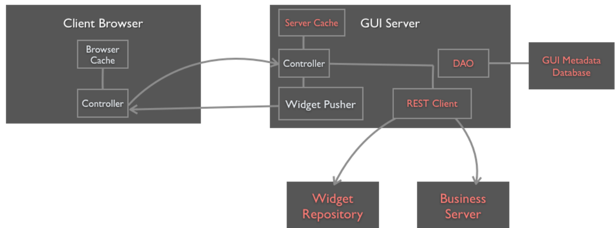
Figura 12 - Arquitetura da implementação web do LOM
