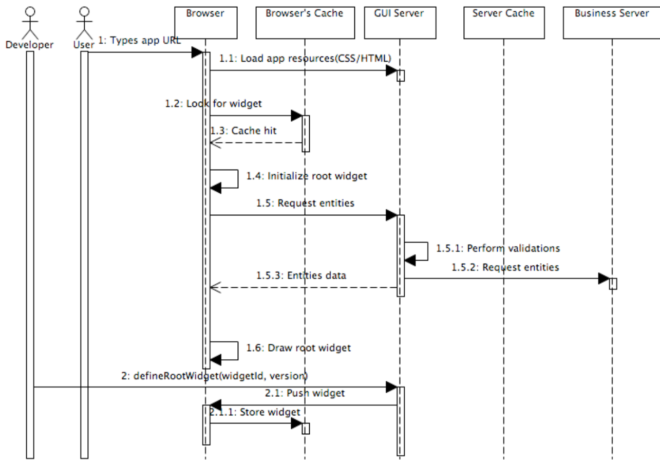
Figura 19 - Diagrama de sequência do cenário 6, onde o widget é atualizado com o usuário online
