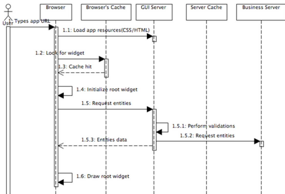
Figura 18 - Diagrama de sequência do cenário 5, usuário reabrindo a aplicação
