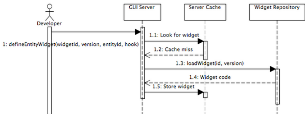
Figura 14 - Cenário 2, definindo entity widgets utilizando widgets que não estão no GUI Server
