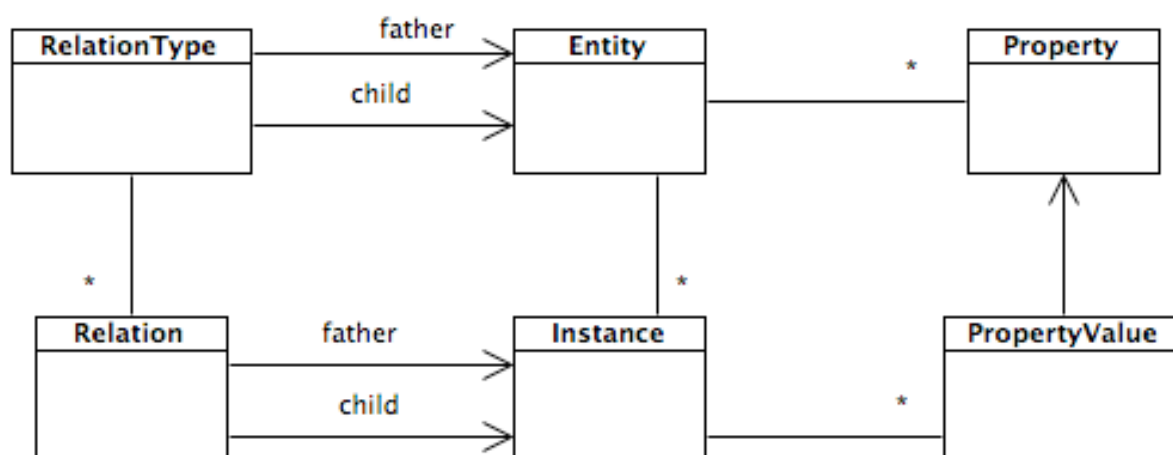
Figura 9 - Variação do Type Square utilizada pelo LOM
