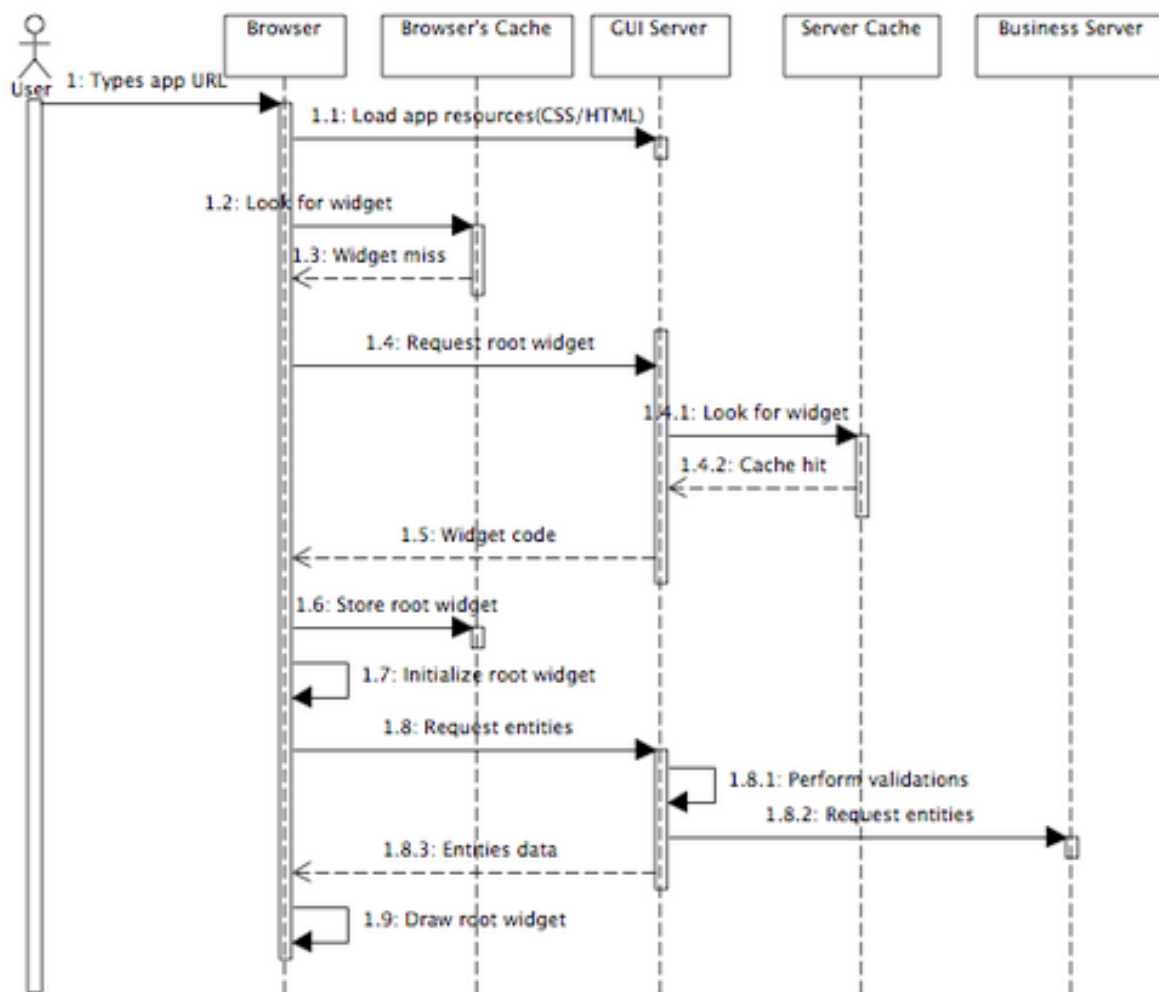
Figura 17 - Diagrama de sequência do cenário 4, outro usuário abrindo a aplicação
