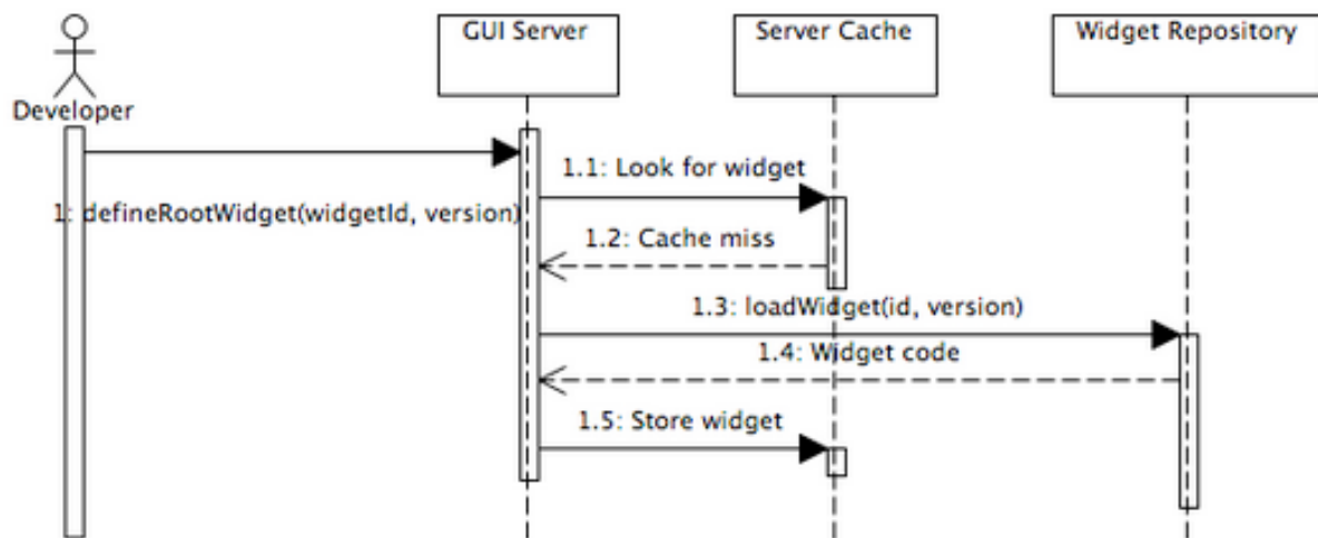
Figura 13 - Cenário 1, definindo Root Widget utilizando widgets que não está no GUI Server
