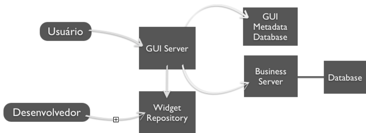
Figura 8 - LOM: Arquitetura geral
