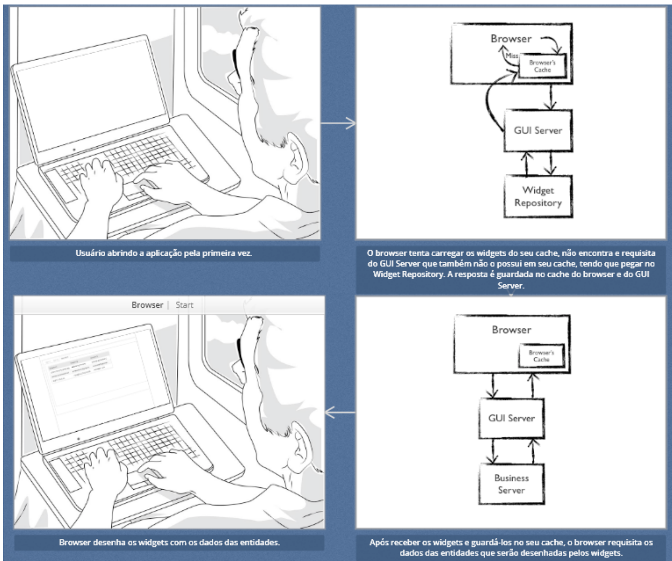
Figura 15 - Cenário 3, usuário abrindo a aplicação pela primeira vez
