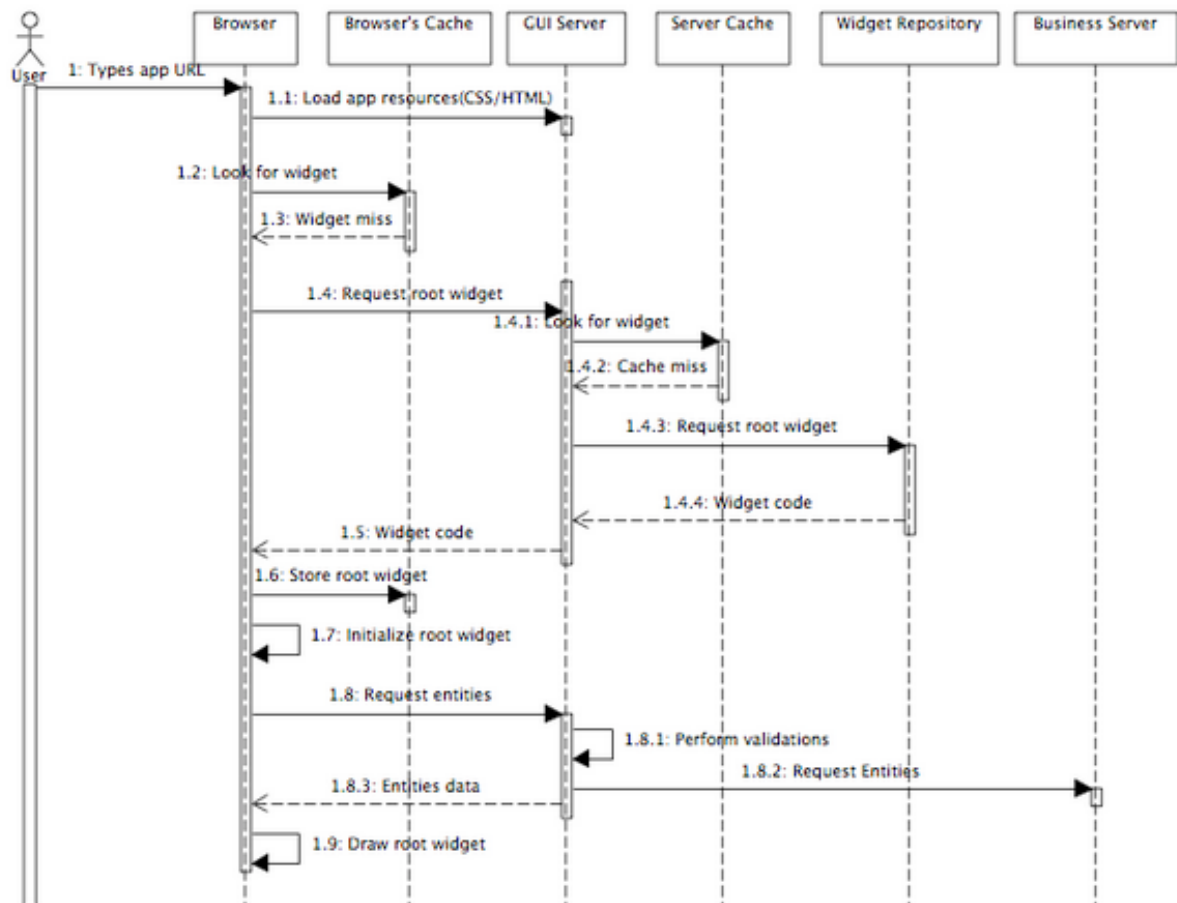
Figura 16 - Diagrama de sequência do Cenário 3, usuário abrindo a aplicação pela primeira vez
