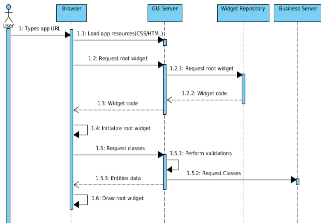
Figura 13 - Diagrama de Sequência User
