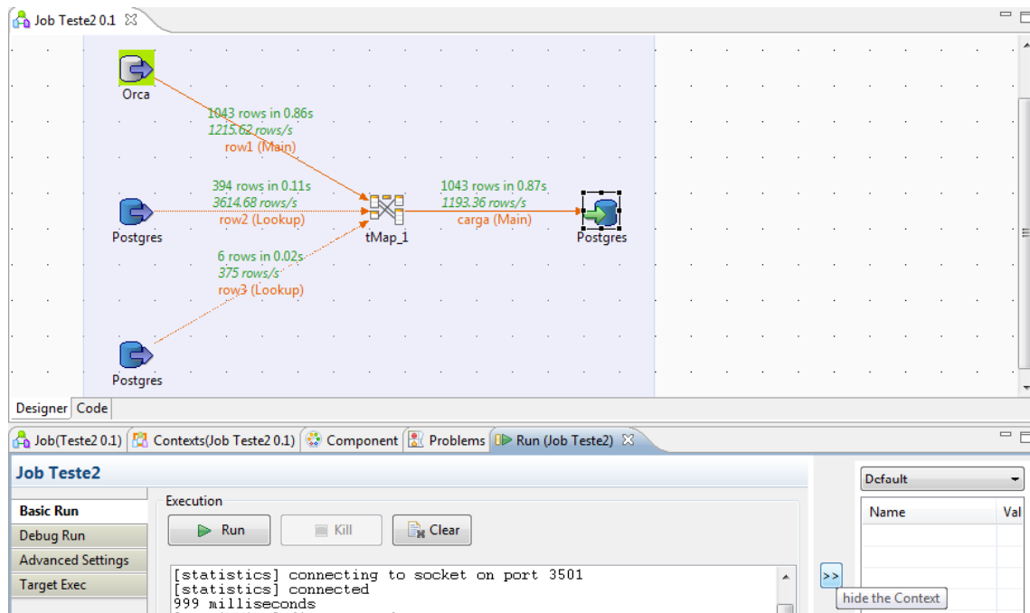
Figura 45 - Job da tabela Produto no Talend
