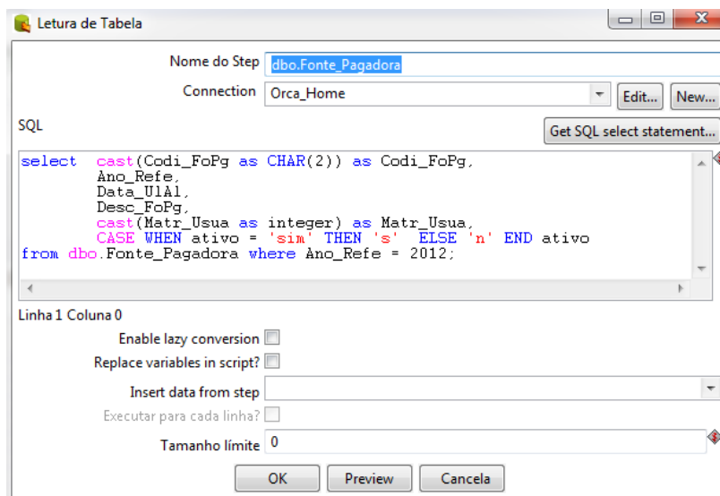
Figura 21 - Step para leitura/seleção dos dados no Kettle conforme a SML2
