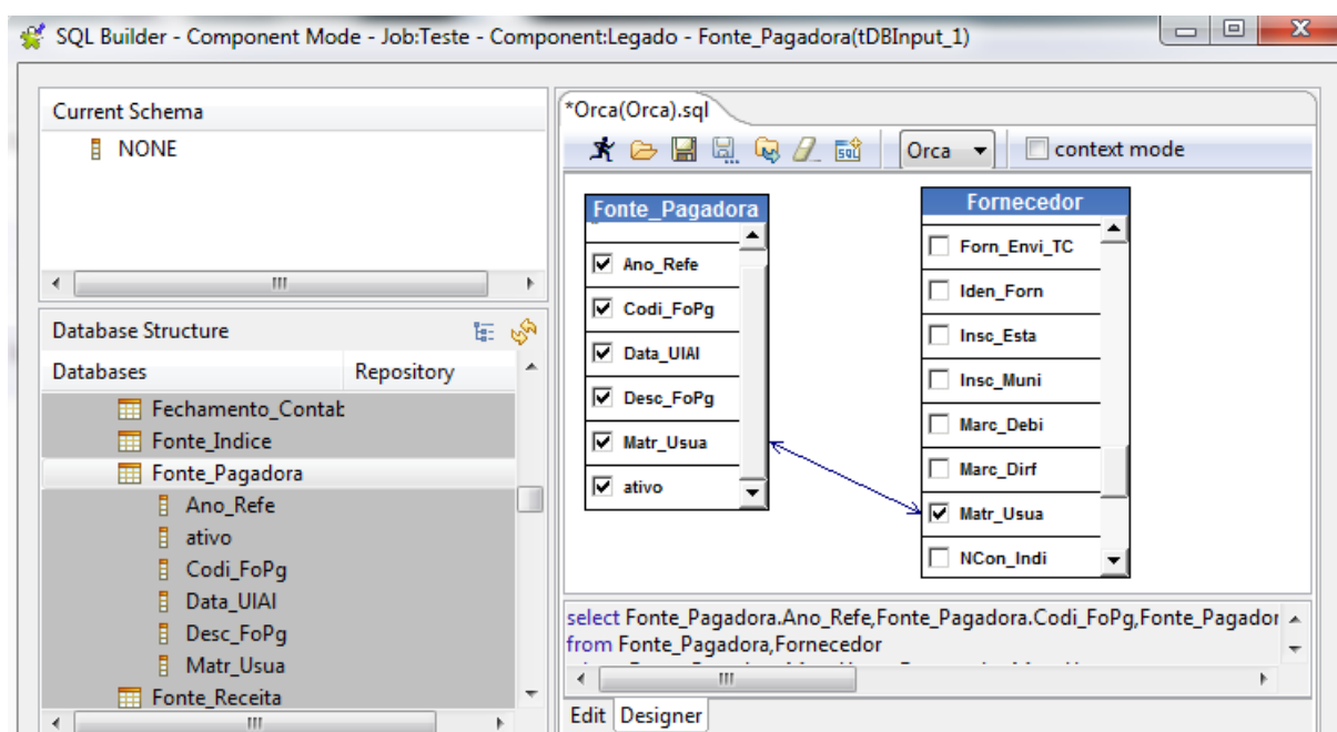
Figura 38 - Tela de geração do SQL de extração dos dados através de um editor gráfico no Talend
