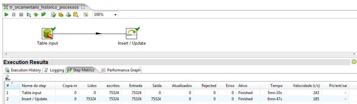
Figura 43 - Transformação da tabela Historico Processos no Kettle
