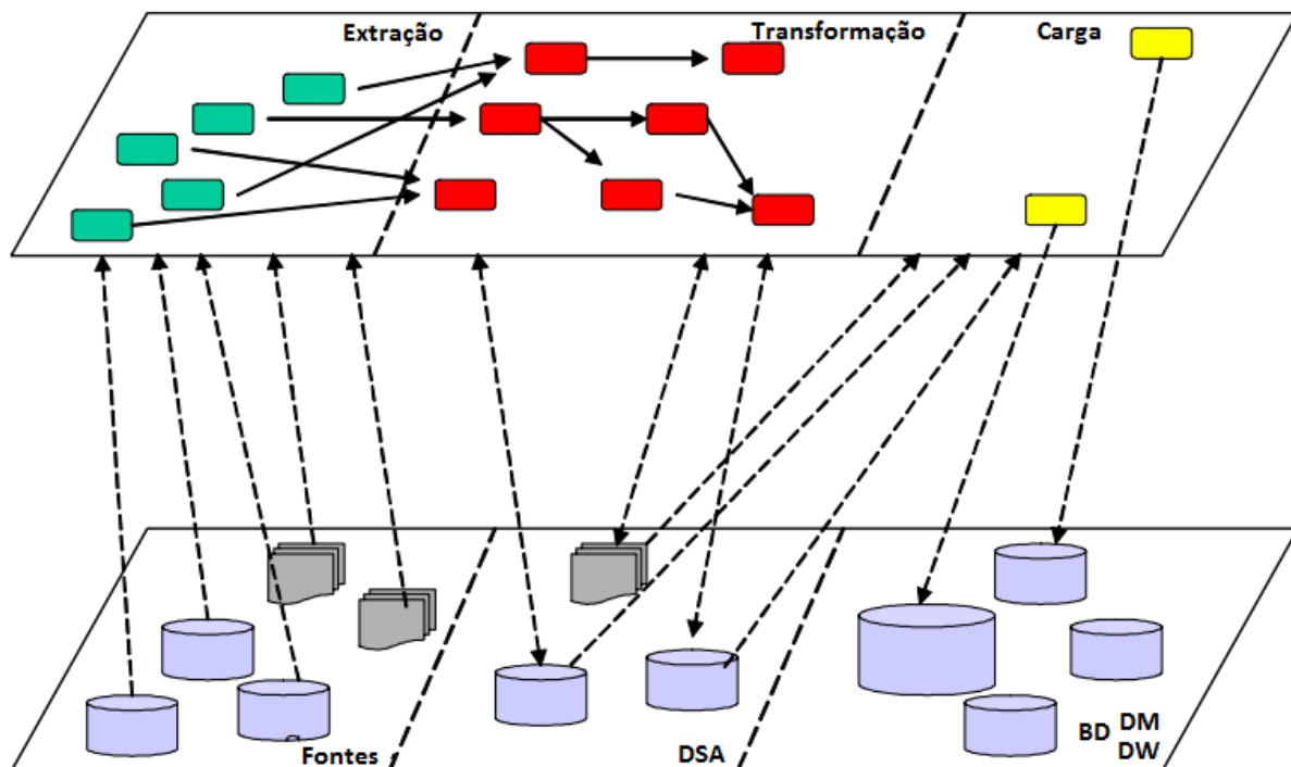
Figura 4 – Processo de ETL, adaptada de Vassiliadis et al. (2002)
