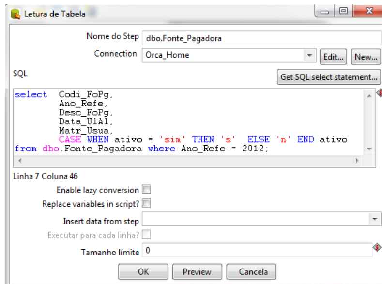
Figura 15 - Step para leitura/seleção dos dados no Kettle conforme a SML1
