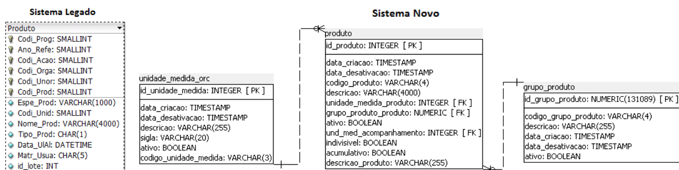
Figura 11 - Modelagem Relacional para migrar dados da tabela Produto
