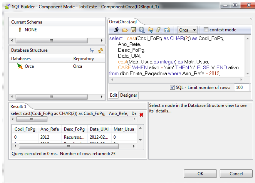
Figura 22 – Parte do step para leitura/seleção dos dados no Talend conforme a SML2
