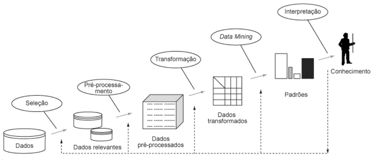
Figura 3 - Etapas do processo de KDD, adaptada de Fayyad et al. (1996b)
