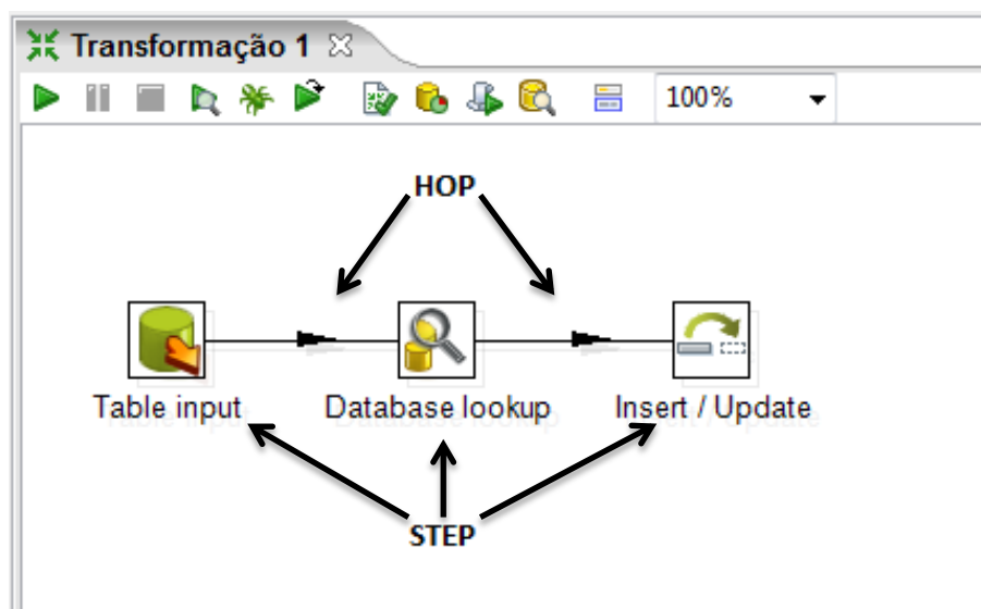
Figura 7 – Transformação no Kettle
