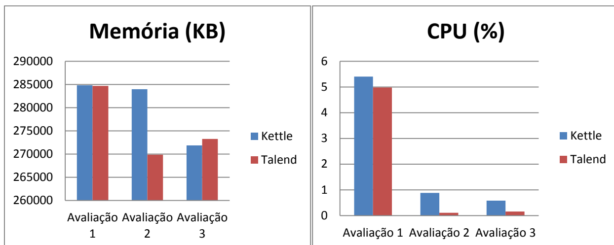
Gráfico 2 - Análise comparativa quanto ao desempenho, tendo como base o acesso a memória e CPU, respectivamente
