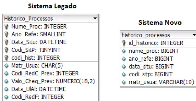
Figura 13 - Modelagem Relacional para migrar dados da tabela Historico Processos
