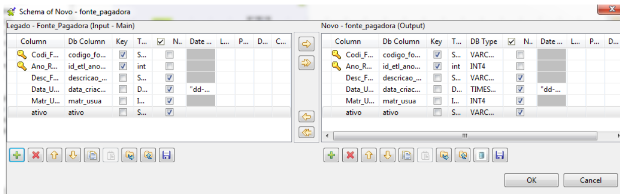
Figura 18 - Parte do step com o mapeamento dos campos no Talend conforme a SML1
