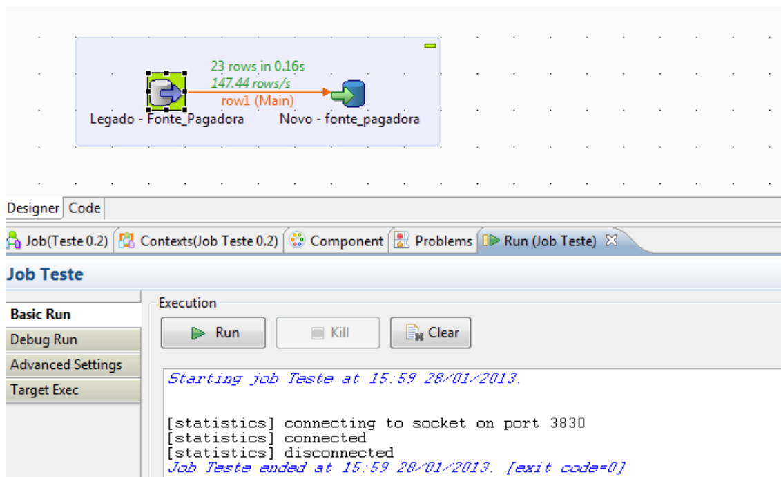
Figura 20 - Job executado no Talend conforme a SML1
