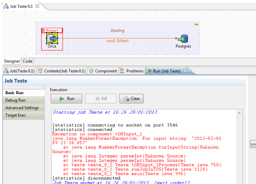
Figura 26 - Job executado no Talend conforme SML2
