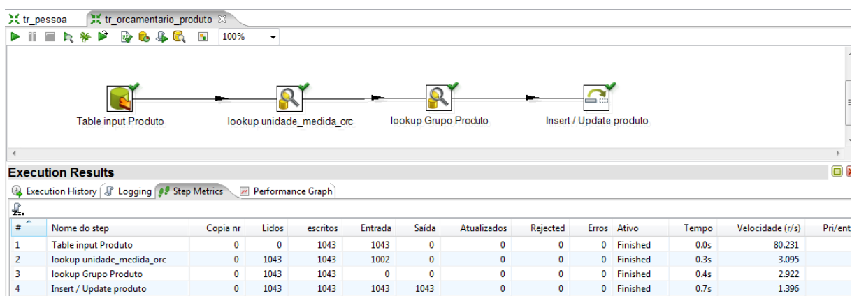
Figura 39 - Transformação da tabela Produto no Kettle
