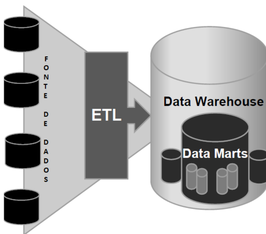
Figura 1 – Estrutura de um Data Warehouse , adaptada de Barbieri (2001)
