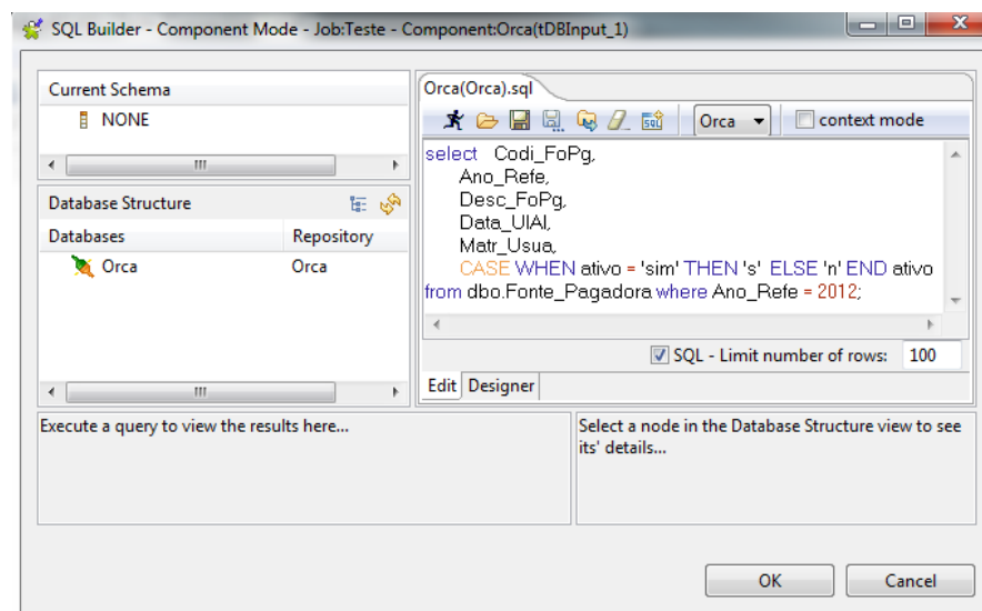
Figura 16 – Parte da estrutura do step para leitura/seleção dos dados no Talend conforme a SML1
