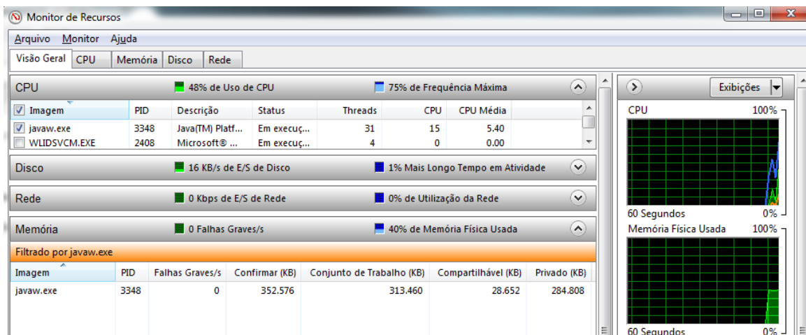
Figura 40 - Monitoramento da transformação da tabela Produto no Kettle, adaptada da ferramenta Monitor de Recursos
