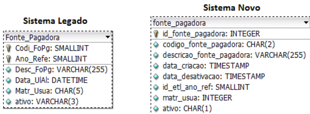
Figura 10 - Modelagem Relacional para migrar dados da tabela Fonte Pagadora
