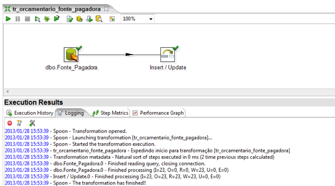
Figura 25 - Transformação executada no Kettle conforme a SML2
