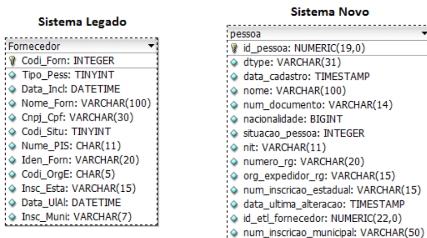
Figura 12 - Modelagem Relacional para migrar dados entre as tabelas Fornecedor e Pessoa
