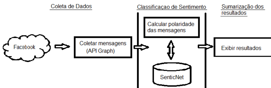
Figura 5 - Arquitetura do sistema desenvolvido.
