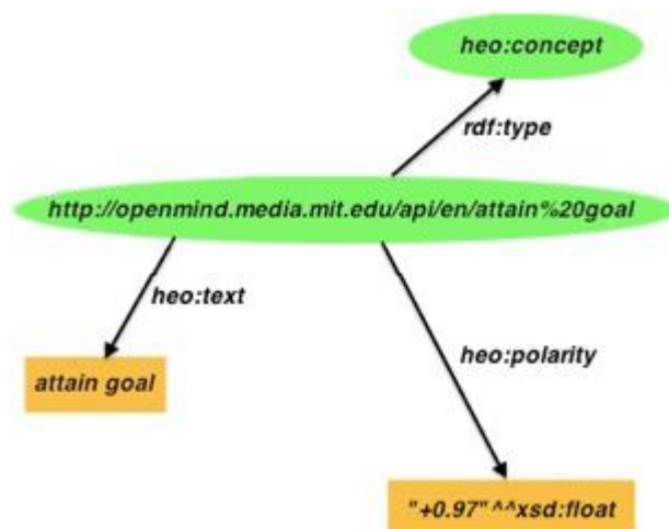
Figura 4 - Modelo de um conceito do SenticNet no formato RDF/XML.
