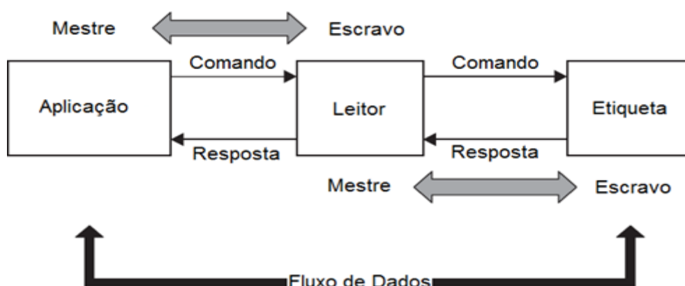
Figura 4. Princípio de funcionamento mestre-escravo usado em leitores RFID.
