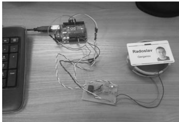
Figura 6. Leitor de clonagem baseado em Arduino.
