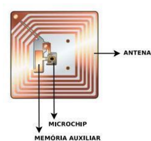
Figura 2. Exemplo de uma Tag RFID.
