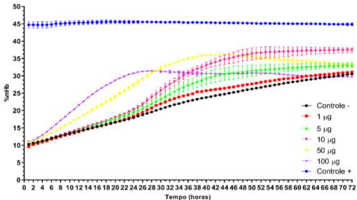
Figura 8 – Efeito oxidante causado pela presença de diferentes quantidades da peçonha bruta de Bothrops jararacussu sobre hemoglobinas provenientes de um concentrado de eritrócitos humano do tipo O+ (solHb-CE) a 5%.
