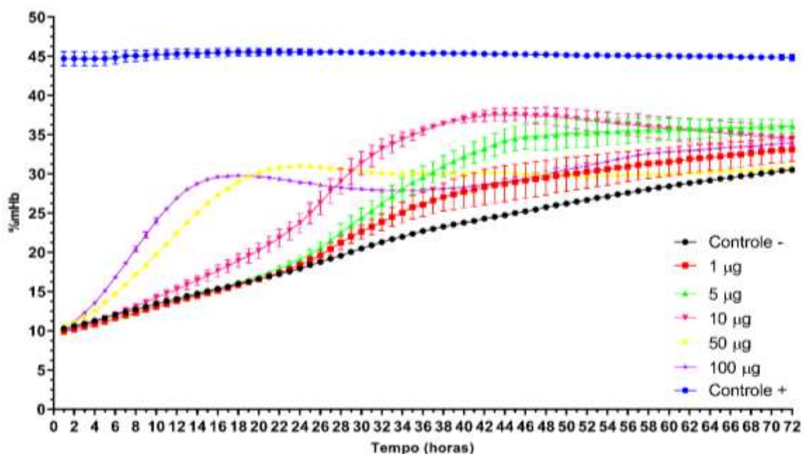
Figura 10 – Efeito oxidante causado pela presença de diferentes quantidades da peçonha bruta de Bothrops moojeni sobre hemoglobinas provenientes de um concentrado de eritrócitos humano do tipo O+ (solHb-CE) a 5%.
