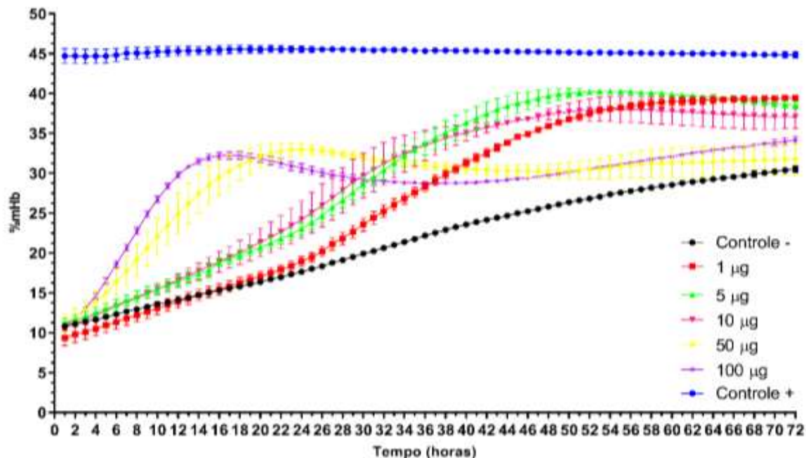
Figura 11 - Efeito oxidante causado pela presença de diferentes quantidades da peçonha bruta de Bothrops moojeni sobre hemoglobinas provenientes do sangue total humano do tipo O+ (solHb-ST) a 10%.
