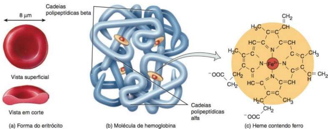
Figura 5 – A forma do eritrócito e a molécula de hemoglobina
