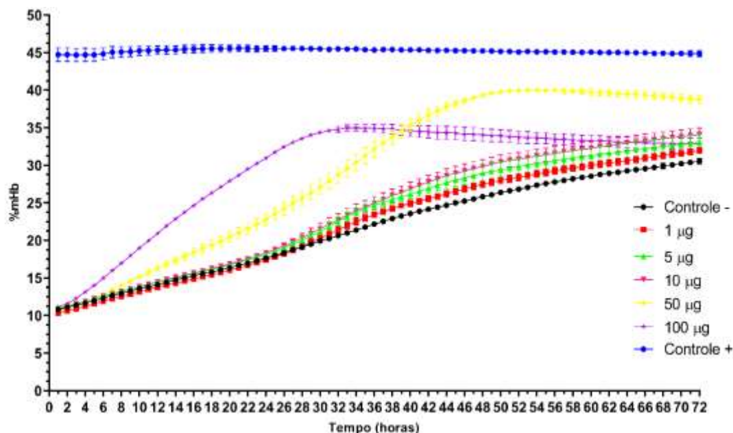
Figura 7 – Efeito oxidante causado pela presença de diferentes quantidades da peçonha bruta de Bothrops alternatus sobre hemoglobinas provenientes de sangue total humano do tipo O+ (solHb-ST) a 10%.
