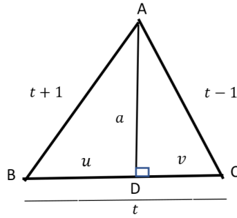
Figura 3.6.1: os conjugados pitagóricos nos triângulos de Brahmagupta.
