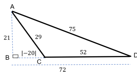
Figura 4.3.1: triângulo (23) - aritmético obtusângulo
