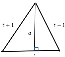
Figura 3.1.1: O triângulo de Brahmagupta
