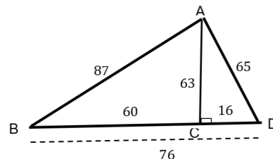
Figura 4.3.3: triângulo (11)- aritmético acutângulo
