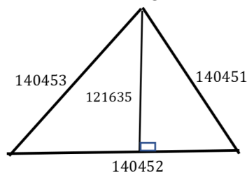
Figura 3.3.1: O 9º triângulo de Brahmagupta
