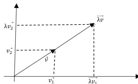
Figura 9.1.1 - Transformação Linear
