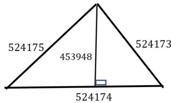
Figura 3.3.2: O 10º triângulo de Brahmagupta
