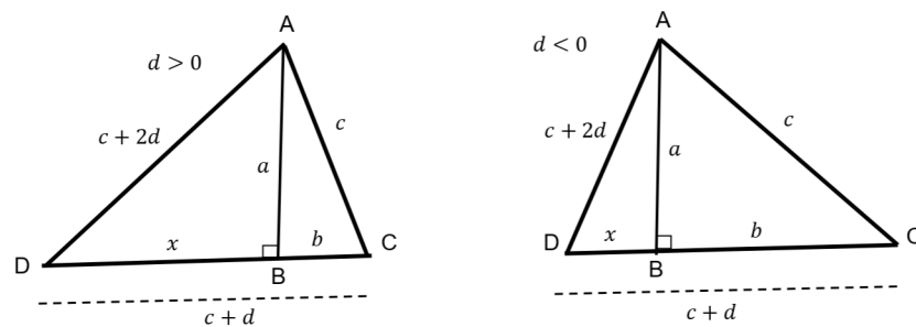
Figura 4.1.1-Triângulos acutângulos aritméticos
