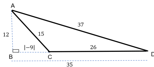
Figura 4.2.1: triângulo (11)-aritmético
