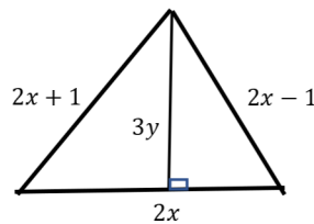
Figura 3.1.2: Um Triângulo de Brahmagupta.
