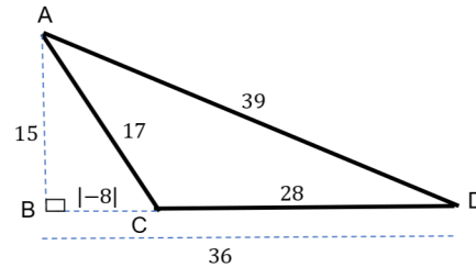
Figura 4.3.2: triângulo (11)- aritmético obtusângulo
