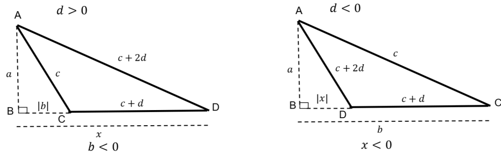
Figura 4.1.2 - Triângulos obtusângulos aritméticos
