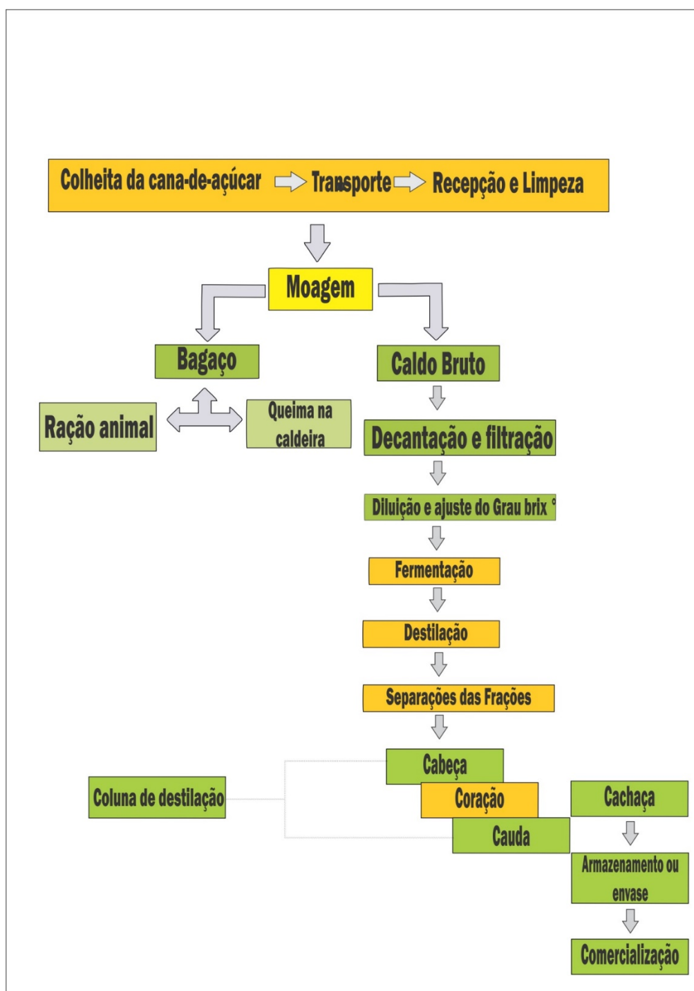
Figura 1- Processo de produção da cachaça
