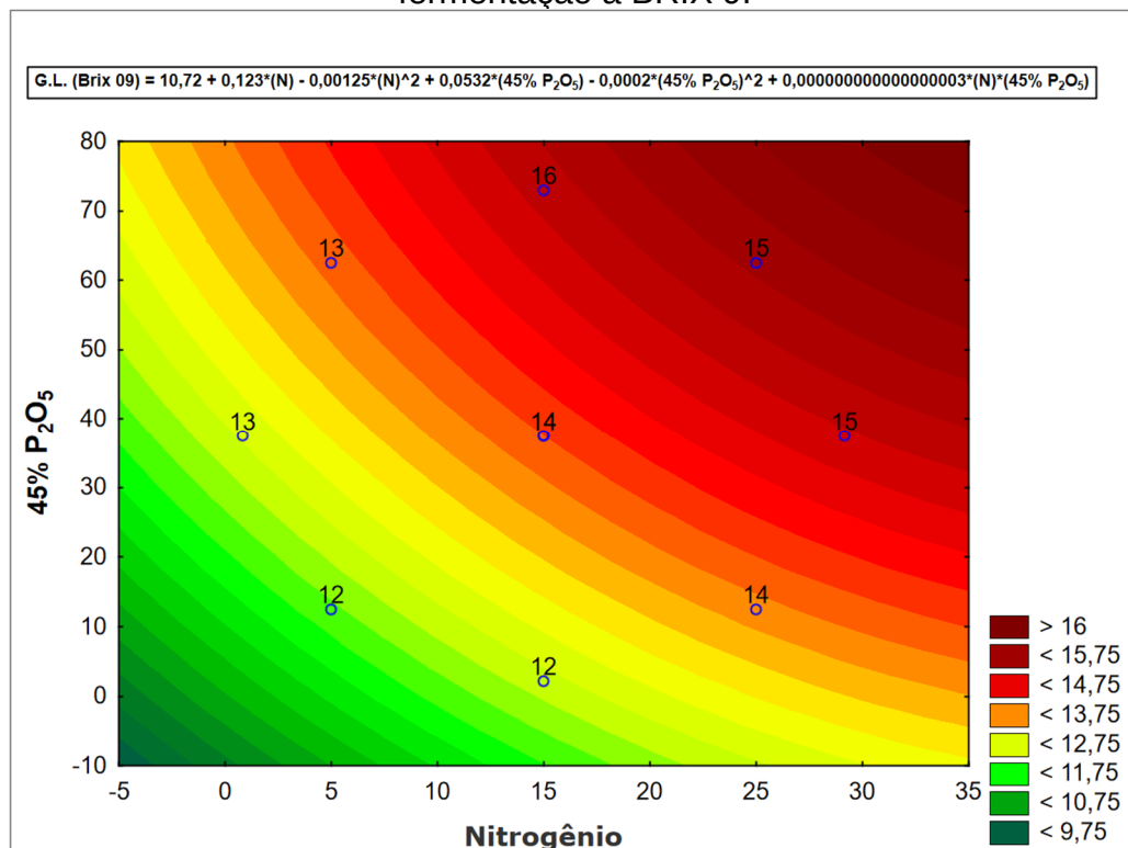
Figura 14- Curvas de contorno do teor alcoólico G.L, obtido a partir da fermentação a BRIX 9.
