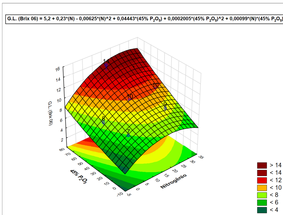
Figura 11 --Superfície de resposta do teor alcoólico G.L, obtido a partir da fermentação a BRIZ 6.
