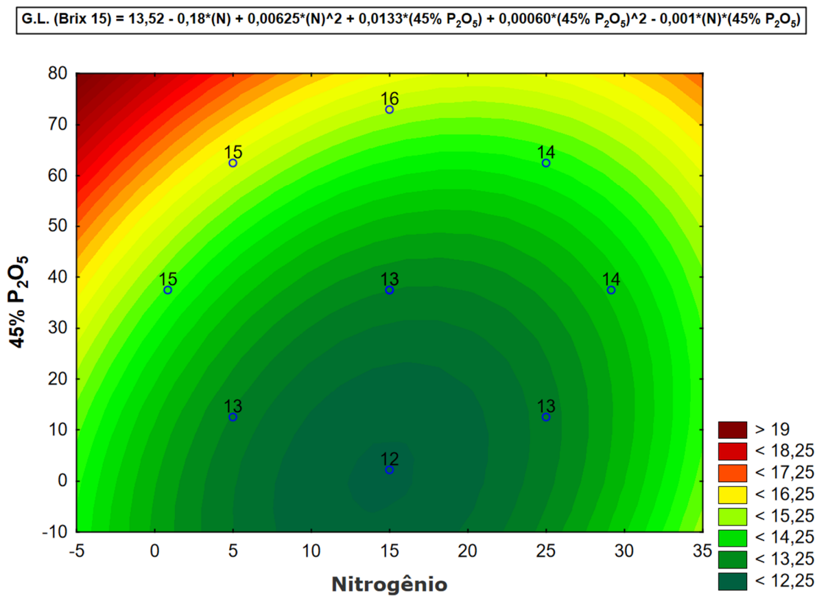
Figura 18- Curvas de contorno do teor alcoólico G.L, obtido a partir da fermentação a BRIX 15.
