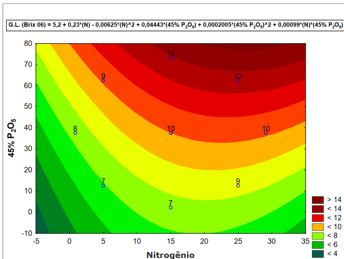
Figura 12- Curvas de contorno do teor alcoólico G.L, obtido a partir da fermentação a BRIX 6
