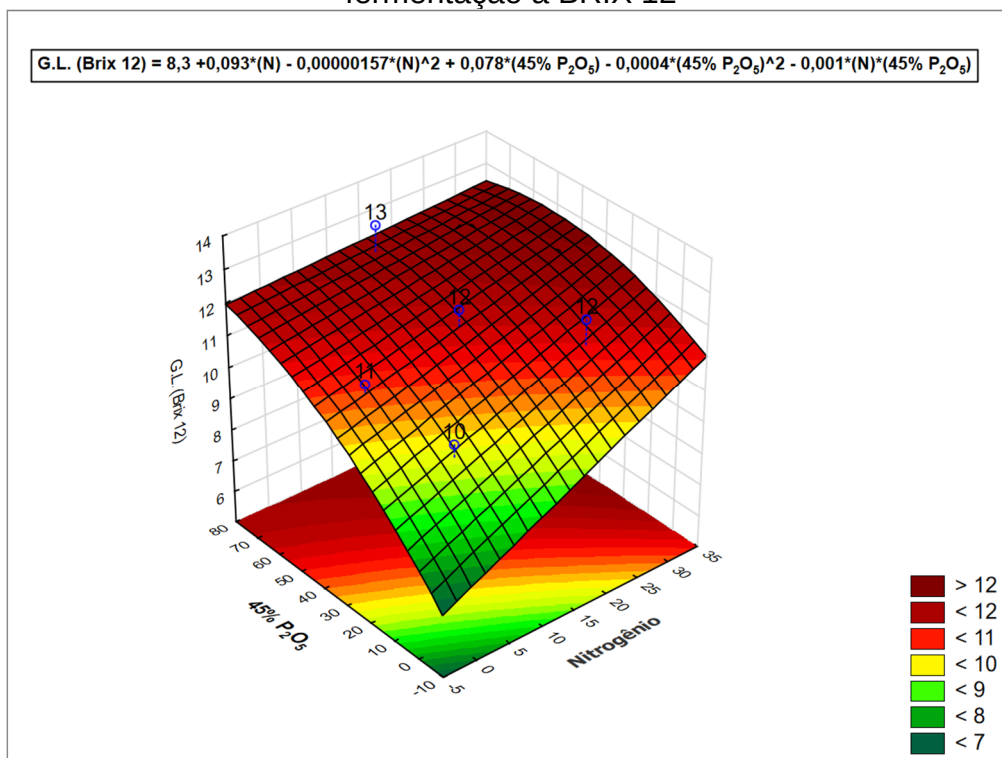
Figura 15-- Superfície de resposta do teor alcoólico G.L, obtido a partir da fermentação a BRIX 12
