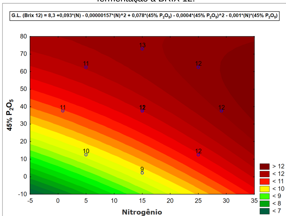
Figura 16- Curvas de contorno do teor alcoólico G.L, obtido a partir da fermentação a BRIX 12.
