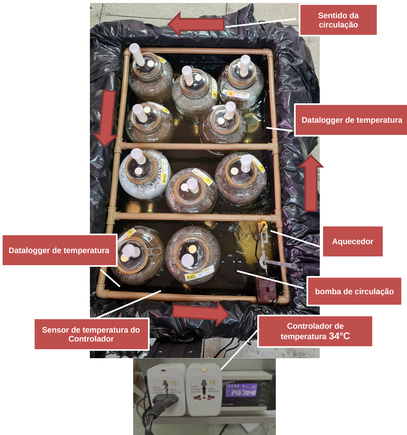
Figura 8- Fermentação alcoólica com temperatura controlada a 34°C
