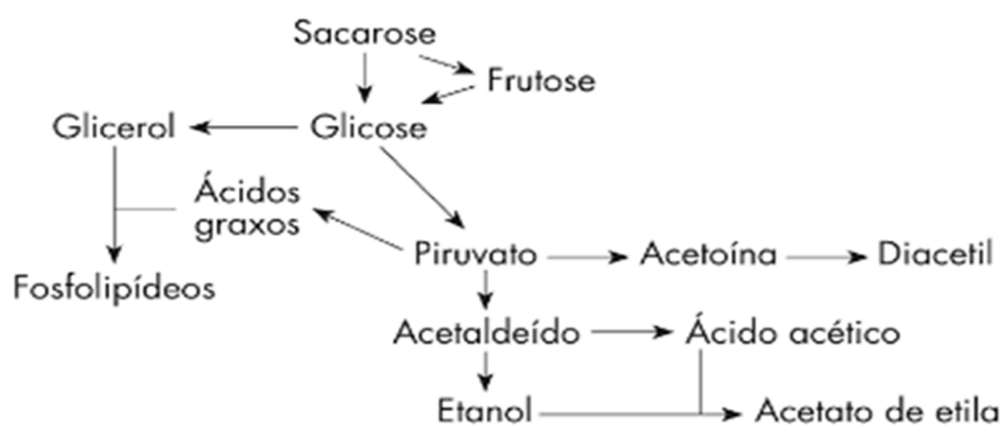
Figura 2 - Reações que ocorrem no processo de fabricação da cachaça que influenciam no sabor e odor do produto
