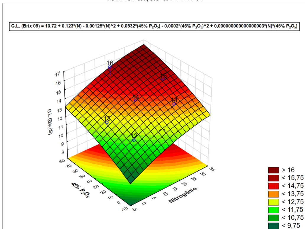
Figura 13-- Superfície de resposta do teor alcoólico G.L, obtido a partir da fermentação a BRIX 9.
