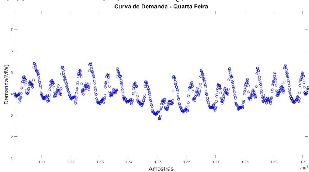
FIGURA 28: CURVA DE DEMANDA ORIGINAL PARA A QUARTA FEIRA
