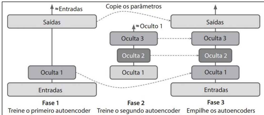
FIGURA 13: TREINANDO UM AUTOENCODER DE CADA VEZ.
