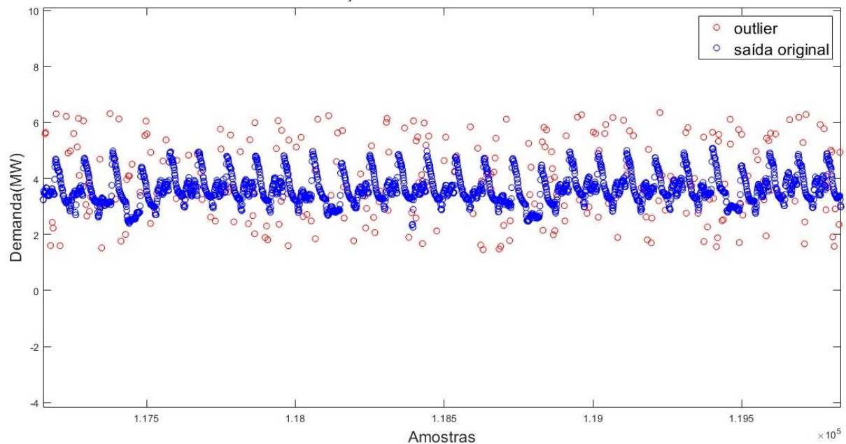
FIGURA 16: PIOR CENÁRIO DE INSERÇÃO DE OUTLIERS NO BANCO DE DADOS.
