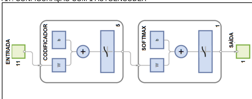
FIGURA 17: CONFIGURAÇÃO COM 1 AUTOENCODER
