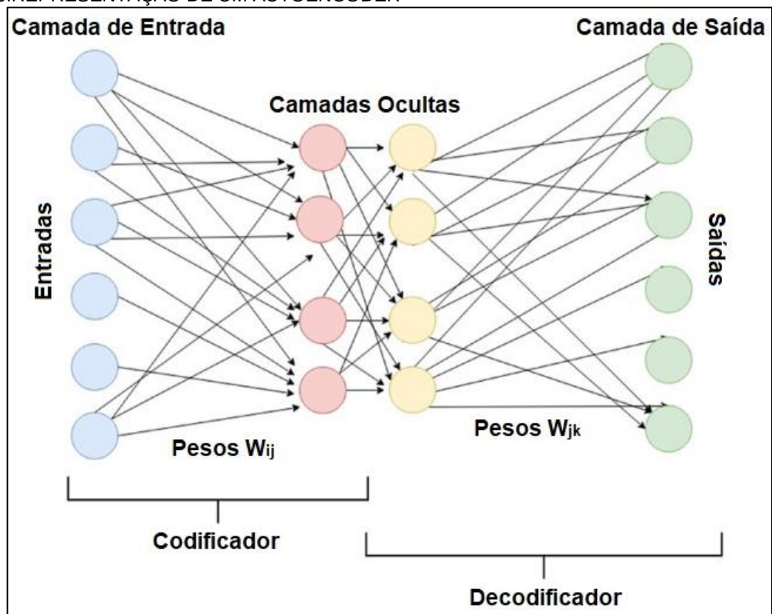
FIGURA 6: REPRESENTAÇÃO DE UM AUTOENCODER
