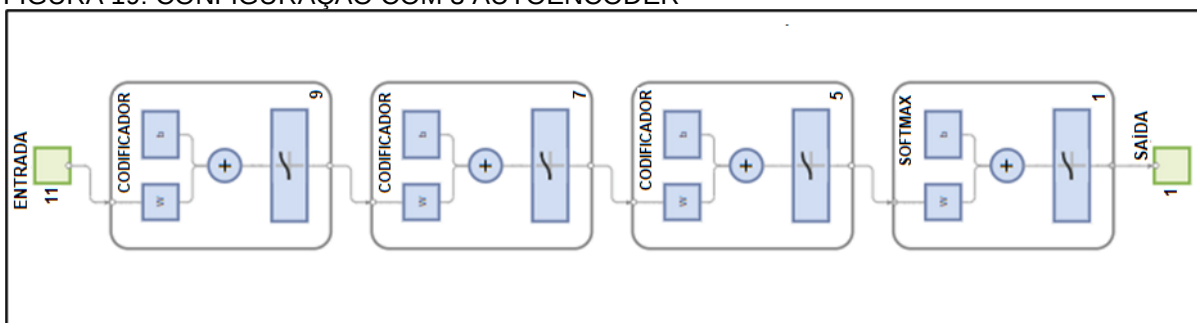
FIGURA 19: CONFIGURAÇÃO COM 3 AUTOENCODER
