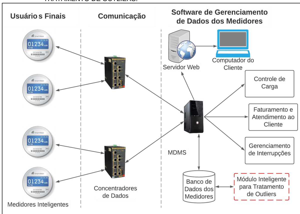
FIGURA 3: TOPOLOGIA PROPOSTA COM INSERÇÃO DO MÓDULO INTELIGENTE PARA TRATAMENTO DE OUTLIERS.
