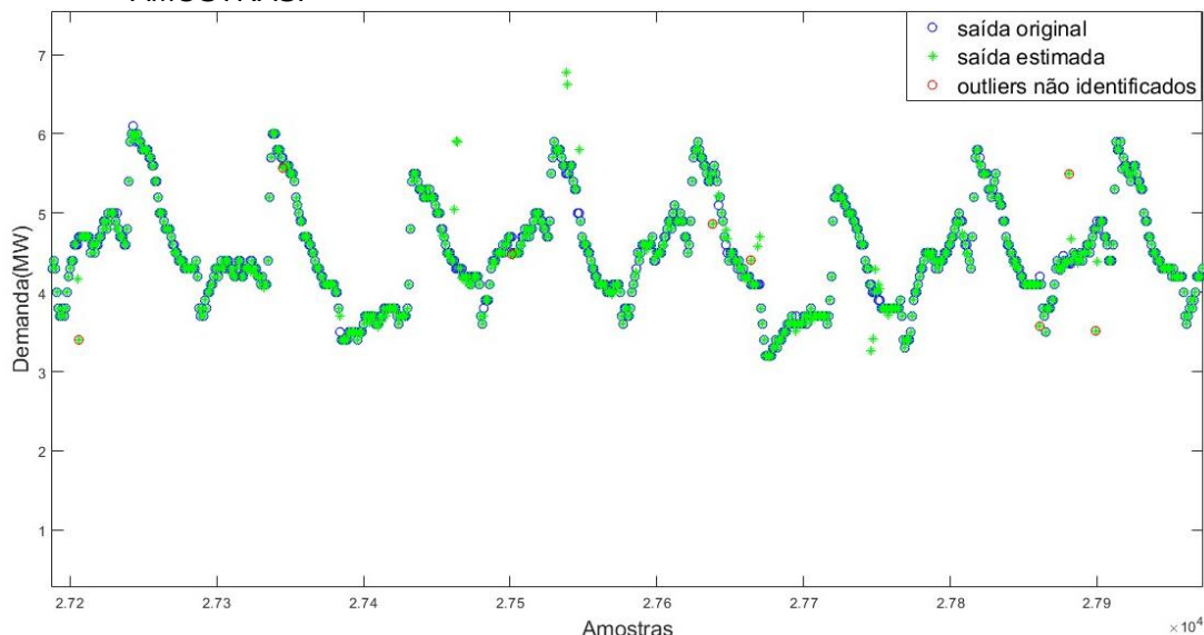
FIGURA 25: CENÁRIO COM NÚMERO DE OUTLIERS EQUIVALENTE A 10% DO TOTAL DE AMOSTRAS.
