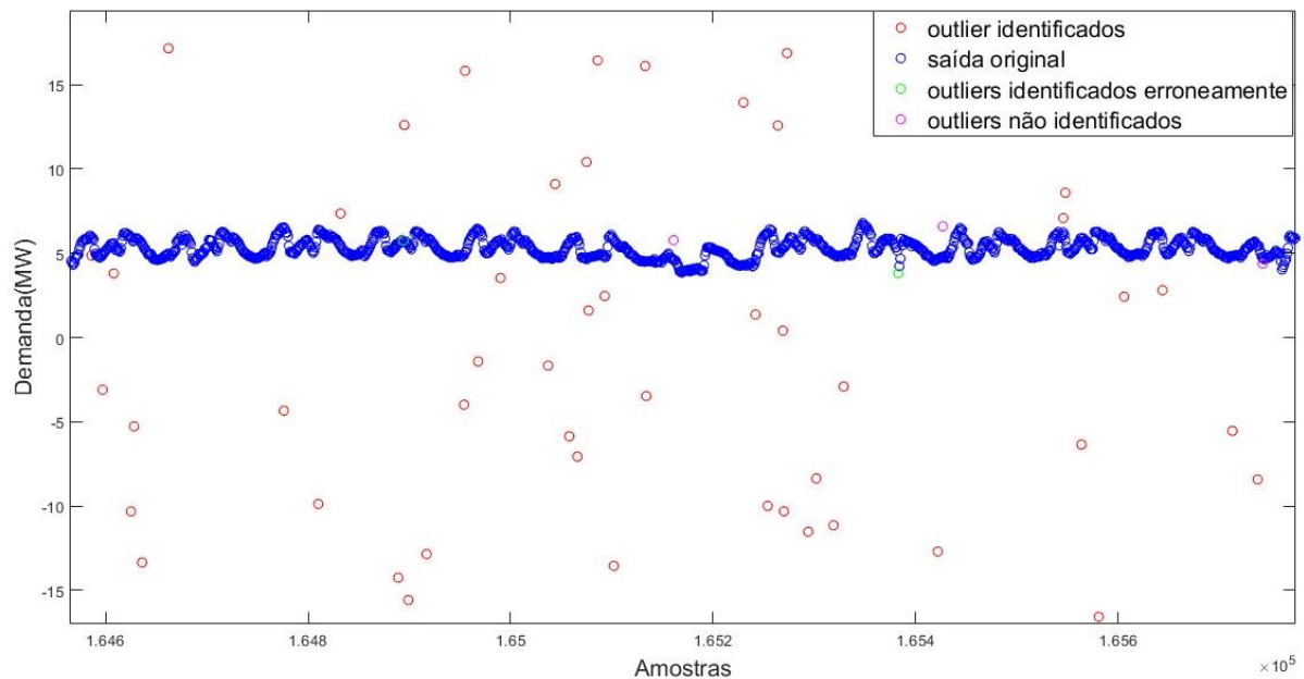
FIGURA 22: CENÁRIO COM NÚMERO DE OUTLIERS EQUIVALENTE A 5% DE L.
