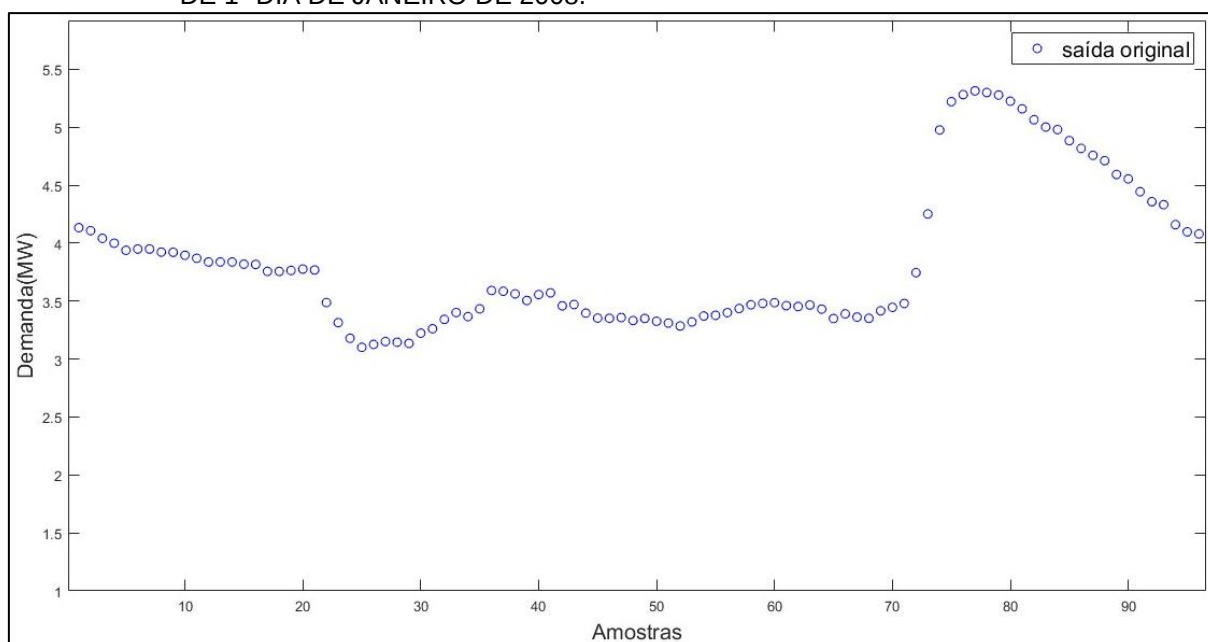
FIGURA 14: GRÁFICO DE PARTE DA CURVA DE DEMANDA COM 96 AMOSTRAS REFERENTE DE 1º DIA DE JANEIRO DE 2008.
