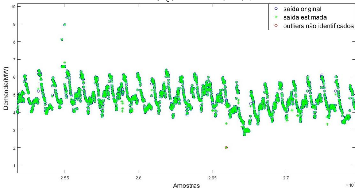
FIGURA 26: CENÁRIO PARA O QUAL AS AMPLITUDES DOS OUTLIERS ESTÃO CONTIDAS NO INTERVALO QUE VARIA DE 0 A 25% DE P MAX .
