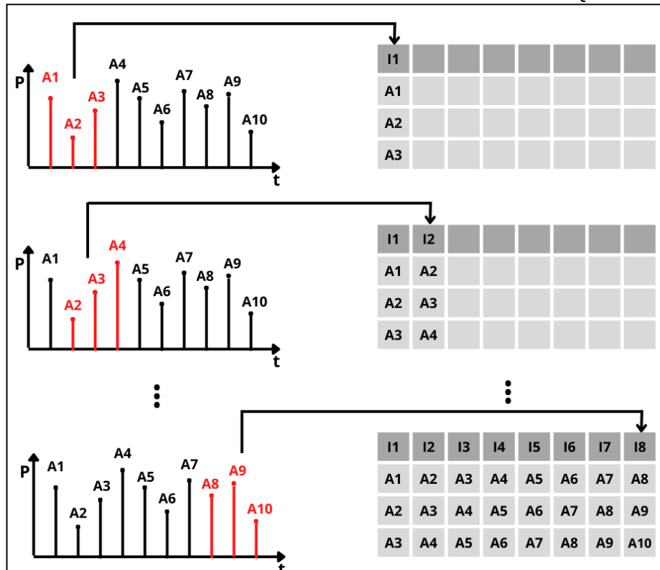
FIGURA 9: ORGANIZANDO OS DADOS DE ENTRADA NA ME COM L = 10 E Q = 3
