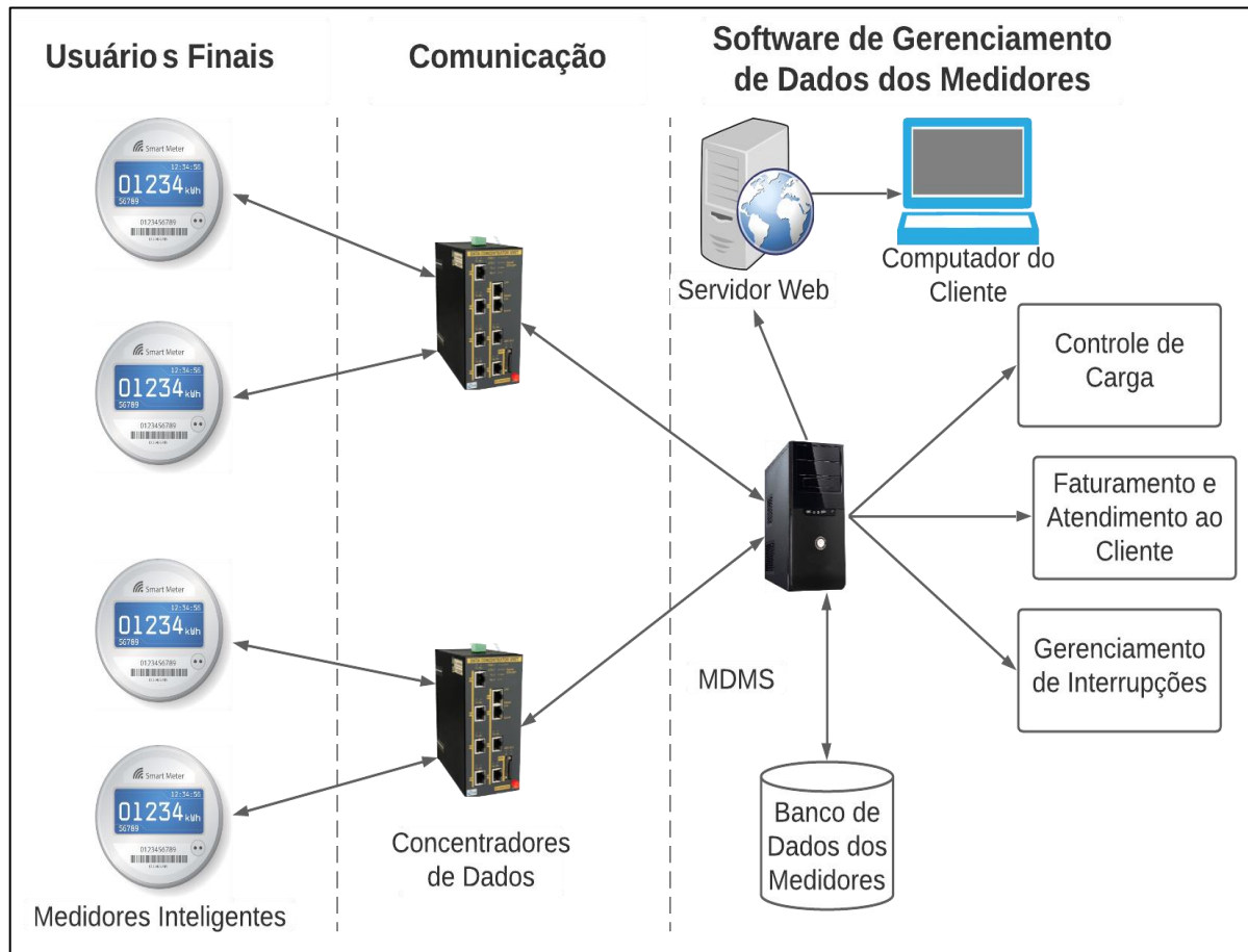
FIGURA 2: ESTRUTURA TÍPICA DE UMA AMI.
