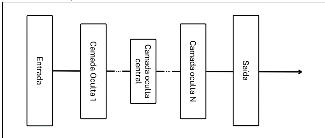
FIGURA 10: DIAGRAMA DO AUTOENCODER UTILIZADO NO ALGORITMO DE DETECÇÃO E CORREÇÃO DE OUTLIERS.
