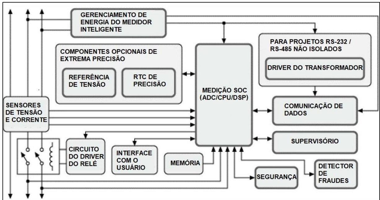
FIGURA 4: DIAGRAMA DE BLOCO DE UM TÍPICO SMART METER.
