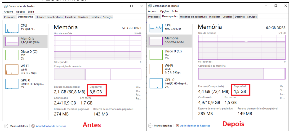
FIGURA 21: ESTIMANDO A QUANTIDADE DE RAM SOLICITADA PARA EXECUÇÃO DOS ALGORITMOS.
