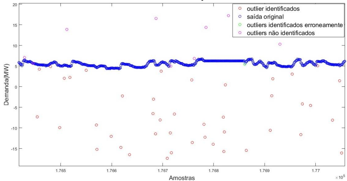
FIGURA 23: CENÁRIO COM NÚMERO DE OUTLIERS EQUIVALENTE A 2% DE L.
