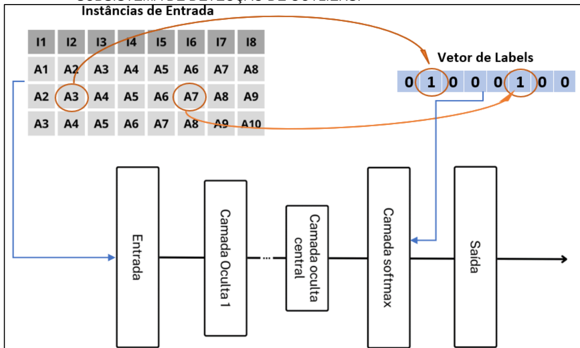
FIGURA 12: REPRESENTAÇÃO DO PROCESSO DE TREINAMENTO DA REDE NEURAL DO SUBSISTEMA DE DETECÇÃO DE OUTLIERS.
