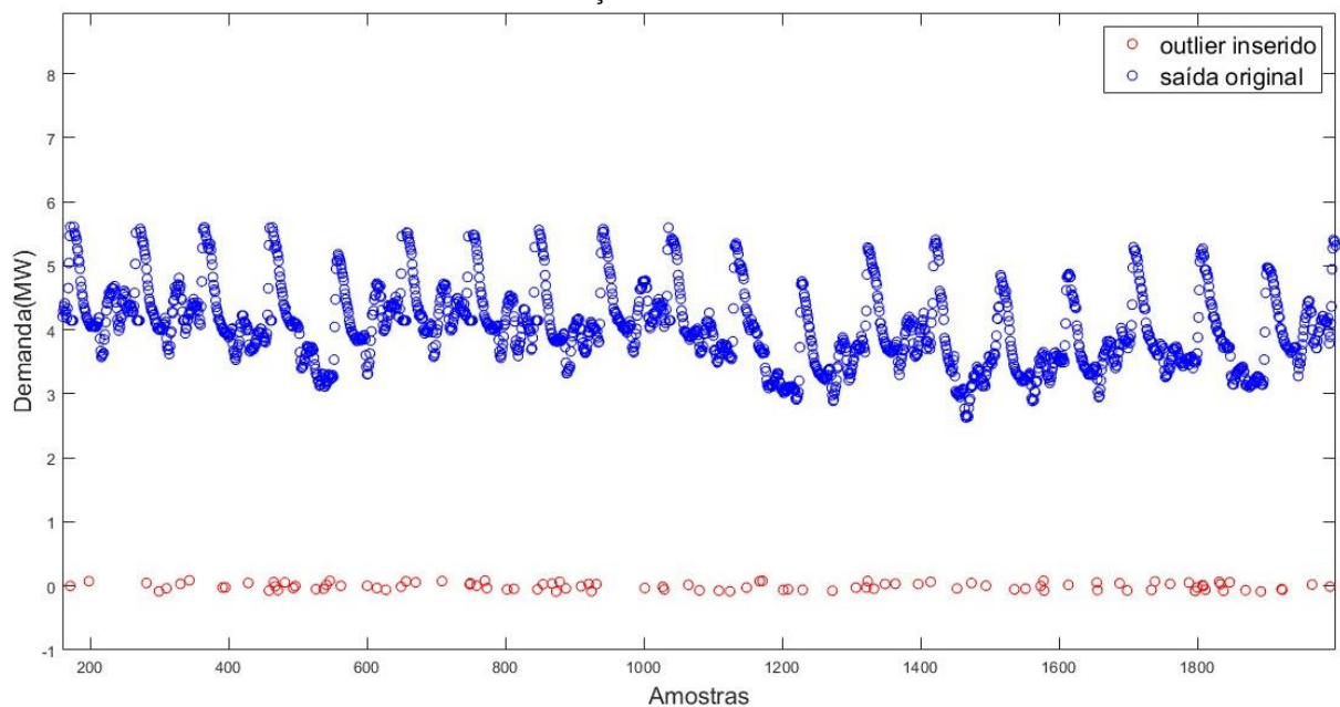
FIGURA 15: MELHOR CENÁRIO DE INSERÇÃO DE OUTLIERS NO BANCO DE DADOS.
