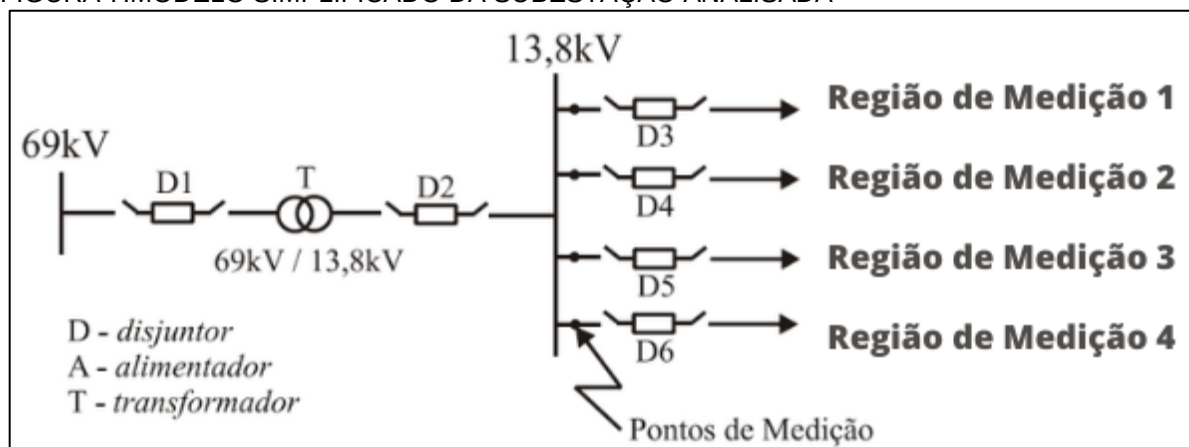
FIGURA 7: MODELO SIMPLIFICADO DA SUBESTAÇÃO ANALISADA
