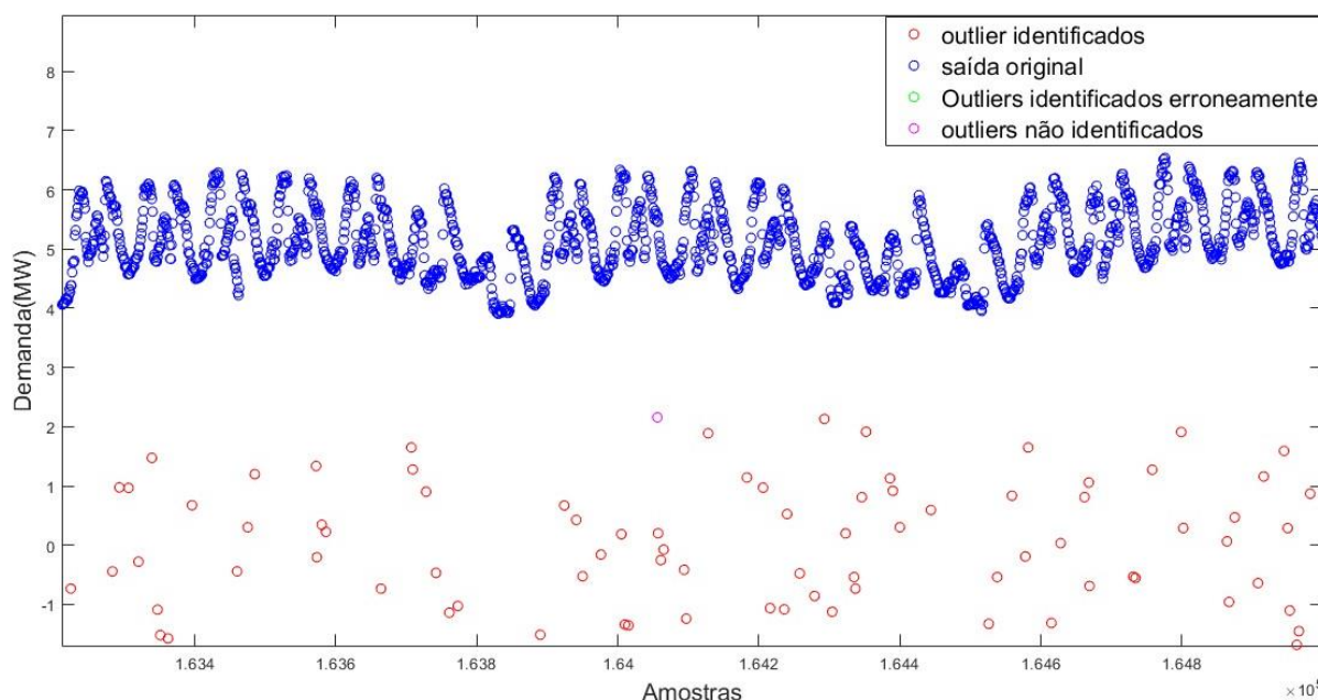
FIGURA 24: CENÁRIO PARA O QUAL AS AMPLITUDES DOS OUTLIERS ESTÃO CONTIDAS NO INTERVALO QUE VARIA DE 0 A 25% DE P MAX .
