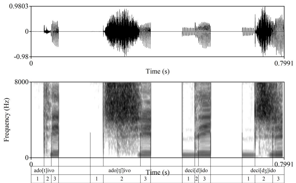
Figura 4 - De cima para baixo, forma de onda, espectrograma de banda larga e camadas com a delimitação dos segmentos produzidos pela informante desta pesquisa
