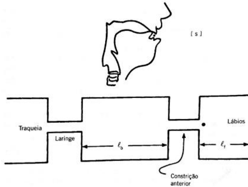
Figura 2 - Modelo idealizado do trato vocal para a fricativa /s/
