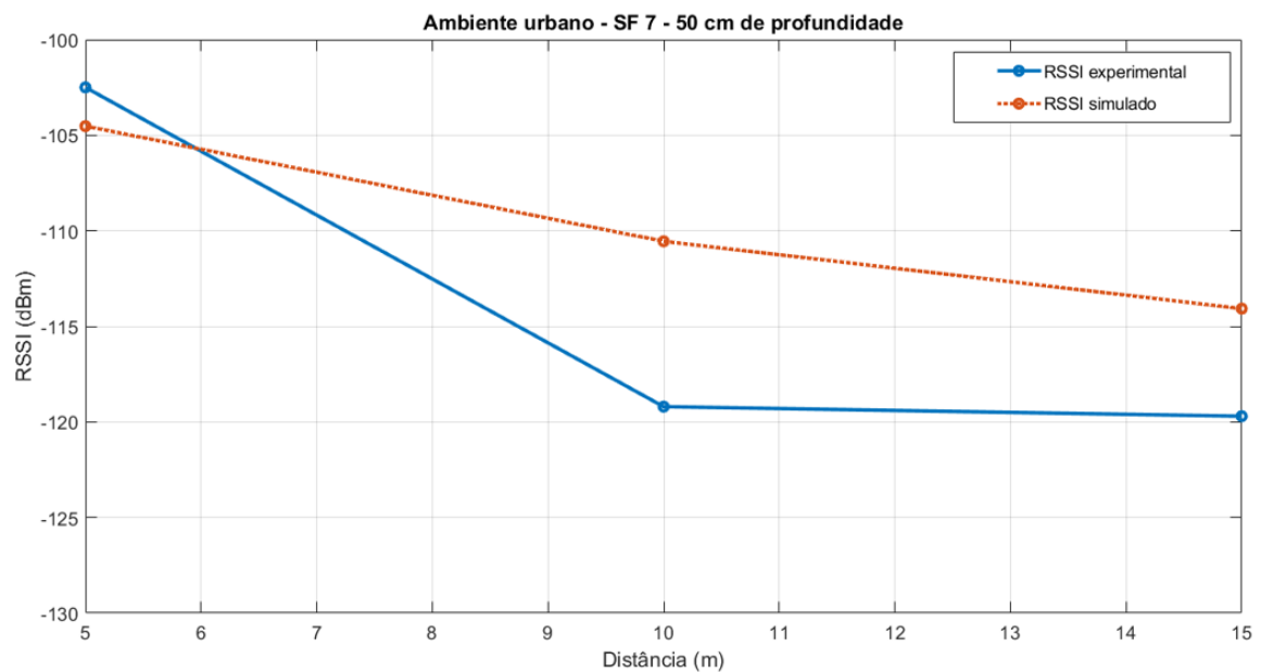
Figura 35 – Relação entre RSSI e a distância comparando valor experimental com resultado simulado para ambiente urbano denso e profundidade igual a 50 cm.
