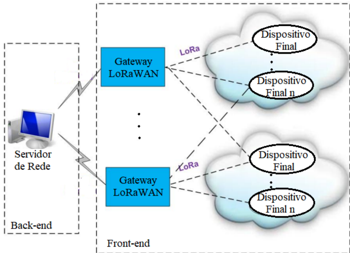
Figura 12 – Arquitetura de uma rede LoRa.
