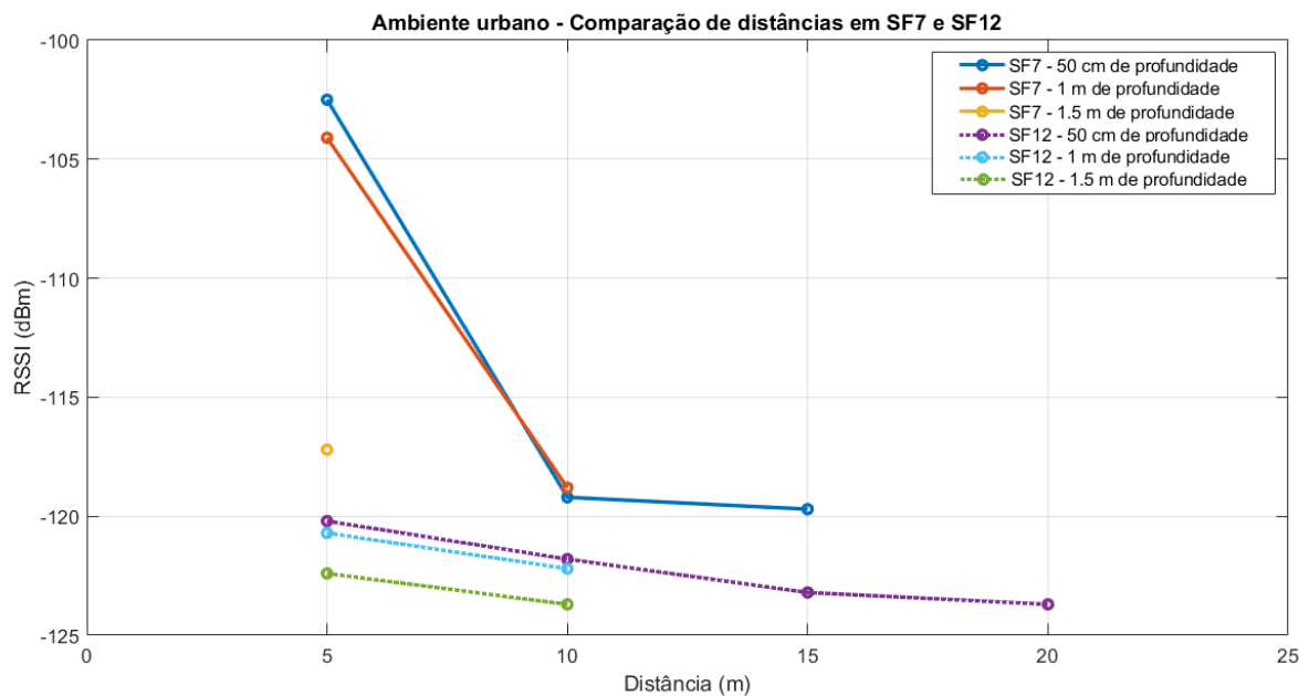
Figura 37 – Relação entre RSSI e a Distância comparando diferentes valores de fator de espalhamento e de profundidade para ambiente urbano denso.
