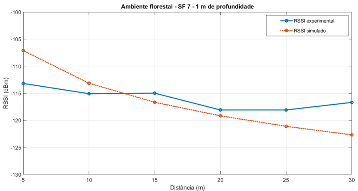
Figura 34 – Relação entre RSSI e a distância comparando valor experimental com resultado simulado para ambiente florestal e profundidade igual a 1 m.
