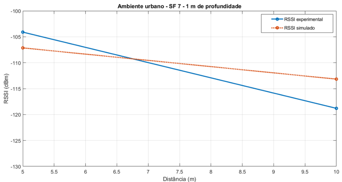
Figura 36 – Relação entre RSSI e a distância comparando valor experimental com resultado simulado para ambiente urbano denso e profundidade igual a 1 m.
