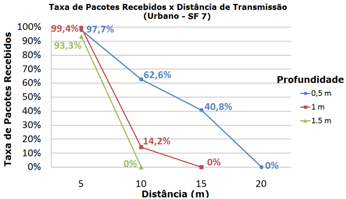
Figura 27 – Relação entre a Taxa de Pacotes Recebidos e a Distância de acordo com a profundidade em ambiente urbano denso e SF = 7.
