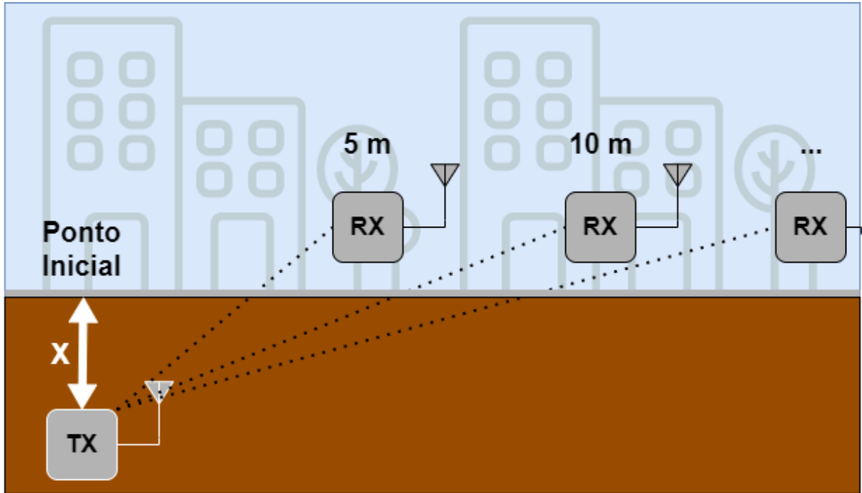
Figura 17 – Experimento realizado para testes da tecnologia de comunicação LoRa em ambientes subterrâneos.
