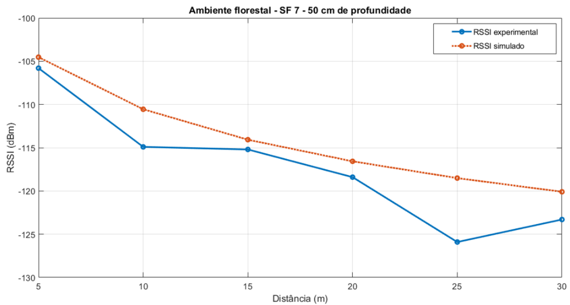
Figura 33 – Relação entre RSSI e a distância comparando valor experimental com resultado simulado para ambiente florestal e profundidade igual a 50 cm.
