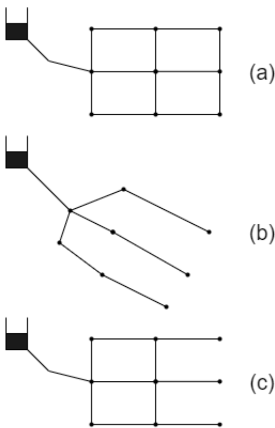
Figura 4 – Traçados da rede de distribuição a) malhada b) ramificada e c) mista
