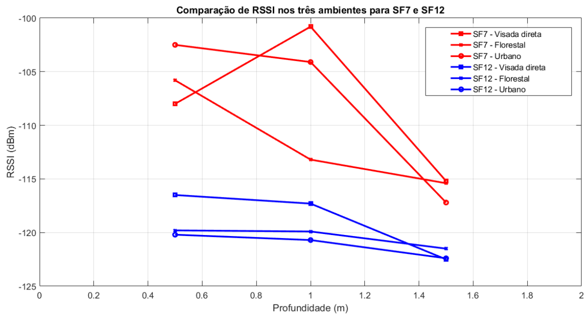
Figura 38 – Relação entre RSSI e a Profundidade comparando diferentes valores de fator de espalhamento e em diferentes cenários em uma distância de 5 metros entre os dispositivos transmissor e receptor.
