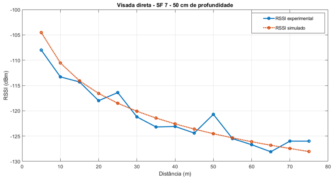
Figura 31 – Relação entre RSSI e a distância comparando valor experimental com resultado simulado para ambiente com visada direta e profundidade igual a 50 cm.
