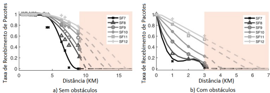
Figura 14 – Experimento realizado para testes da tecnologia de comunicação LoRa em ambientes com e sem obstáculos.
