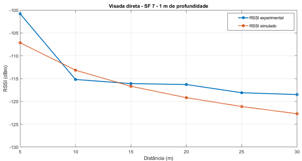
Figura 32 – Relação entre RSSI e a distância comparando valor experimental com resultado simulado para ambiente com visada direta e profundidade igual a 1 m.
