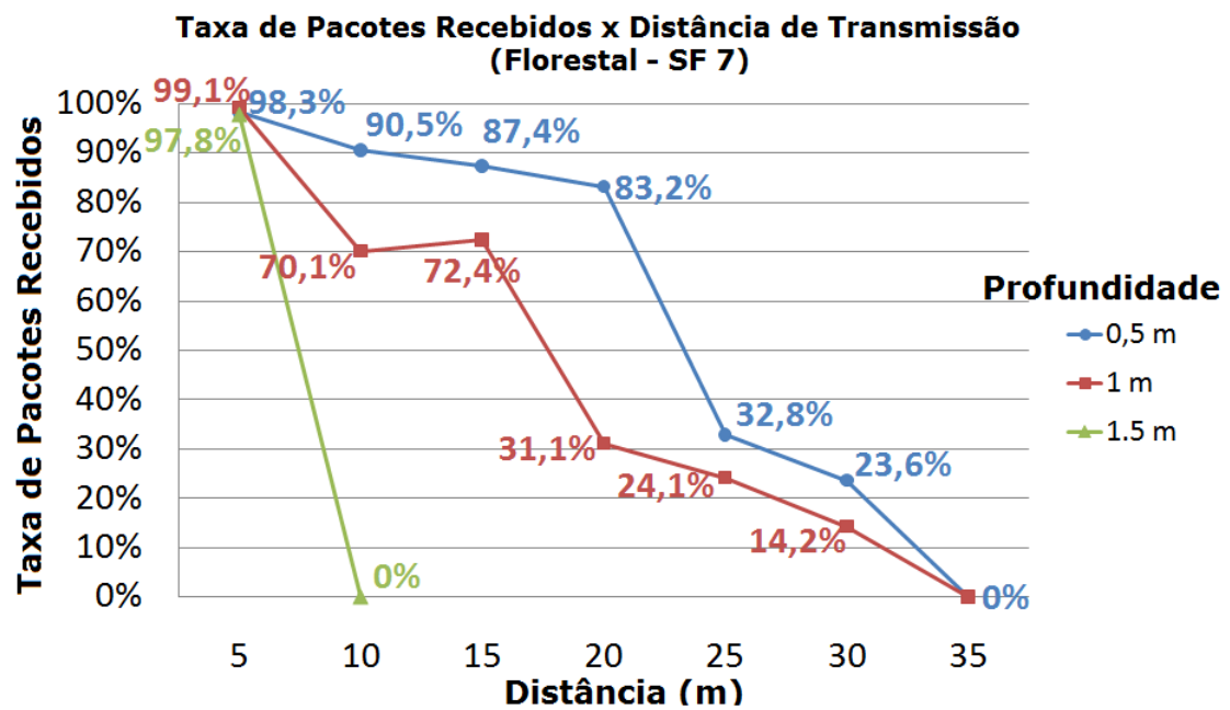
Figura 23 – Relação entre a Taxa de Pacotes Recebidos e a Distância de acordo com a profundidade em ambiente florestal e SF = 7.
