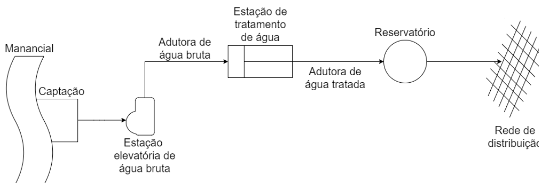
Figura 1 – Esquema básico de um sistema de abastecimento de água
