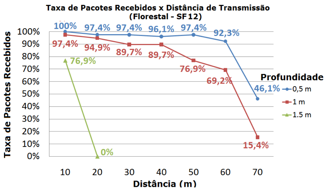
Figura 24 – Relação entre a Taxa de Pacotes Recebidos e a Distância de acordo com a profundidade em ambiente florestal e SF = 12.
