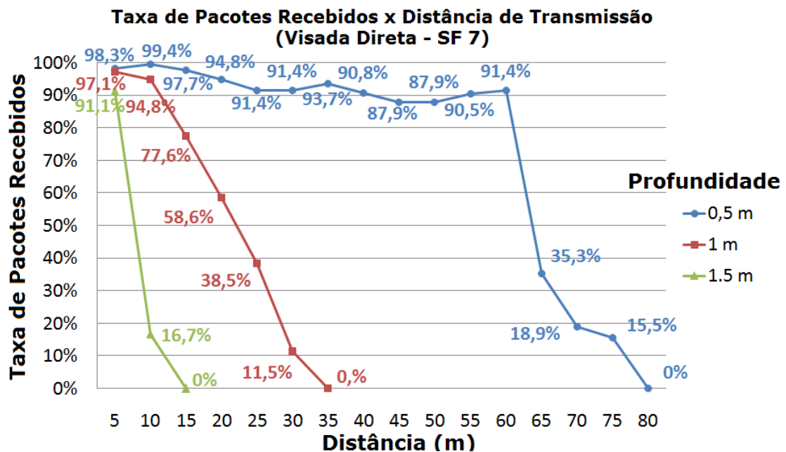
Figura 20 – Relação entre a Taxa de Pacotes Recebidos e a Distância de acordo com a profundidade em ambiente com visada direta e SF = 7.
