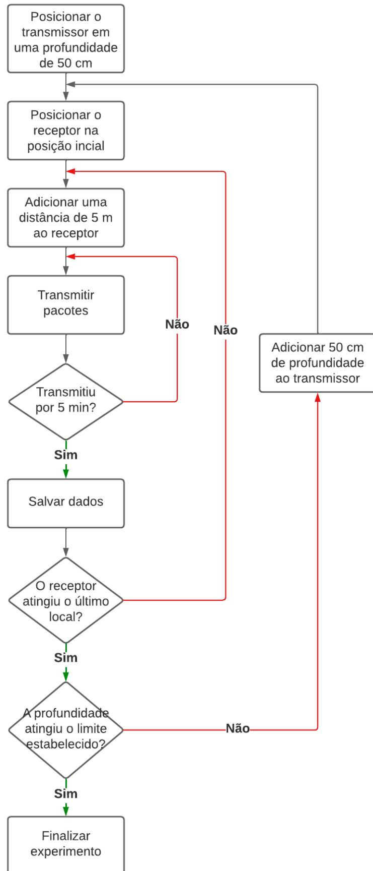
Figura 18 – Fluxograma que apresenta a metodologia do experimento realizado.
