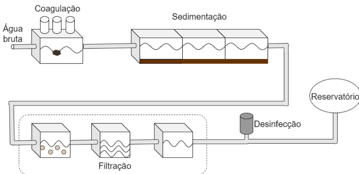
Figura 3 – Esquema do funcionamento básico de uma Estação de Tratamento de Água (ETA)
