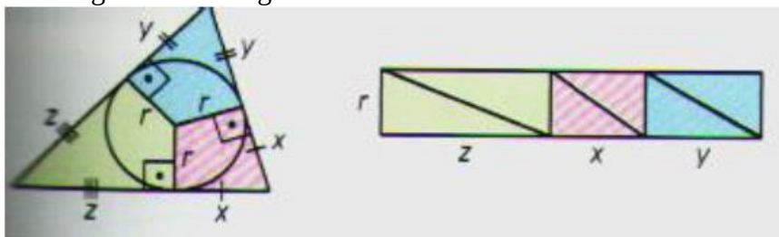
Figura 02: Triângulo circunscrito em uma circunferência
