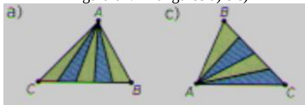
Figura 04: Triângulos a) e c)
