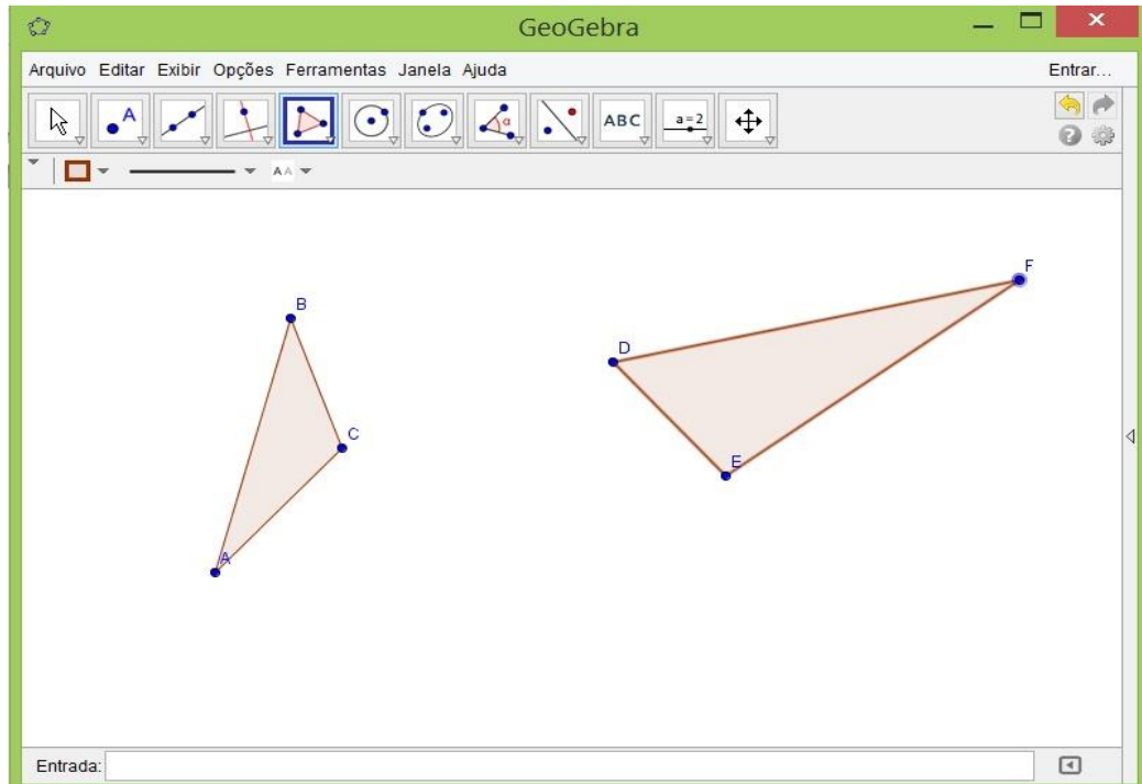
Figura 08- Construção de diversos triângulos a partir de três pontos quaisquer
