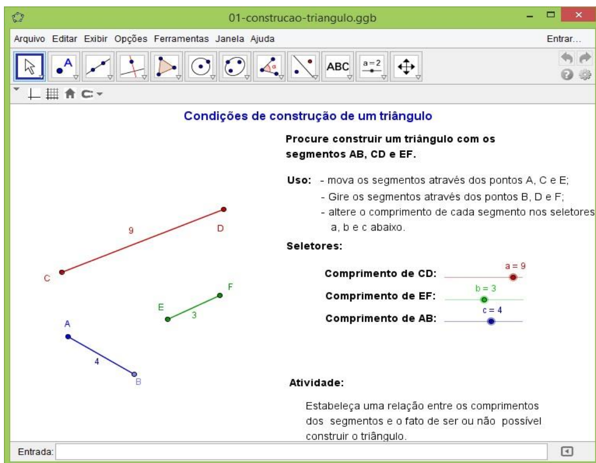
Figura 19 – Objeto de Aprendizagem: Construção de triângulos possíveis
