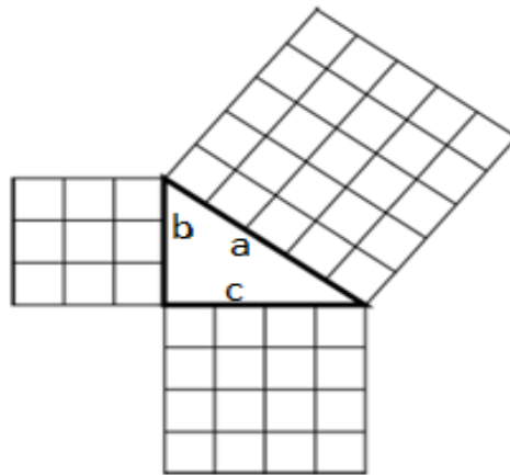
Figura 05 – Representação gráfica do Teorema de Pitágoras a^2 = b^2 + c^2
