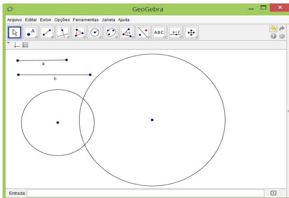
Figura 10 – Duas possíveis circunferências construídas com o GeoGebra
