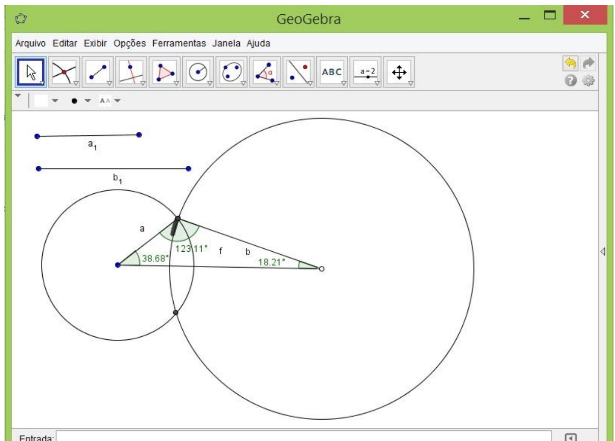
Figura 11 – Formação de um triângulo a partir de dois segmentos dados
