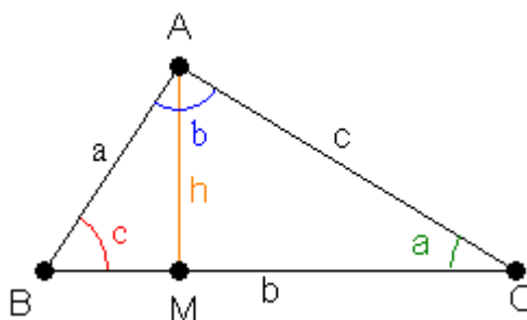
Figura 21: Representação de um triângulo qualquer
