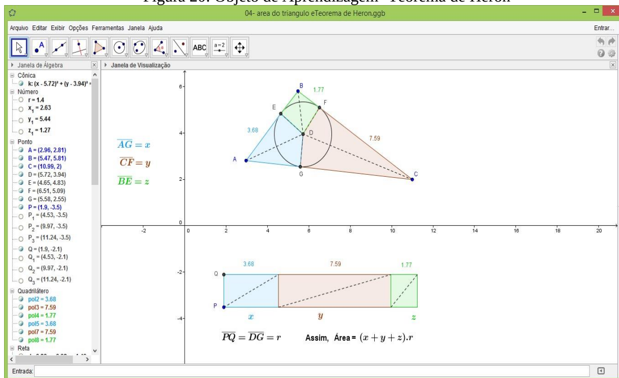
Figura 20: Objeto de Aprendizagem- Teorema de Heron
