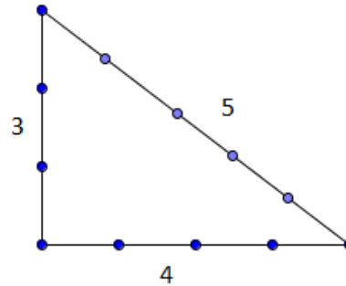
Figura 04- Corda com nós 3, 4 e 5
