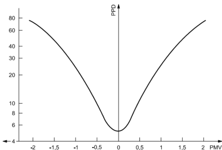
Figura 4 - Relação entre os índices PMV e PPD
