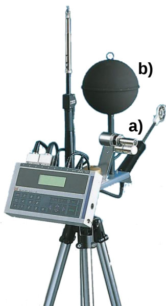
Figura 8 - Estação microclimática BABUC-A. a)psicrômetro; b)termômetro de globo
