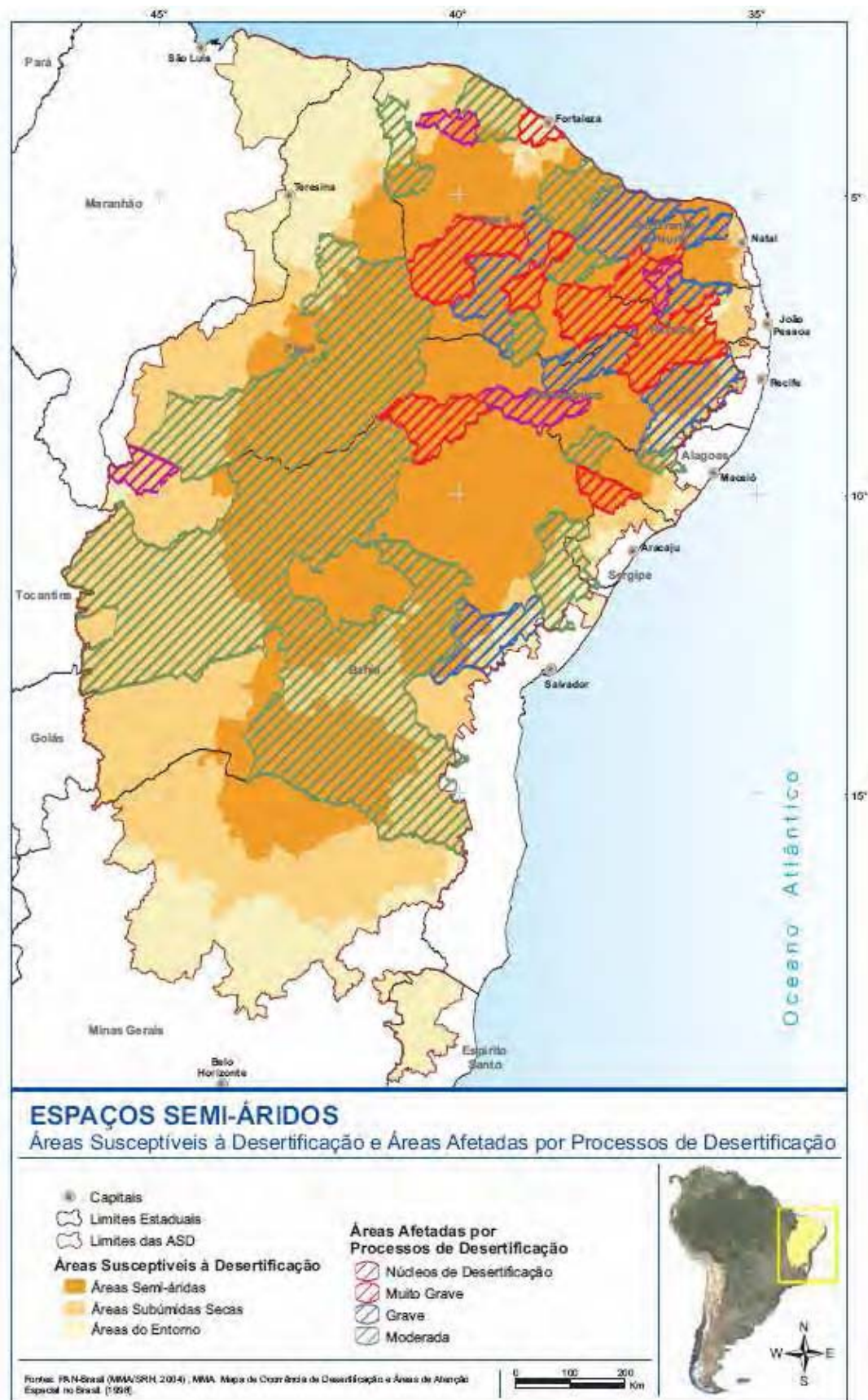
Figura 2 – Áreas Suscetíveis à Desertificação e áreas afetadas por processo de desertificação. Fonte: Ministério da Integração Nacional, 2005.
