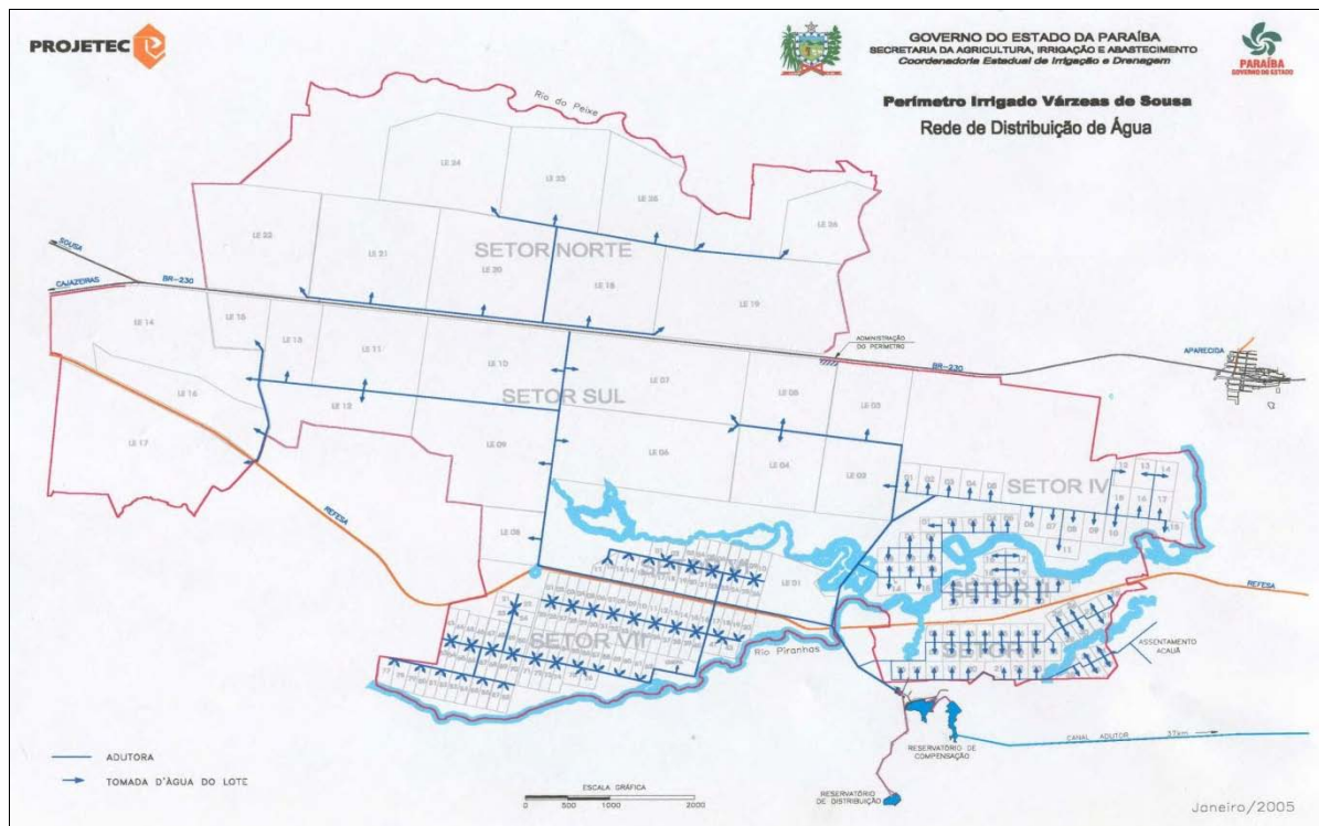
Ilustração 03: Perímetro Irrigado Várzeas de Sousa, Rede de distribuição de água, ano 2005
