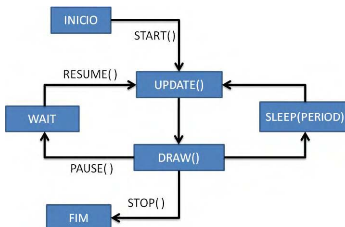
Figura 16 - Comportamento componente Animation. O Ciclo, depois iniciado, fica indeterminadamente fazendo chamadas às funções UPDATE e DRAW com um intervalo de tempo fixo entre a sequência de chamadas. O ciclo pode ser pausado ou parado pelo programa.
