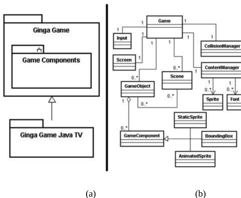
Figura 8 - Diagrama UML do GingaGame. Em (a) Diagrama de Pacotes e em (b) Diagrama de Classes.
