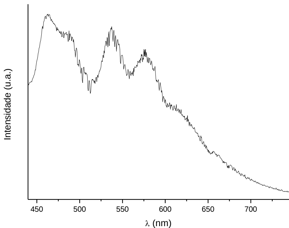
Figura 31 - Espectro de emissão do complexo [\text{Gd}(\text{Py-dk-Ph})_3(\text{H}_2\text{O})] (21), no intervalo de 400 a 720 nm, registrado a 77 K, no estado sólido.
