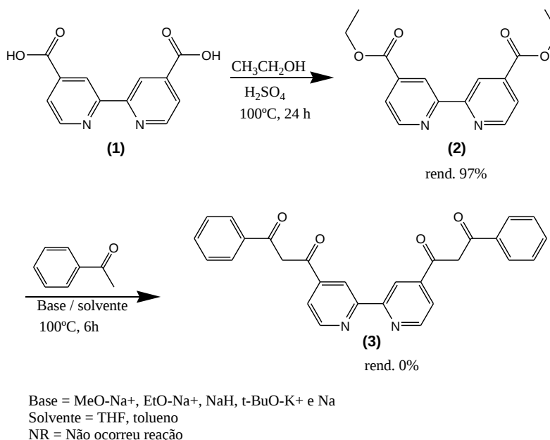
Esquema 10 – Esquema geral para reação de obtenção do composto 3,3'-[4,4'-(2,2'-bipiridil)]bis(1-fenilpropan-1,3-diona) (3)
