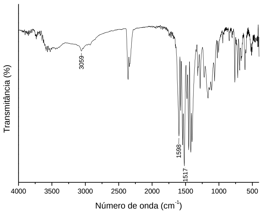
Figura 22 - Espectro de absorção na região do infravermelho do [\text{Gd}(\text{Py-dk-Ph})_3(\text{H}_2\text{O})]
