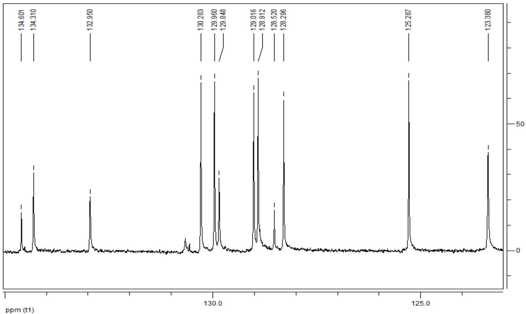
Espectro 33 - Expansão do espectro de RMN ^{13}\text{C} ( \text{CDCl}_3 , 100 MHz) da 1,3-Difenil-2-(4-piridil)-propano-1,3-diona (18) na região de 122 e 135 ppm
