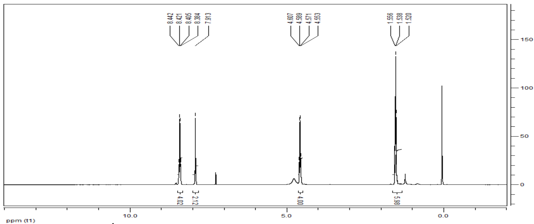
Espectro 12 - Espectro de RMN ^1\text{H} (CDCl 3 , 400 MHz) 1,10-fenantrolina-2,9-dicarboxilato de dietila (8)
