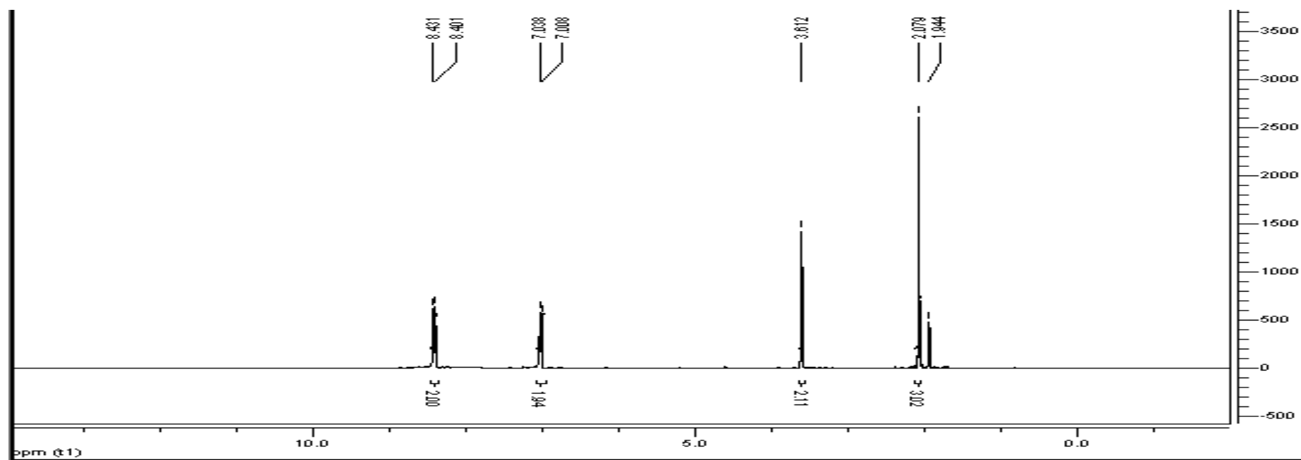
Espectro 23 - Espectro de RMN 1 H (CDCl 3 , 200 MHz) da 1-(4-Piridil)-propano-2-ona (17)
