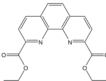
Figura 40 – Estrutura do 1,10-fenantrolina-2,9-dicarboxilato de dietila
