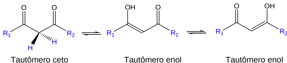
Figura 3 - Tautomerismo ceto-enólico apresentado para as \beta -dicetonas
