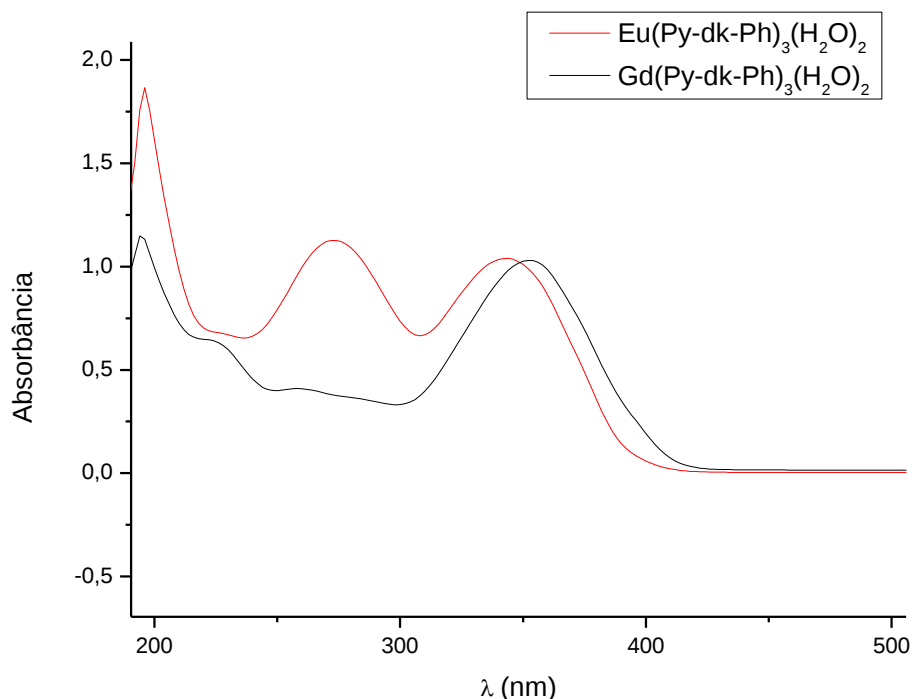
Figura 25 - Espectros de absorção na região do UV-visível dos complexos hidratados do ligante 1-fenil-3-(4-piridil)-propano-1,3-diona (Py-dk-Ph) ( 12 ) contendo os íons \text{Eu}^{3+} ( 20 ) e \text{Gd}^{3+} ( 21 ) em solução etanólica ( 10^{-4} \text{ mol.L}^{-1} ), no intervalo de 190 a 500 nm.
