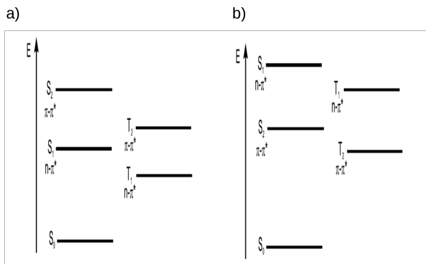
Figura 28 - (a) Diagrama de energia qualitativo do ligante 1-fenil-3-(4-piridil)-propano-1,3-diona (Py-dk-Ph) ( 12 ) neutro. (b) Diagrama de energia qualitativo do ligante 1-fenil-3-(4-piridil)-propano-1,3-diona (Py-dk-Ph) ( 12 ) na forma do sal hidrocloreto ( 14 ) 51 .
