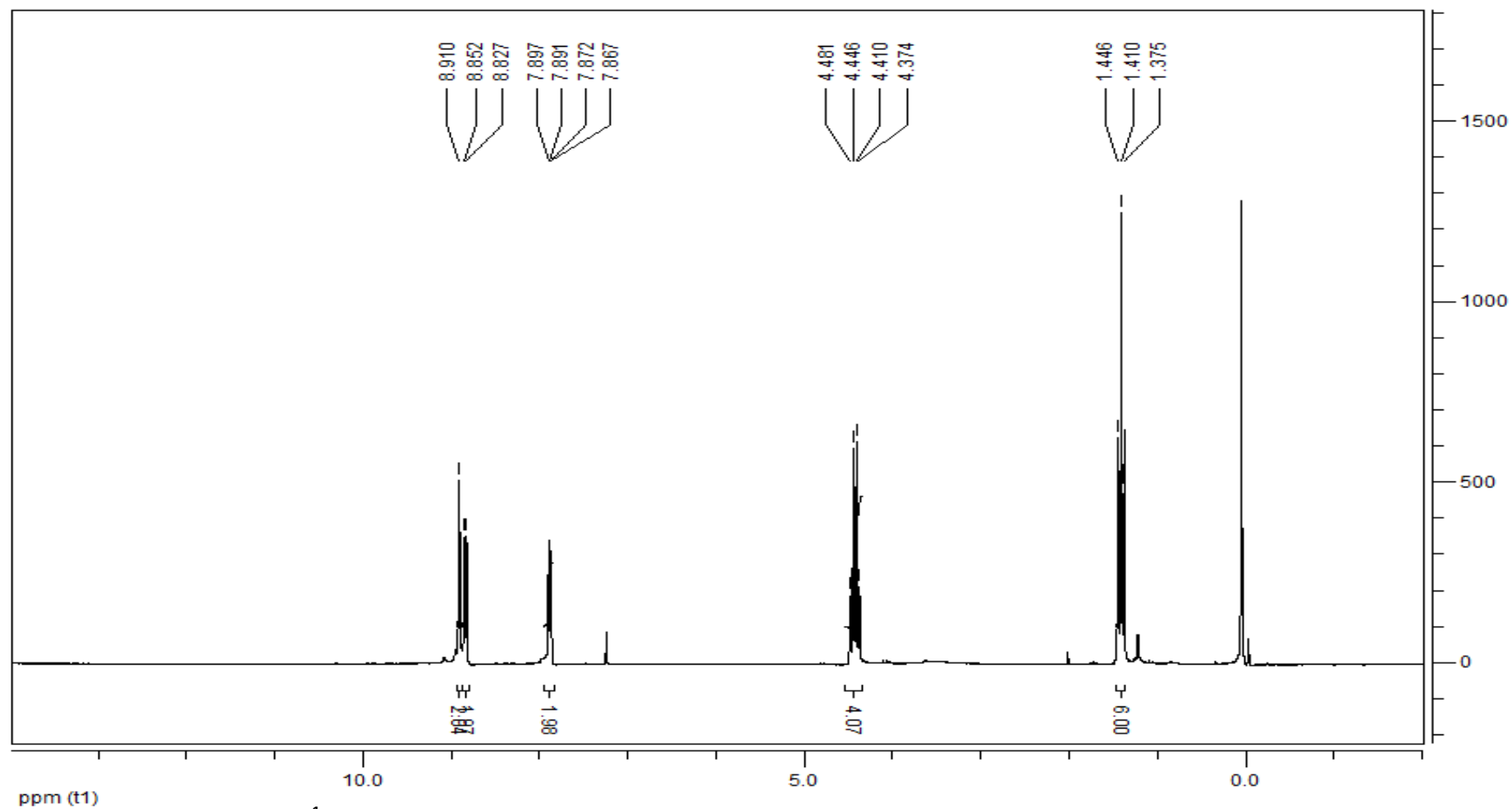
Espectro 1 - Espectro de RMN ^1\text{H} ( \text{CDCl}_3 , 200 MHz) do 2,2'-bipiridina-4,4'-dicarboxilato de dietila (2)
