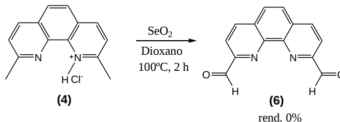
Esquema 12 - Síntese da 2,9-dicarbonil-1,10-fenantrolina
