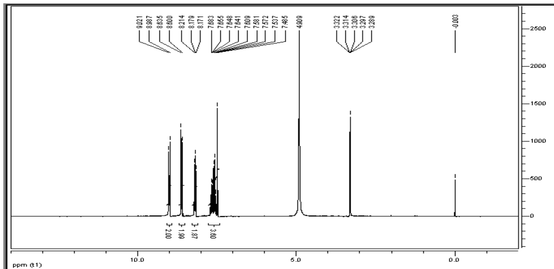
Espectro 20 - Espectro de RMN ^1\text{H} (MeOD, 200 MHz) do sólido obtido da fase aquosa (13) da reação de obtenção da 1-fenil-3-(4-piridil)-propano-1,3 diona (Py-dk-Ph) (12) após adição de \text{NaHCO}_3
