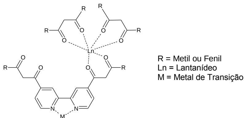
Figura 11 – Representação de complexo heterobimetálico do íon lantanídeo e metal de transição
