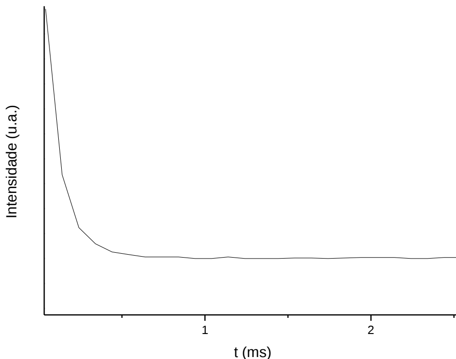
Figura 35 - Curva de decaimento de luminescência dos níveis emissores para o complexo [\text{Eu}(\text{Py-dk-Ph})_3(\text{H}_2\text{O})] (20), registrado a 298 K, no estado sólido.
