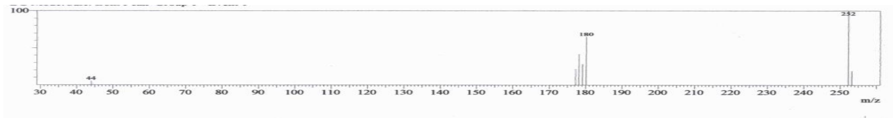
Espectro 11 – Espectro de massa 1,10-fenantrolina-2,9-dicarboxilato de dietila (8)
