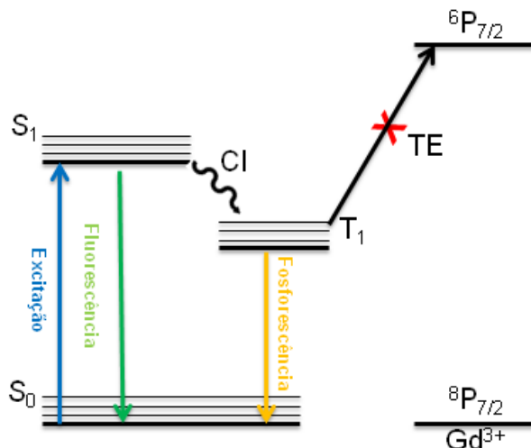
Figura 29 – Diferença dos níveis de energia dos ligantes orgânicos e do íon Gd^{3+} . CI: conversão interna e TE: Transferência de energia.
