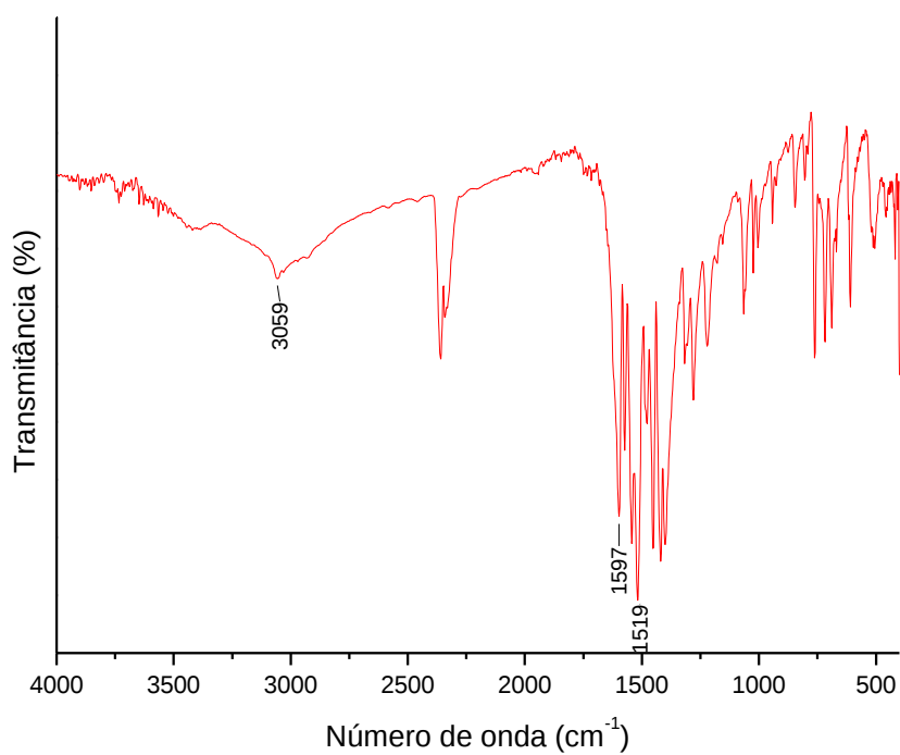
Figura 21- Espectro de absorção na região do infravermelho do [\text{Eu}(\text{Py-dk-Ph})_3(\text{H}_2\text{O})]
