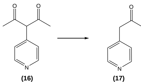
Esquema 16 - Síntese da 1-(4-Piridil)-propano-2-ona (17)
