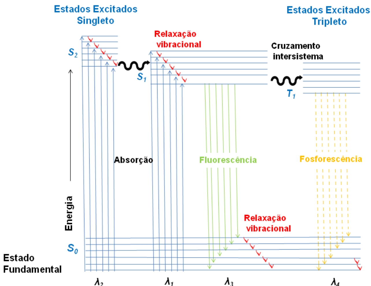
Figura 1 - Diagrama de Jablonski para o sistema de níveis de energia sendo S_0 estado singlete fundamental, S_1 e S_2 estados singletos excitados, T_1 estado tripleto
