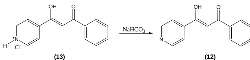
Esquema 14- Esquema exemplificando a obtenção da 1-fenil-3-(4-piridil)-propano-1,3-diona (12) a partir do respectivo hidrocloreto (13)
