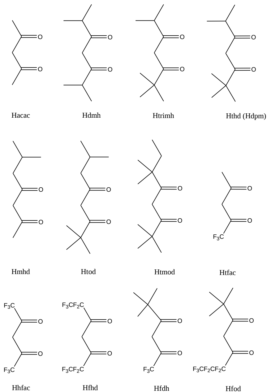
Figura 4 - Estruturas de \beta -dicetonas com substituintes alifáticos 26 .
