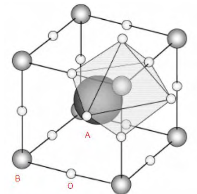
Figura 1 - Estrutura cristalina da perovskita cúbica ABO_3 (SILVA et al. , 2007).
