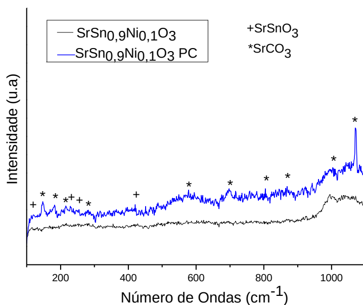
Figura 15 – Espectros Raman do sistema \text{SrSn}_{0.9}\text{Ni}_{0.1}\text{O}_3 antes e após a reação de redução do NO com CO.
