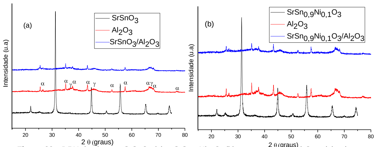
Figura 29 - DRX do sistema \text{SrSnO}_3 (a) e \text{SrSn}_{0,9}\text{Ni}_{0,1}\text{O}_3 (b) suportados em \text{Al}_2\text{O}_3 calcinados a 800°C.
