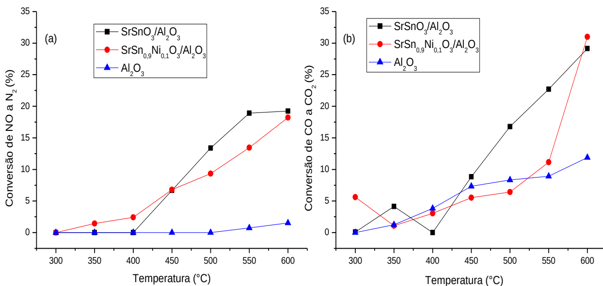
Figura 48 - Conversão de NO a N 2 (a) e de CO a CO 2 (b) dos catalisadores puro e dopado com níquel suportado em Al 2 O 3 .
