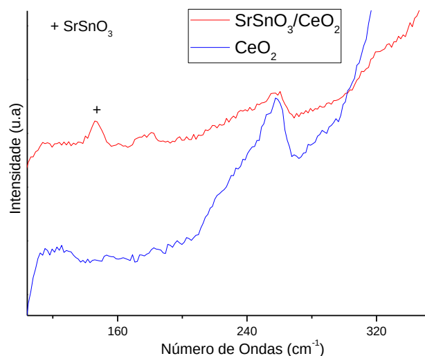
Figura 37 – Espectros Raman do sistema \text{SrSnO}_3/\text{CeO}_2 e do \text{CeO}_2 ampliado entre 105 e 345\text{ cm}^{-1} .
