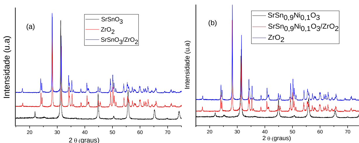
Figura 42 - DRX do sistema \text{SrSnO}_3 (a) e \text{SrSn}_{0,9}\text{Ni}_{0,1}\text{O}_3 (b) suportados em \text{ZrO}_2 calcinados a 800^\circ\text{C} .
