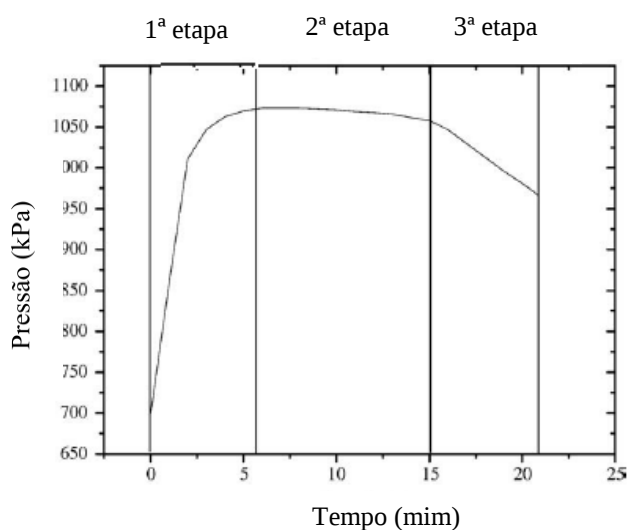
Figura 9. Representação esquemática da variação de pressão do teste oxidativo petroOXY. (ARAÚJO et al. , 2009). 1ª etapa de 0 a 5 minutos; 2ª etapa de 5 a 15 minutos; 3ª de 5 a 20 minutos.
