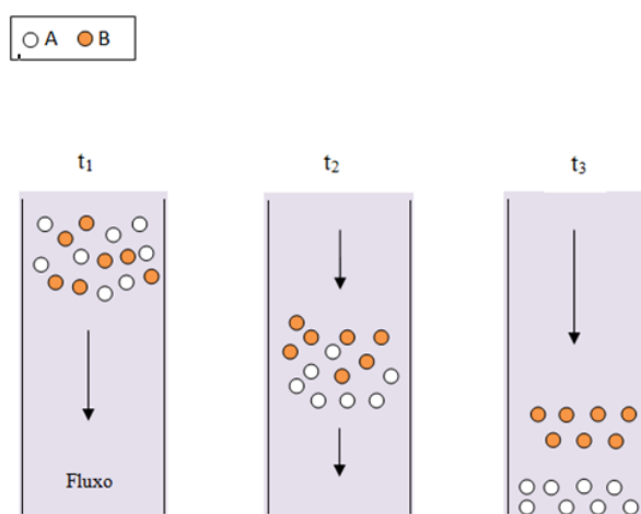
Figura 10. Representação esquemática do processo de separação de dois compostos, denominados A e B, em uma coluna cromatográfica. (adaptado de LANÇAS, 2009).
