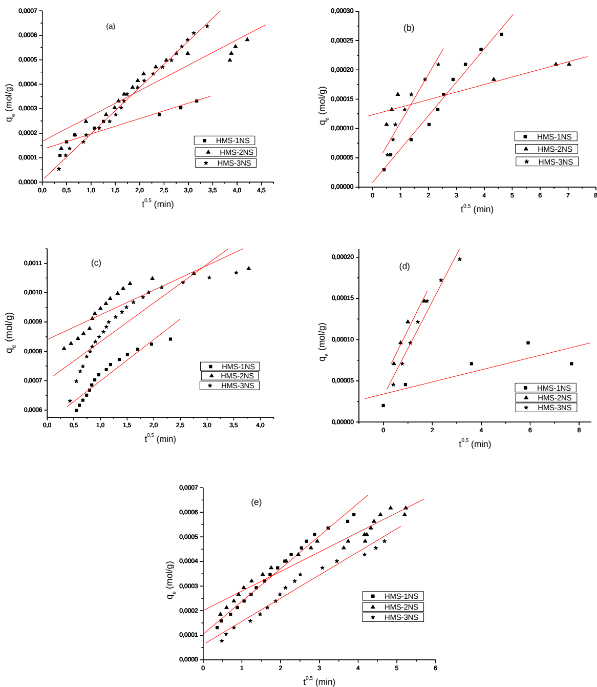
Figura 5.45 – Cinética de difusão intrapartícula para adsorção a 25°C dos cátions \text{Cd}^{2+} (a), \text{Co}^{2+} (b), \text{Cu}^{2+} (c), \text{Ni}^{2+} (d) e \text{Pb}^{2+} (e) nas matrizes funcionalizadas com ácido tioglicólico.
