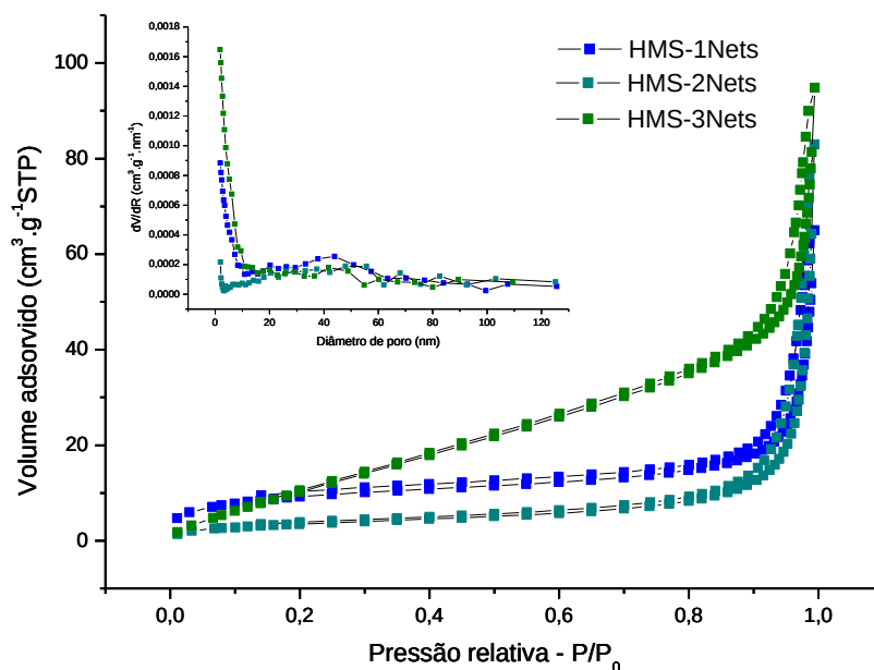
Figura 5.33 - Isotermas de adsorção de \text{N}_2 das amostras das matrizes HMS funcionalizadas com etilenossulfeto. Em destaque as curvas de distribuições de diâmetro de poro segundo o método BJH.
