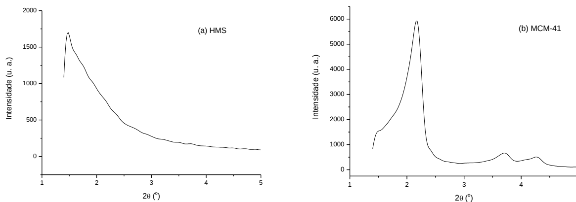
Figura 5.3 – Difratomogramas de raios-X das amostras das matrizes precursoras de sílica HMS (a) e MCM-41 (b).
