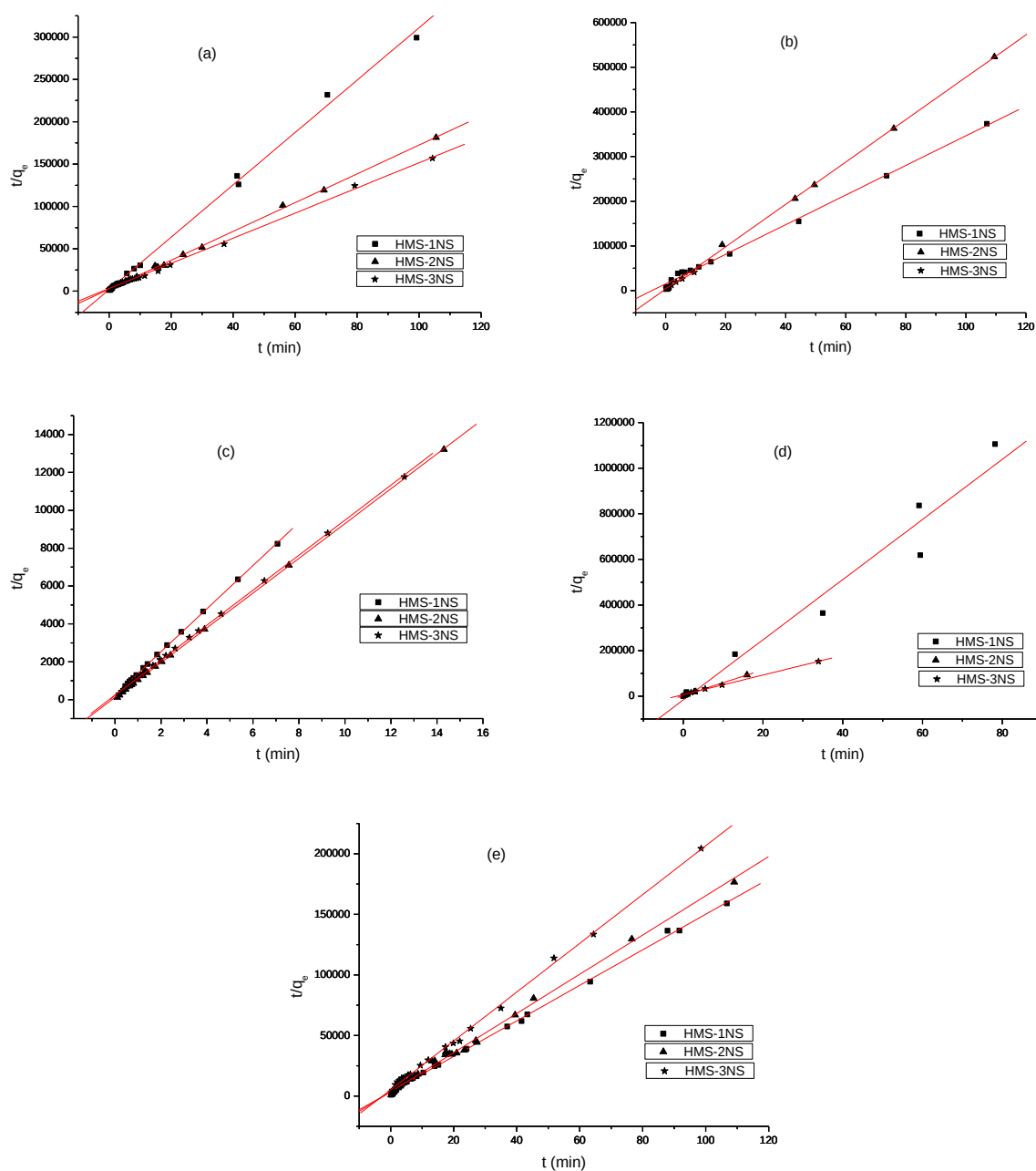
Figura 5.43 – Cinética de pseudo-segunda ordem para adsorção a 25°C dos cátions Cd 2+ (a), Co 2+ (b), Cu 2+ (c), Ni 2+ (d) e Pb 2+ (e) nas matrizes funcionalizadas com ácido tioglicólico.
