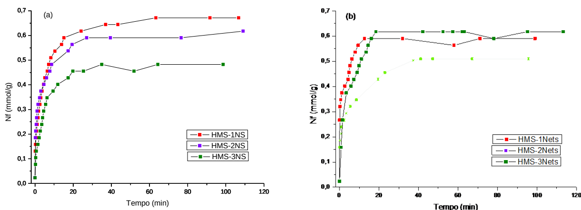
Figura 5.40 - Isotermas de tempo para retenção de \text{Pb}^{2+} na concentração de 10^{-2} mol/L a 25^\circ\text{C} nas matrizes HMS funcionalizadas com ácido tioglicólico (a) ou etilenossulfeto (b).
