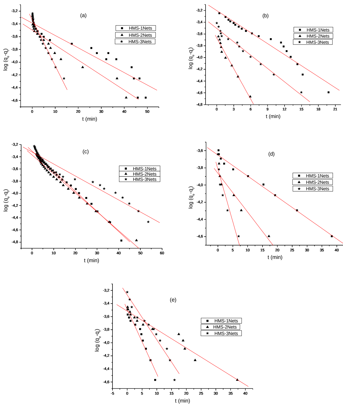
Figura 5.42 – Cinética de pseudo-primeira ordem para adsorção a 25°C dos cátions Cd 2+ (a), Co 2+ (b), Cu 2+ (c), Ni 2+ (d) e Pb 2+ (e) nas matrizes funcionalizadas com etilenossulfeto.
