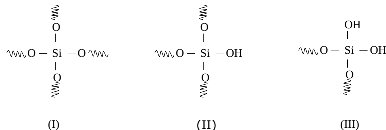
Figura 5.8 – Esquema das estruturas das espécies \text{Q}^4 (I), \text{Q}^3 (II) e \text{Q}^2 (III).
