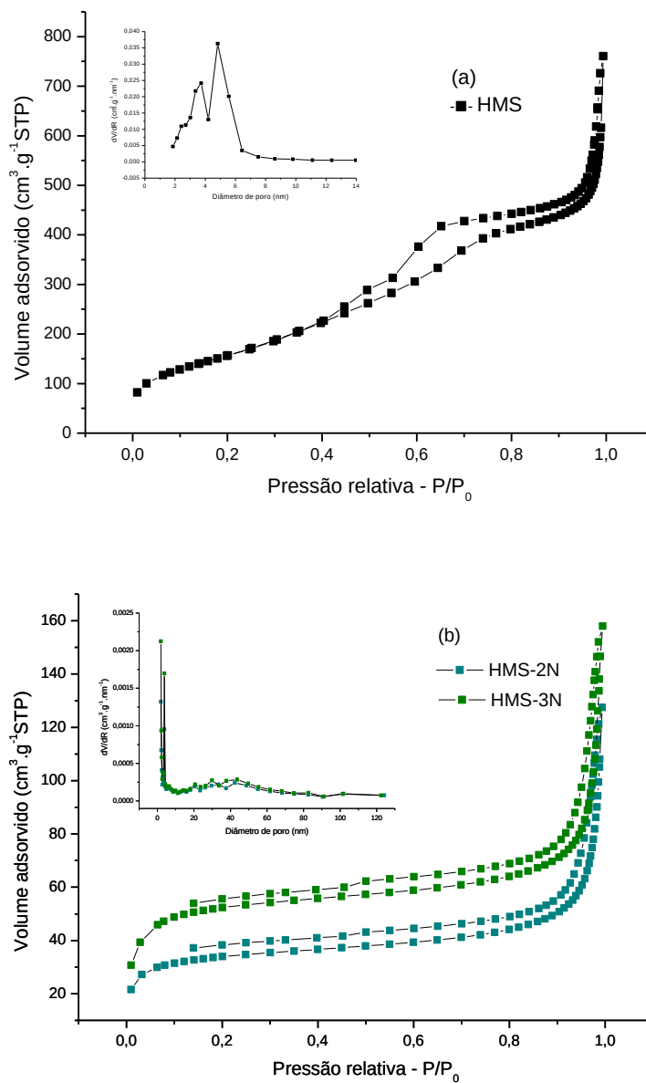
Figura 5.31 - Isotermas de adsorção-dessorção de nitrogênio das amostras das matrizes HMS: pura (a) e modificadas (b). Em destaque as curvas de distribuições de diâmetro de poro segundo o método BJH.
