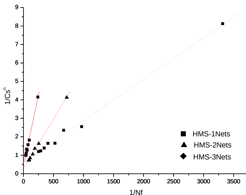
Figura 5.52 – Formas linearizadas das isothermas de concentração do cobre a 25°C segundo o modelo de Langmuir-Freundlich para as matrizes HMS funcionalizadas com etilenossulfeto.
