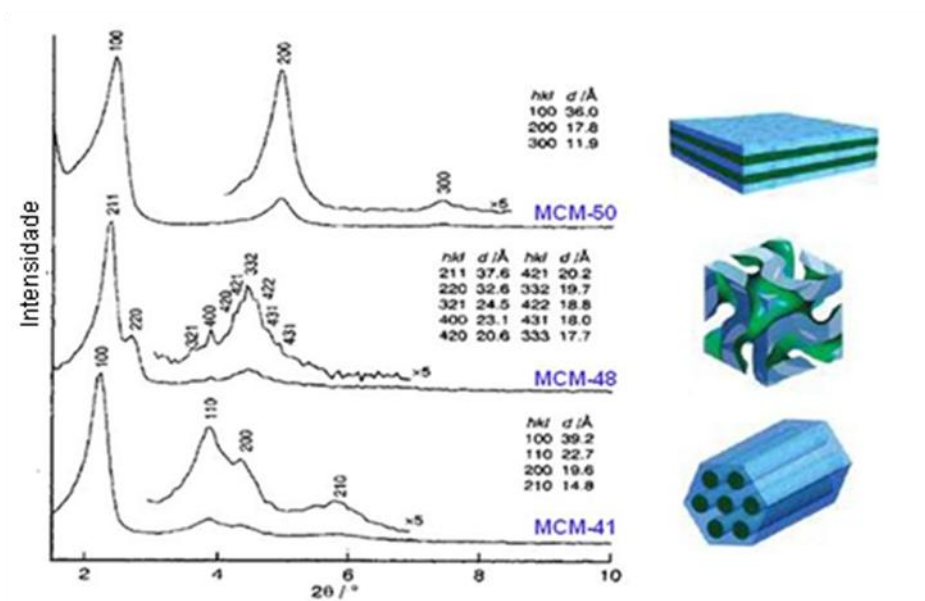
Figura 2.3 - Padrões de DRX das fases MCM-41 (hexagonal), MCM-48 (cúbica), e MCM-50 (lamelar). Adaptado de CORMA, 1997.
