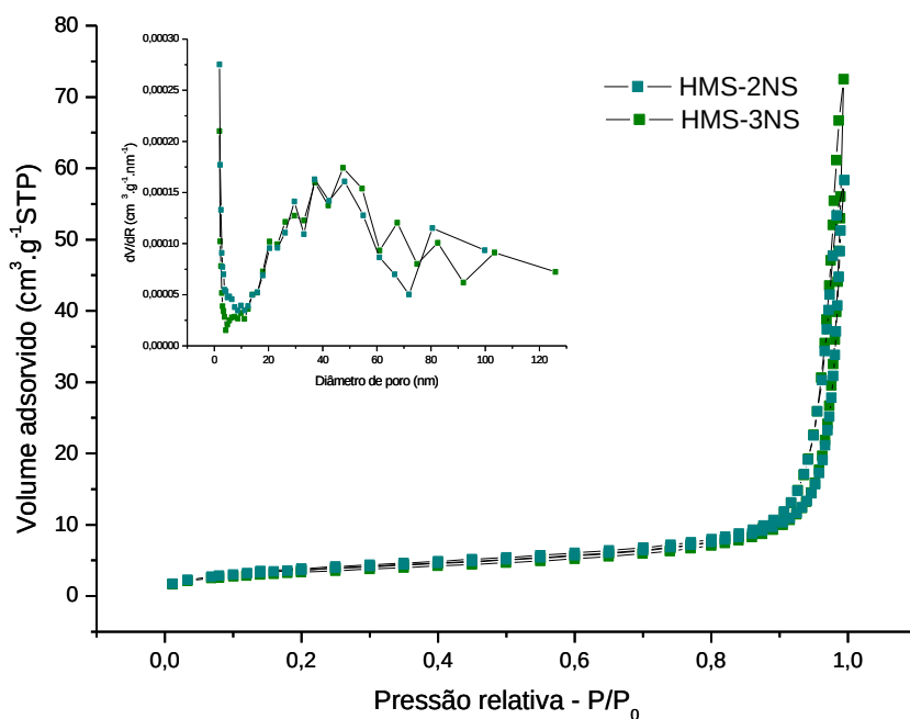
Figura 5.32 - Isotermas de adsorção-dessorção de nitrogênio das amostras das matrizes HMS funcionalizadas com ácido tioglicólico. Em destaque as curvas de distribuições de diâmetro de poro segundo o método BJH.
