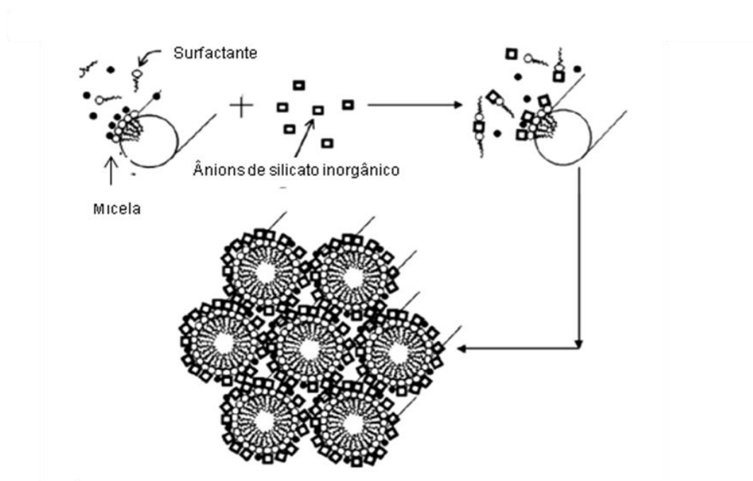
Figura 2.8 – Detalhamento da síntese de sílica mesoporosa a partir do mecanismo de reunião cooperativa. Adaptado de CHEW et al., 2010.
