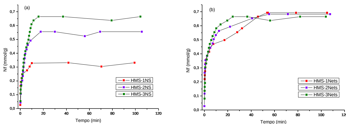
Figura 5.36 - Isotermas de tempo para retenção de \text{Cd}^{2+} na concentração de 10^{-2} mol/L a 25°C nas matrizes HMS funcionalizadas com (a) ácido tioglicólico e (b) etilenossulfeto.
