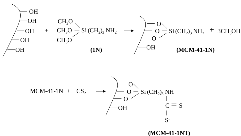
Figura 5.17 - Esquema de reação de modificação da sílica MCM-41 com aminopropil e reação subsequente com dissulfeto de carbono.
