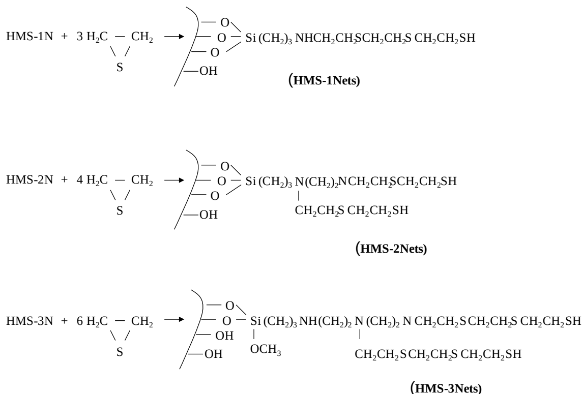
Figura 5.16 - Esquema de reação de funcionalização da sílica HMS-xN (x=1, 2 ou 3) com etilenossulfeto.
