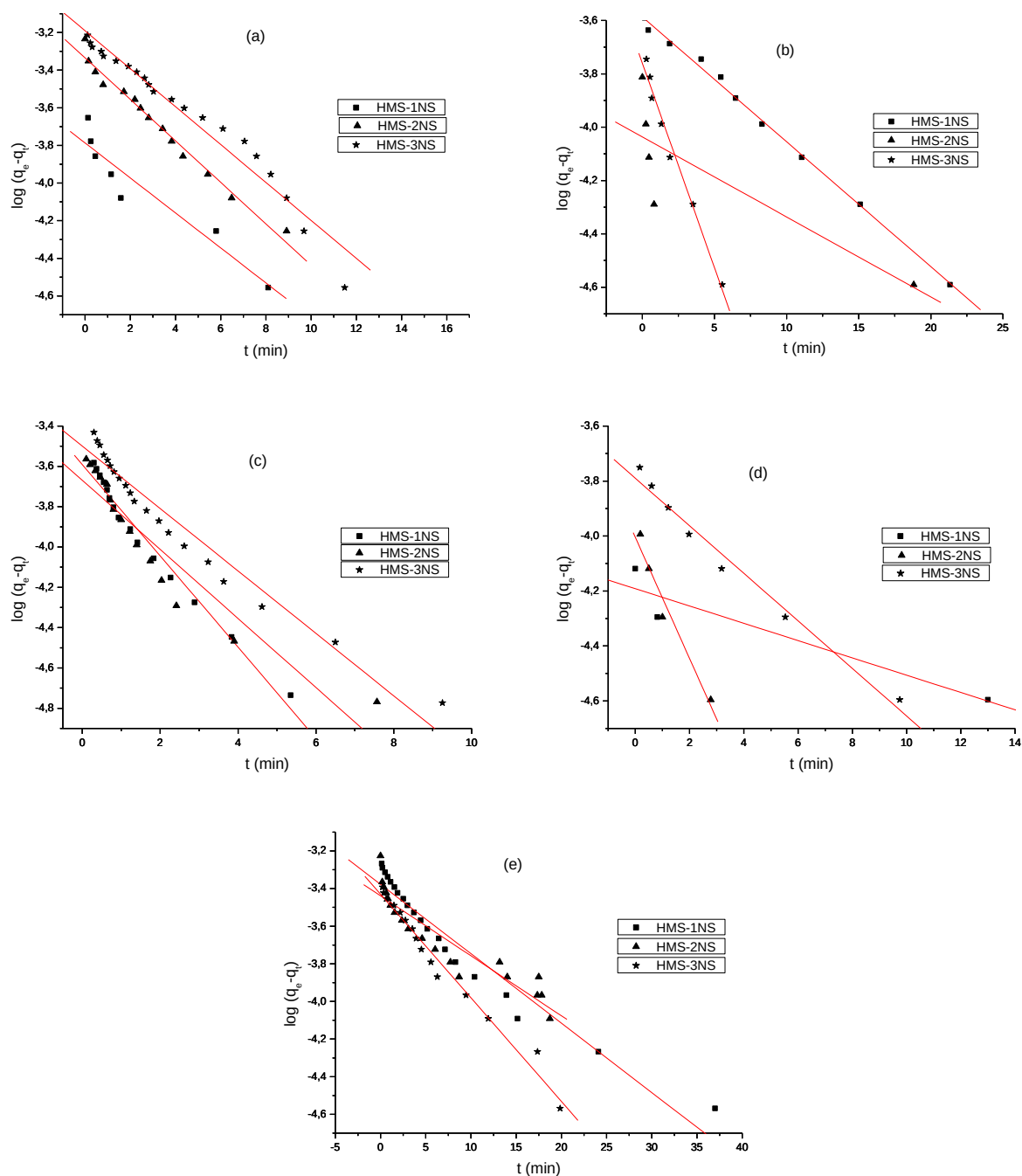
Figura 5.41 – Cinética de pseudo-primeira ordem para adsorção a 25°C dos cátions Cd 2+ (a), Co 2+ (b), Cu 2+ (c), Ni 2+ (d) e Pb 2+ (e) nas matrizes funcionalizadas com ácido tioglicólico.
