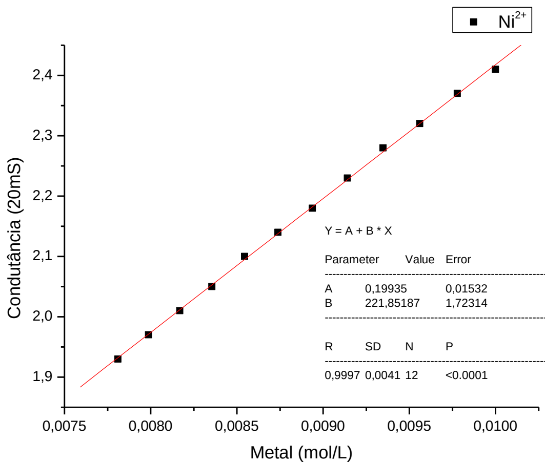
Figura - Curva de calibração para cátion metálico \text{Ni}^{2+} .
