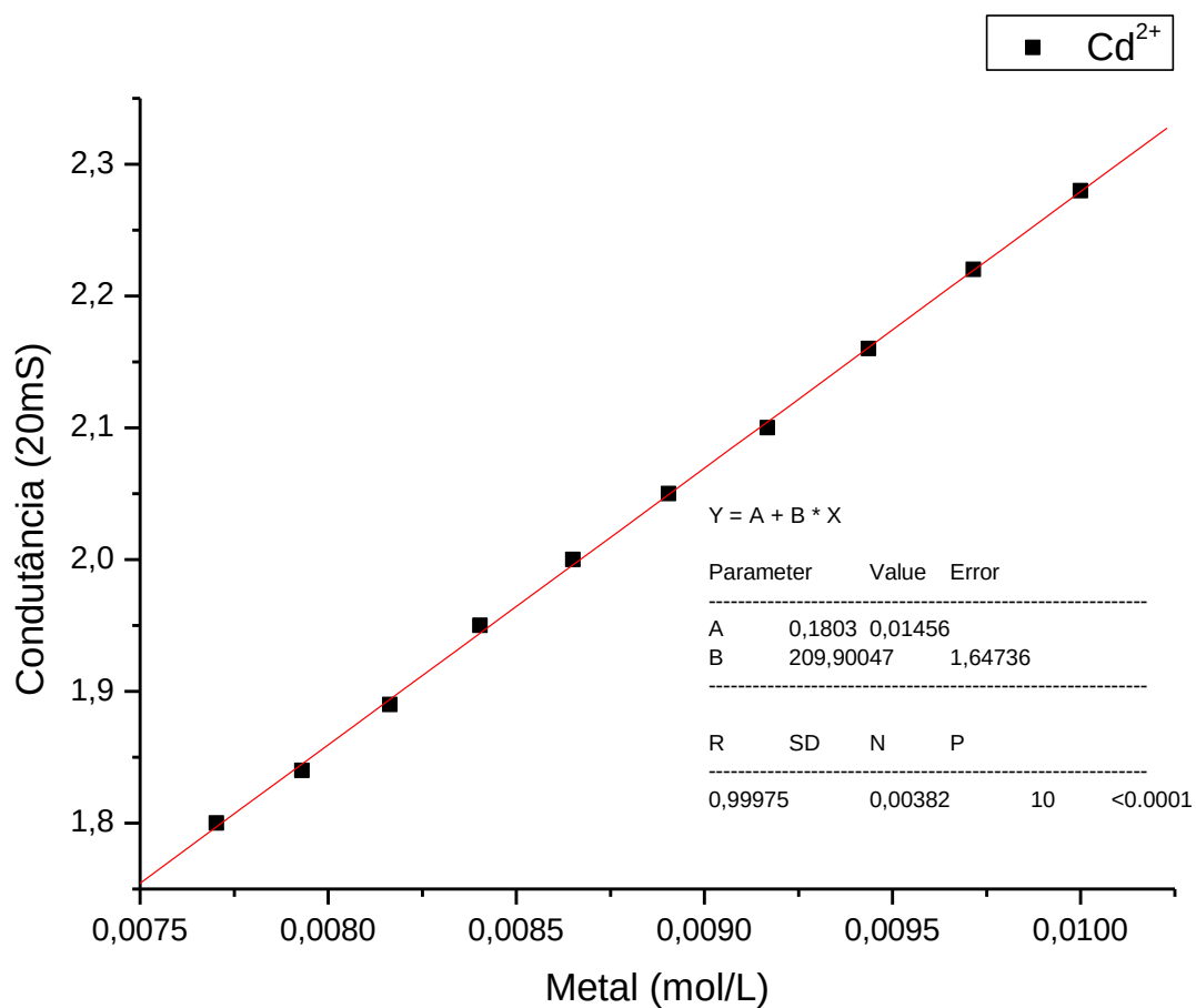
Figura - Curva de calibração para cátion metálico \text{Cd}^{2+} .
