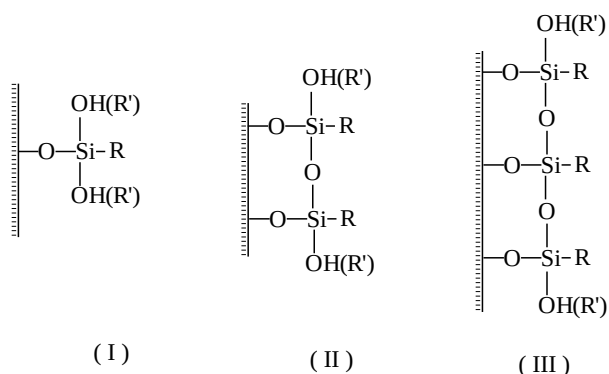
Figura 5.9 – Esquemas das estruturas das espécies químicas do T: \text{T}^1 (I), \text{T}^2 (II) e \text{T}^3 (III).
