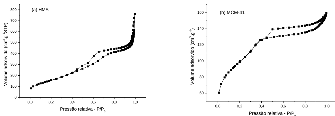
Figura 5.6 – Isotermas de adsorção de N 2 das matrizes HMS (a) e MCM-41(b).
