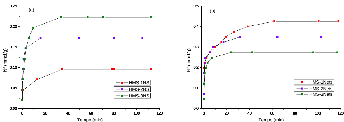
Figura 5.39 - Isotermas de tempo para retenção de \text{Ni}^{2+} na concentração de 10^{-2} mol/L a 25^\circ\text{C} nas matrizes HMS funcionalizadas com ácido tioglicólico (a) ou etilenossulfeto (b).
