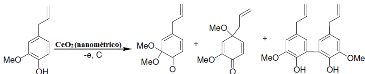
Figura 63 - Ilustração esquemática da oxidação do eugenol pela a ação de nanoestruturas de óxido de cério (IV) (adaptado de COSTA, 2000).
