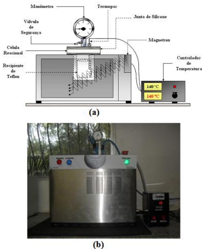
Figura 14 Representação esquemática (a) e Fotos (b) Reator de Micro-ondas industrial(VOLANTE et al,2008).
