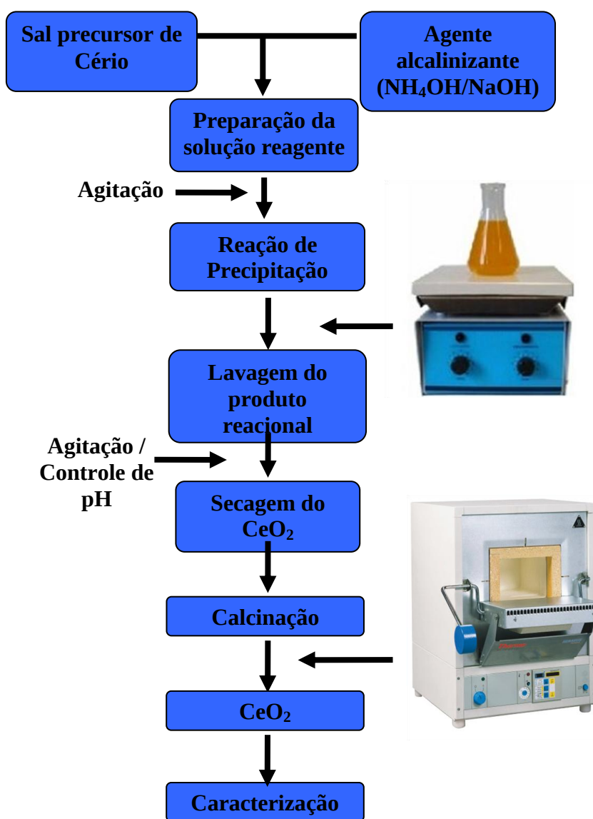
Figura 12 - Processo de obtenção de nanopartículas de CeO 2 pelo método de precipitação.
