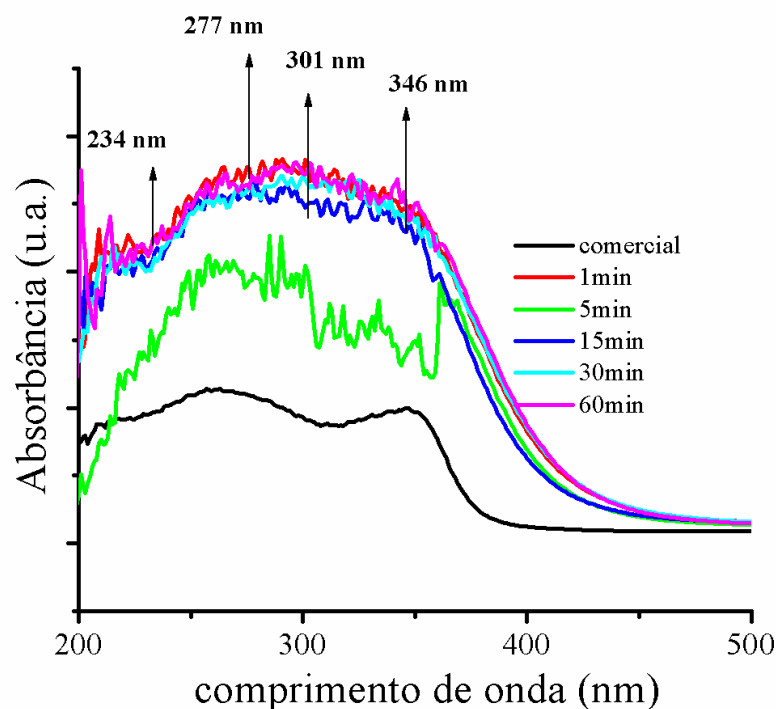
Figura 47 - Espectros na região do UV-visível, do sistema \text{CeO}_2 , na seguinte rota de síntese: \text{CeO}_2\text{-NH}_4\text{OH-PEG-150}^\circ\text{C} .
