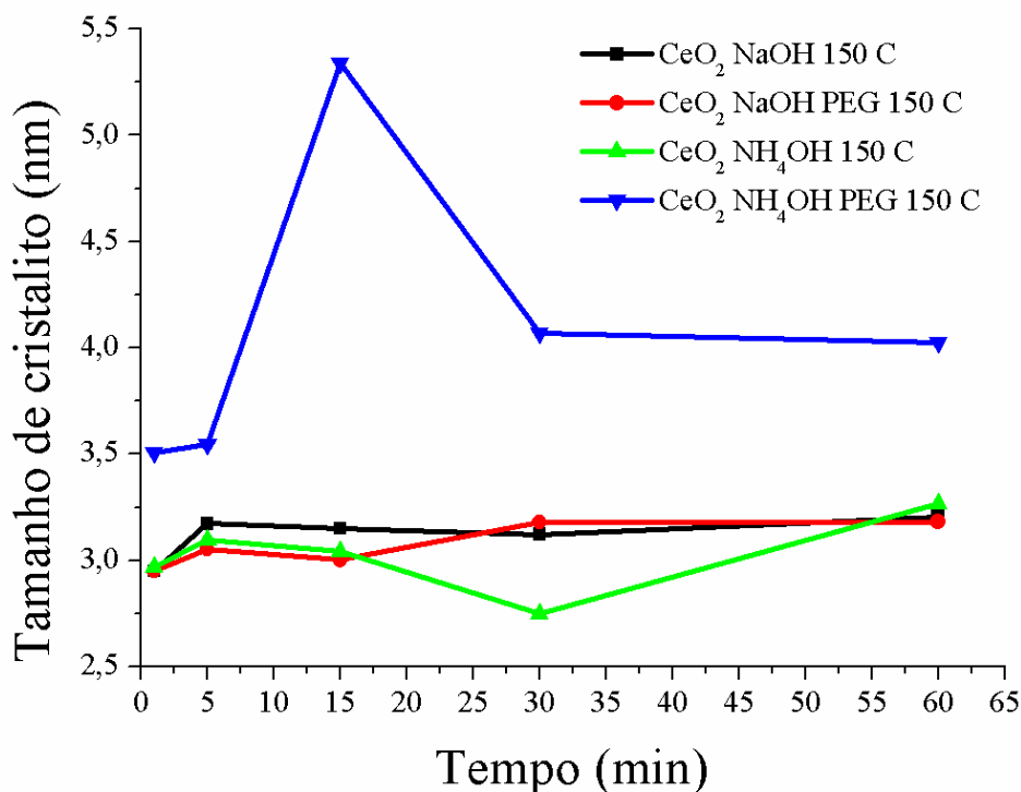
Figura 33 - Tamanho de cristalito para os sistema de \text{CeO}_2 nas seguintes rotas de síntese: \text{CeO}_2\text{-NaOH-150}^\circ\text{C} ; \text{CeO}_2\text{-NaOH-PEG-150}^\circ\text{C} ; \text{CeO}_2\text{-NH}_4\text{OH-150}^\circ\text{C} e \text{CeO}_2\text{-NH}_4\text{OH-PEG-150}^\circ\text{C} .
