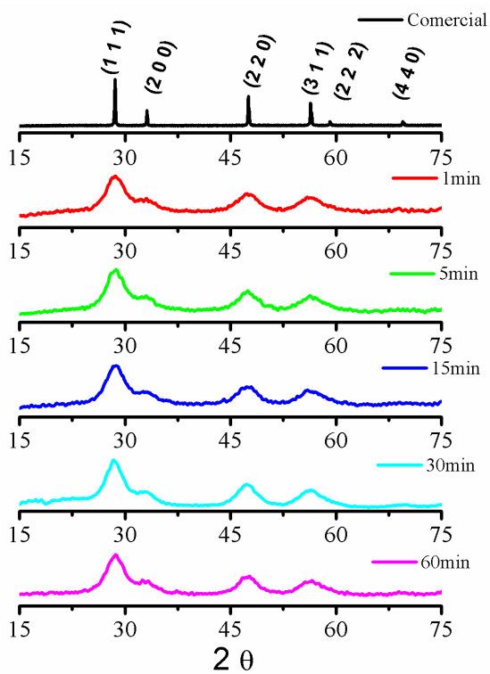
Figura 28 - Difratomogramas de raios-X do sistema \text{CeO}_2 na seguinte rota de síntese: \text{CeO}_2 -NaOH-PEG-150°C.
