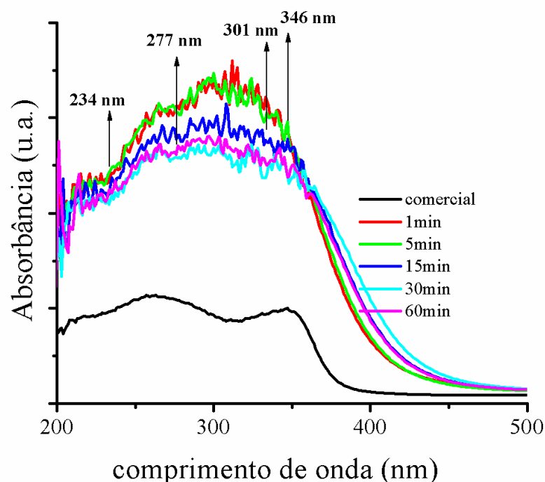
Figura 44 - Espectros na região do UV-visível, do sistema \text{CeO}_2 , na seguinte rota de síntese: \text{CeO}_2\text{-NaOH-}150^\circ\text{C} .
