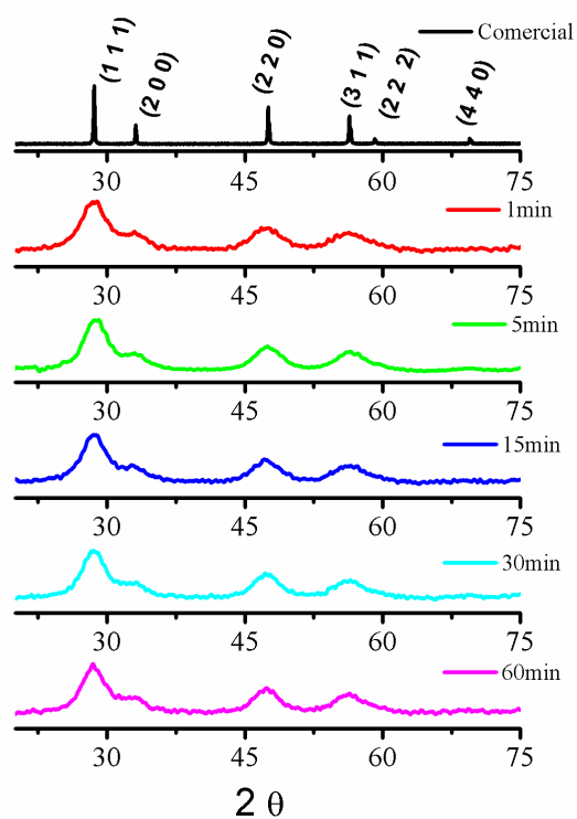
Figura 27 - Difratomogramas de raios-X do sistema \text{CeO}_2 na seguinte rota de síntese: \text{CeO}_2 -NaOH-150°C.
