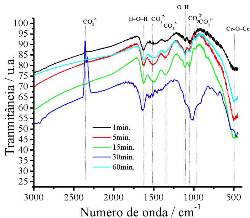
Figura 37 - Espectros de absorção na região do infravermelho do óxido de cério (IV) para o sistema:CeO 2 -NH 4 OH-150°C.
