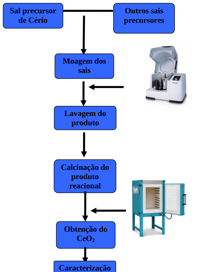
Figura 8 - Processo de obtenção de nanopartículas de \text{CeO}_2 a partir do método de síntese mecânica.
