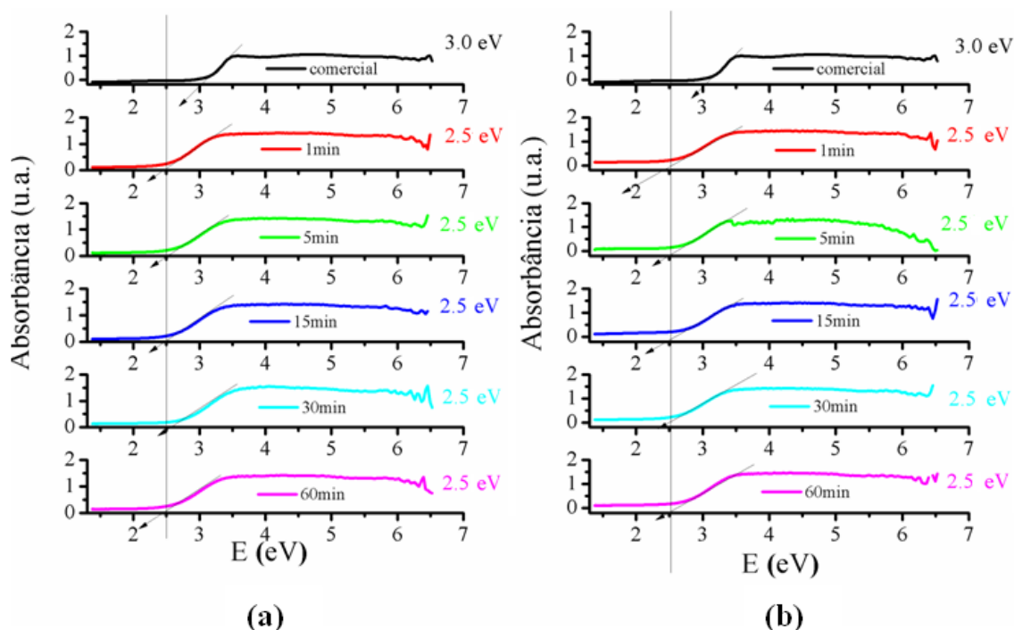
Figura 49 - Espectros na região do UV-visível (valor do gap), do sistema \text{CeO}_2 nas seguintes rotas de síntese: (a) \text{CeO}_2\text{-NH}_4\text{OH-150}^\circ\text{C} e (b) \text{CeO}_2\text{-NH}_4\text{OH-PEG-150}^\circ\text{C} .
