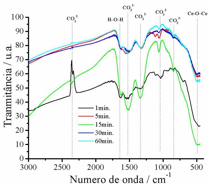
Figura 36 - Espectros de absorção na região do infravermelho do óxido de cério (IV) para o sistema:CeO 2 -NaOH-PEG-150°C.
