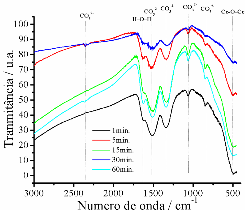
Figura 35 - Espectros de absorção na região do infravermelho do óxido de cério (IV): \text{CeO}_2 -NaOH-150°C.
