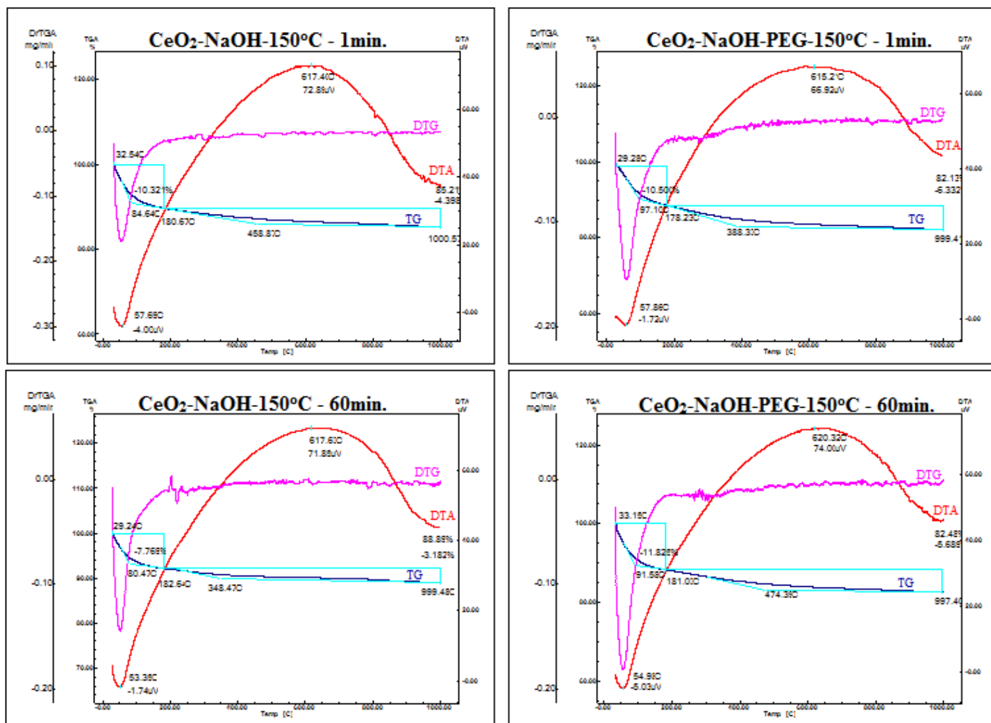
Figura 34 – Curvas de termogravimetria (TG), termogravimetria derivada (DTG) e de análise térmica diferencial (DTA) do sistema CeO 2 nas seguintes rotas de síntese: CeO 2 -NaOH-150°C; CeO 2 -NaOH-PEG-150°C.
