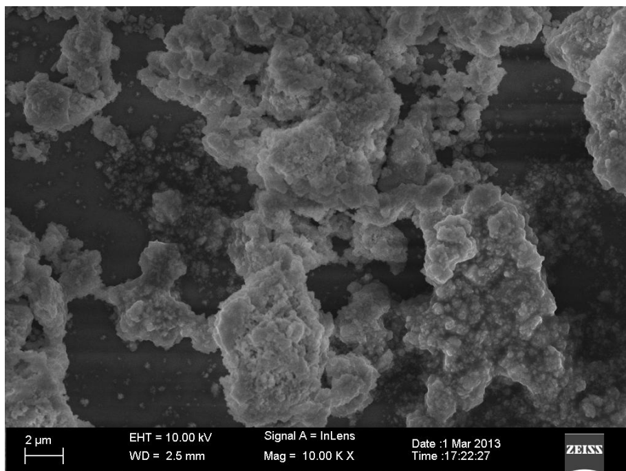
Figura 50 - Microscopia eletrônica de varredura do sistema CeO 2 na seguinte rota de síntese: CeO 2 -NaOH-150°C.
