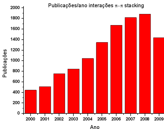
FIGURA 1.9: Número de publicações/ano envolvendo estudos sobre as interações \pi - \pi stacking , baseado em busca informatizada com o programa SciFinder™ Scholar 2007 (palavras-chave: " \pi - \pi stacking interactions").
