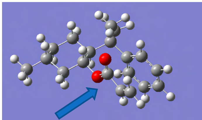
Figura 1.6: Reação de Diels-Alder estereosseletiva, ocorrendo na face pró-quiral re (em seta azul) do acrilato de 8-fenilmentila.
