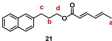
Figura 4.5: Determinação estrutural de 21 .
