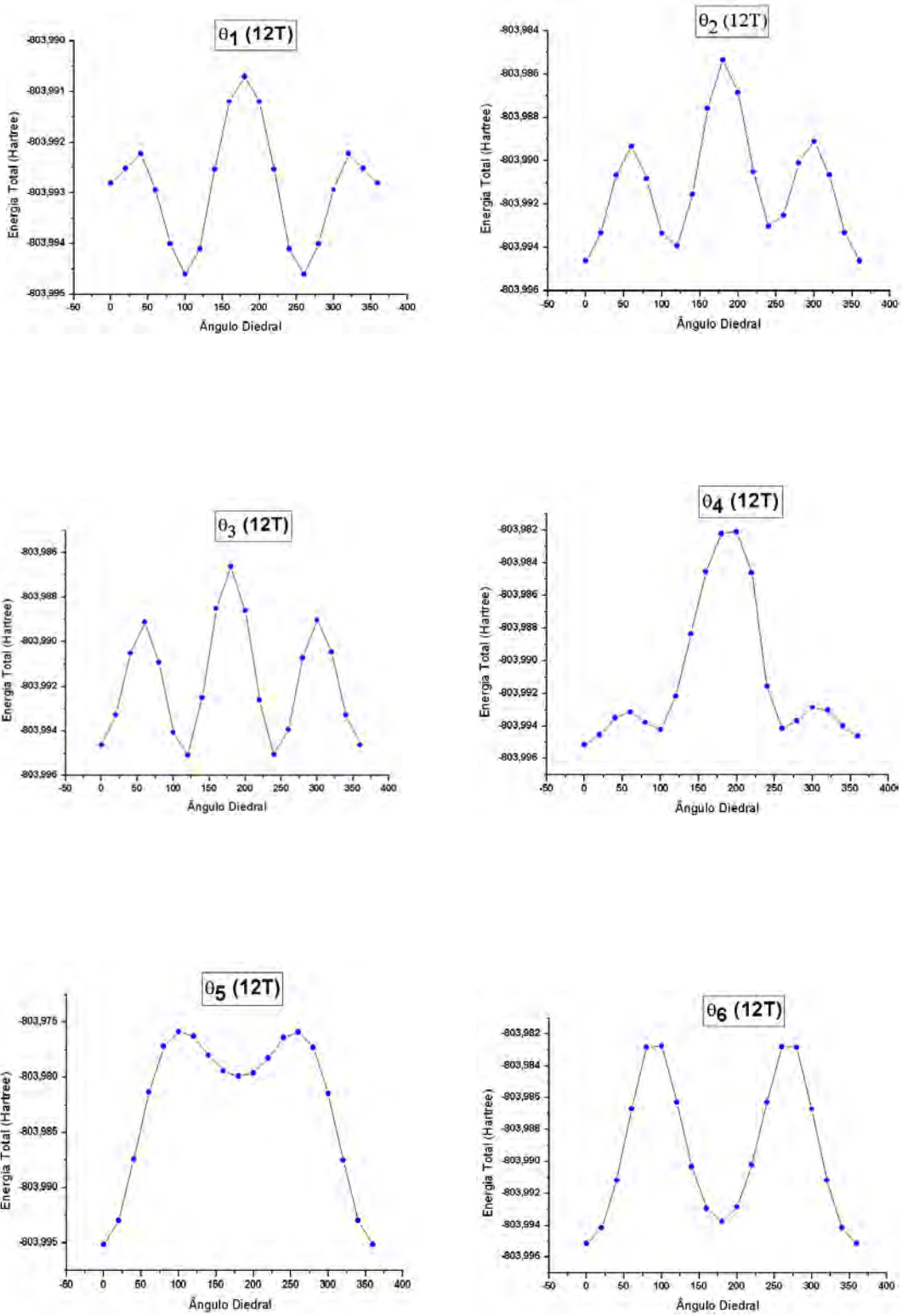
Figura 4.10: Curvas de energia potencial para a conformação 12T calculado com o método HF/6-31G(d).
