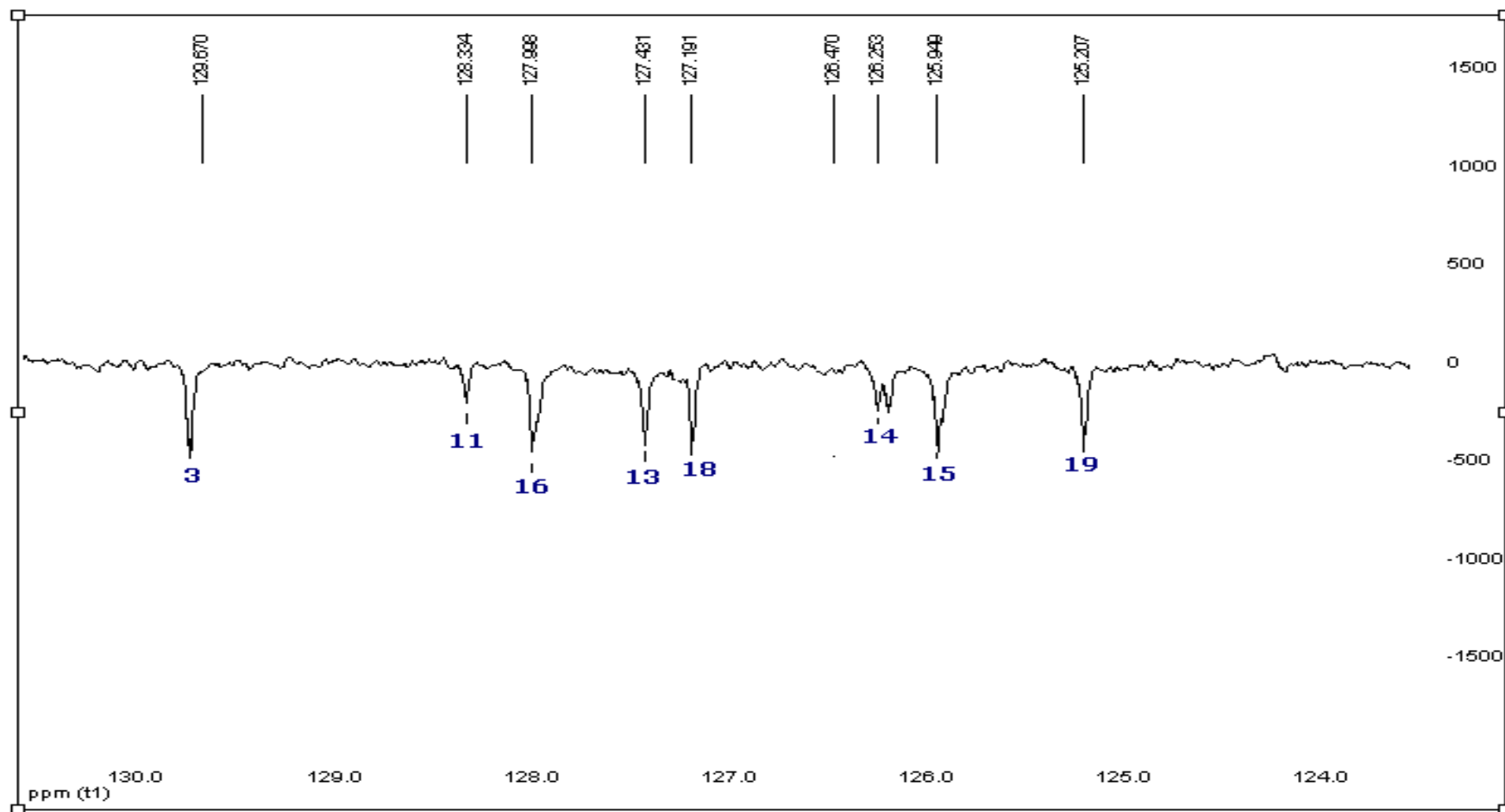
Espectro 8.12: Expansão do Espectro RMN ^{13}\text{C} - APT de sorbato de 3- Naftilpropila ( 21 ) na região de 129,6 a 125,2 ppm (CDCl _3 , 50 MHz).
