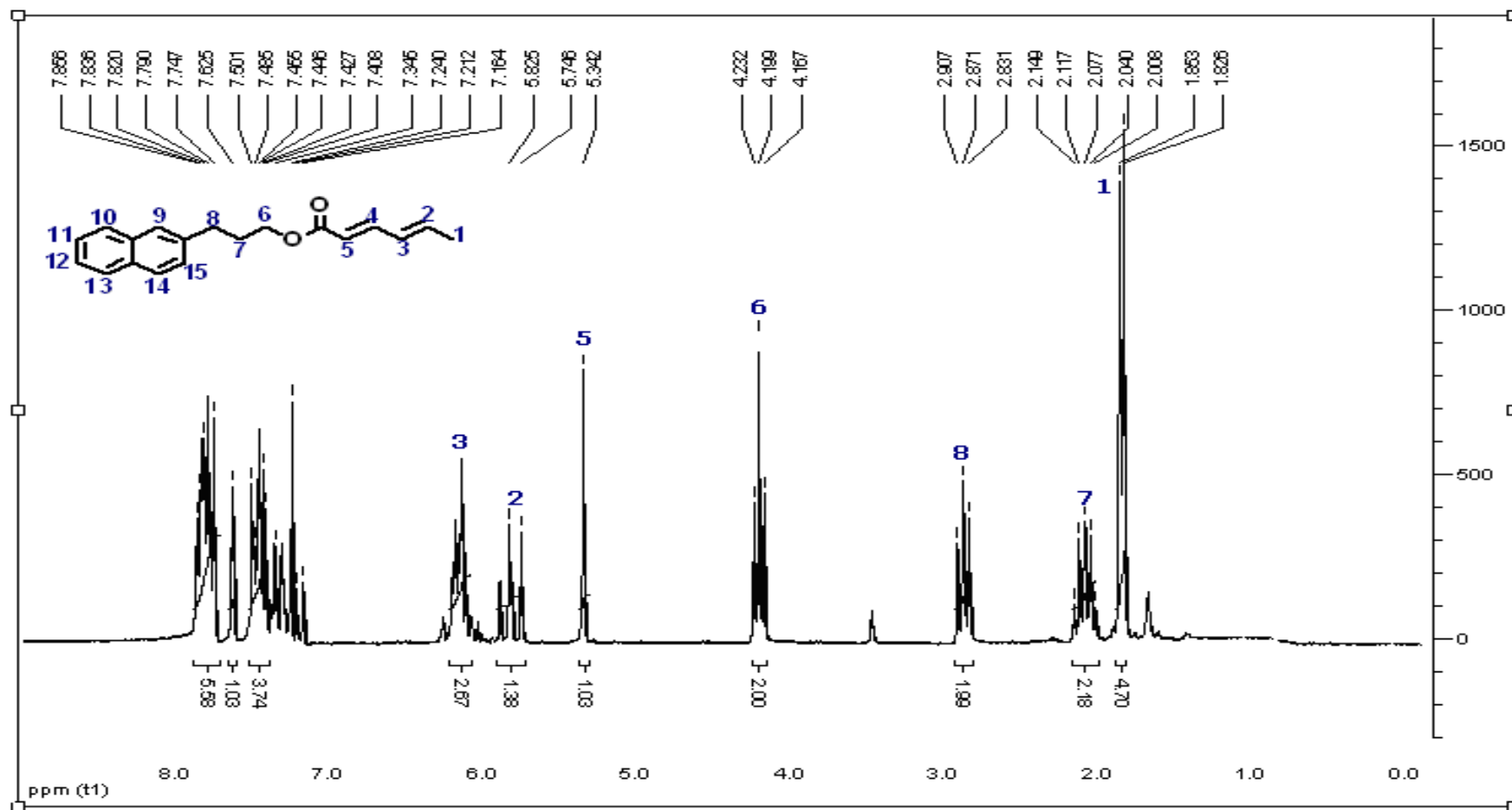
Espectro 8.9: Espectro de RMN 1 H do sorbato de 3- Naftilpropila ( 21 ) (CDCl 3 , 200 MHz).
