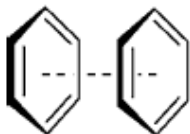
Figura 1.11: Dímero do benzeno, formado a partir da interação \pi - \pi stacking , adaptada da referência (SHERRILL et. al, 2006)
