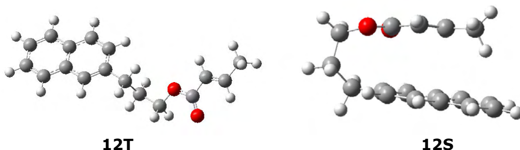
Figura 4.12: Estruturas de mínimo global para as conformações 12T e 12S.
