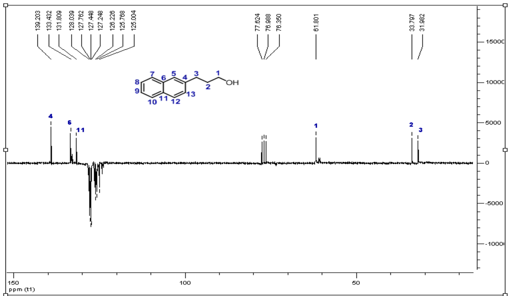
Espectro 8.3: Espectro de RMN 13 C - APT do 3-(Naftalen-2-il) propanol-1-ol ( 13 ) (CDCl 3 , 50 MHz).
