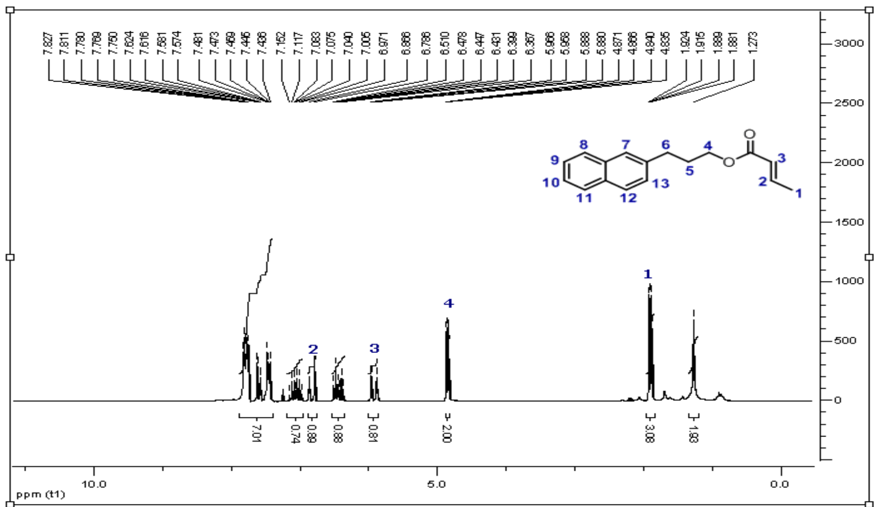
Espectro 8.5: Espectro de RMN 1 H do crotonato de 3- Naftilpropila ( 12 ) (CDCl 3 , 200 MHz).
