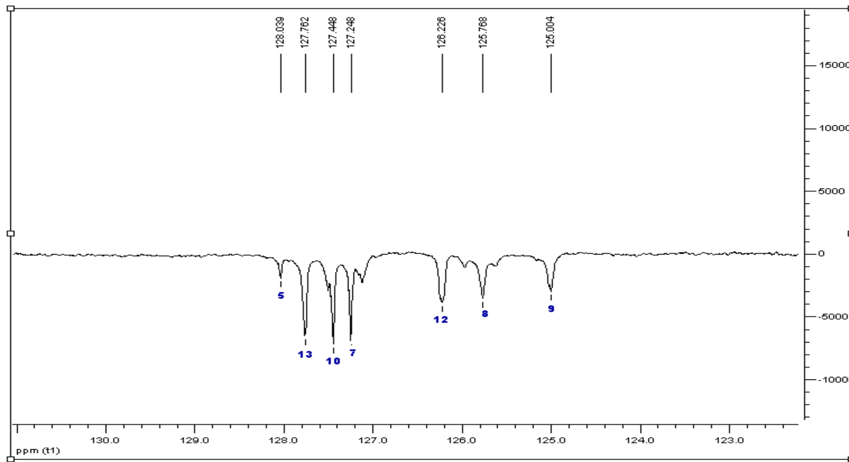
Espectro 8.4: Expansão do Espectro RMN 13 C - APT de 3-(Naftalen-2-il)propanol-1-ol ( 13 ) na região de 128,0 a 125,0 ppm (CDCl 3 , 50 MHz).
