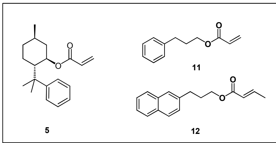
Figura 2.1: Moléculas estudadas nesta dissertação.
