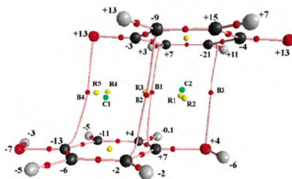
Figura 1.12: Complexo intermolecular quinona-hidroquinona (quinidrona) adaptada da referência (MOA et al , 2007).
