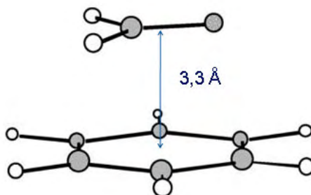
Figura 1.8: Interação \pi - \pi stacking entre o formaldeído e o benzeno, na distância de 3,3 Å, adaptada da referência (CARNEIRO et. al , 2001).
