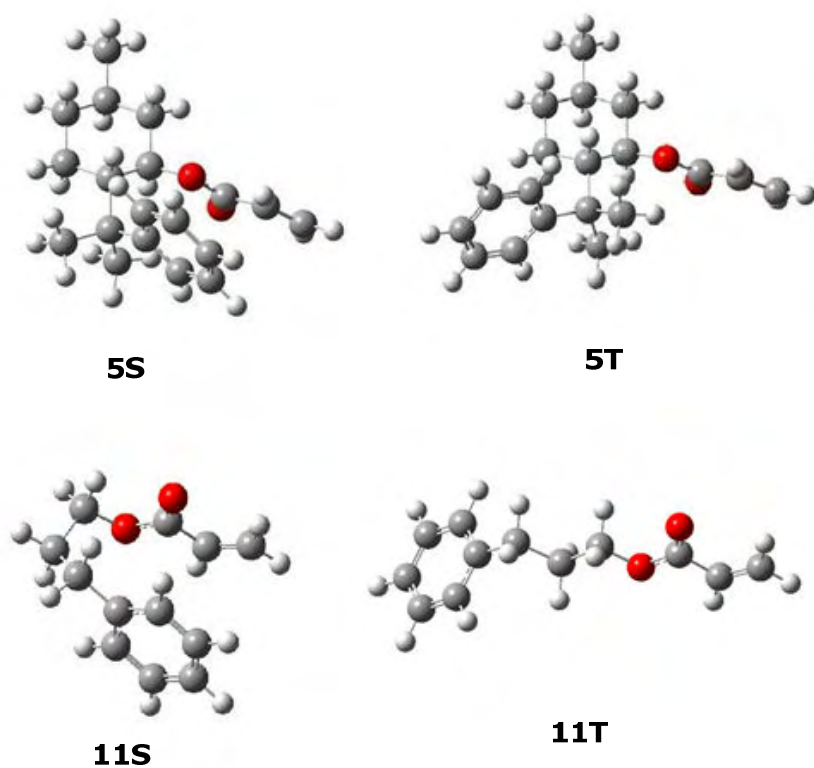
Figura 4.7: Geometrias minimizadas usando MPW1B95/6-311++G(2d,2p) 6d como nível de cálculo.
