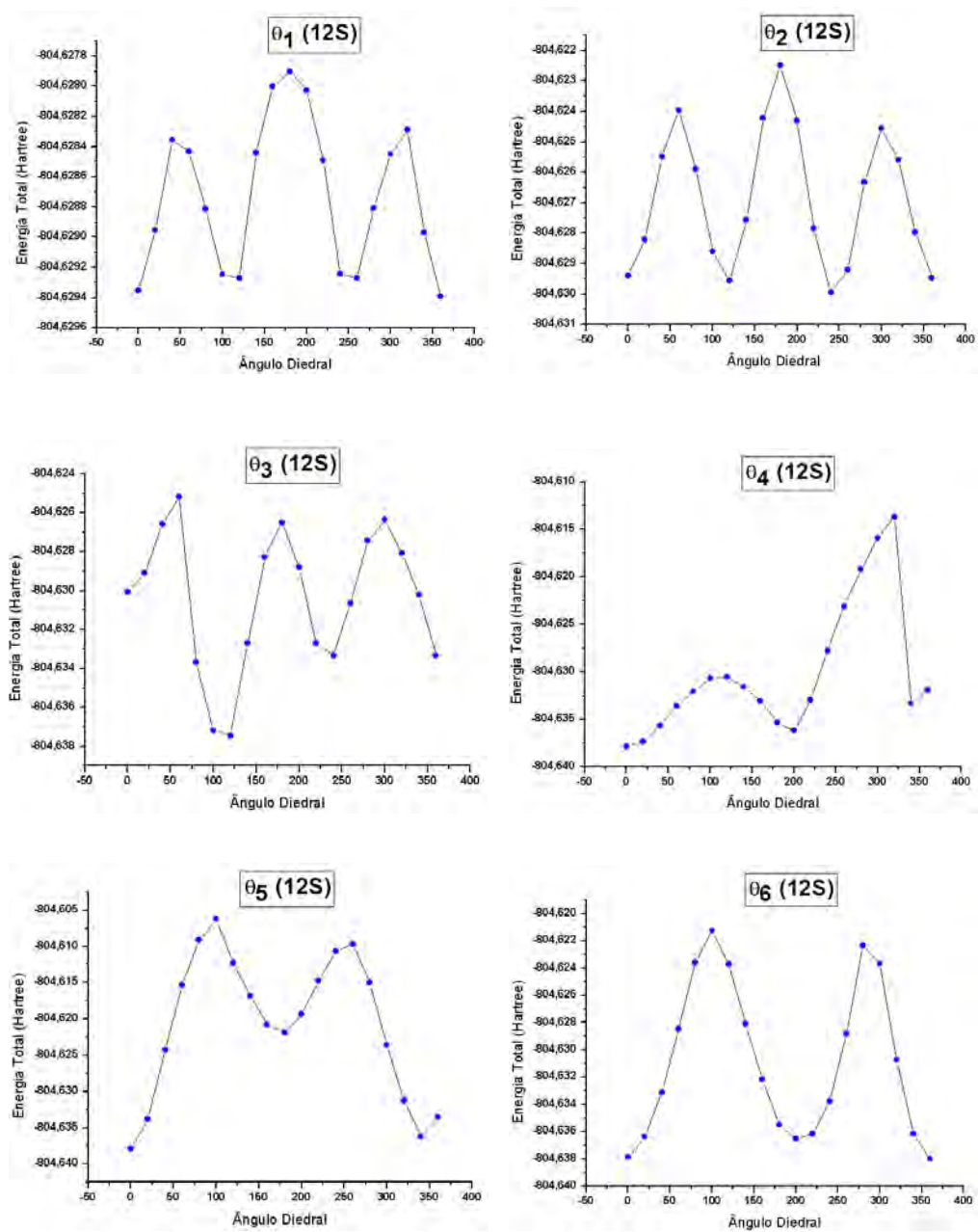
Figura 4.11: Curvas de energia potencial para a conformação 12S calculado com o método LSDA/6-31G(d).
