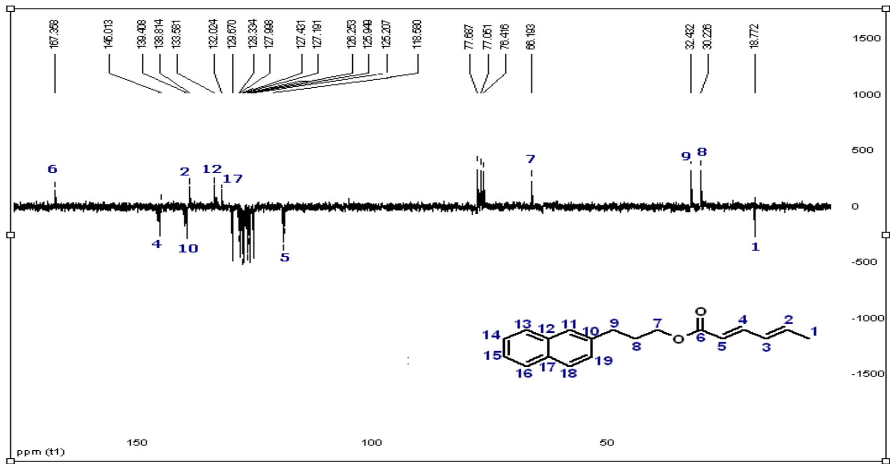
Espectro 8.11: Espectro de RMN 13 C - APT do sorbato de 3- Naftilpropila ( 21 ) (CDCl 3 , 50 MHz).
