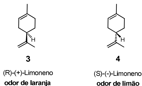
Figura 1.2: Configuração (R) e (S) do Limoneno.
