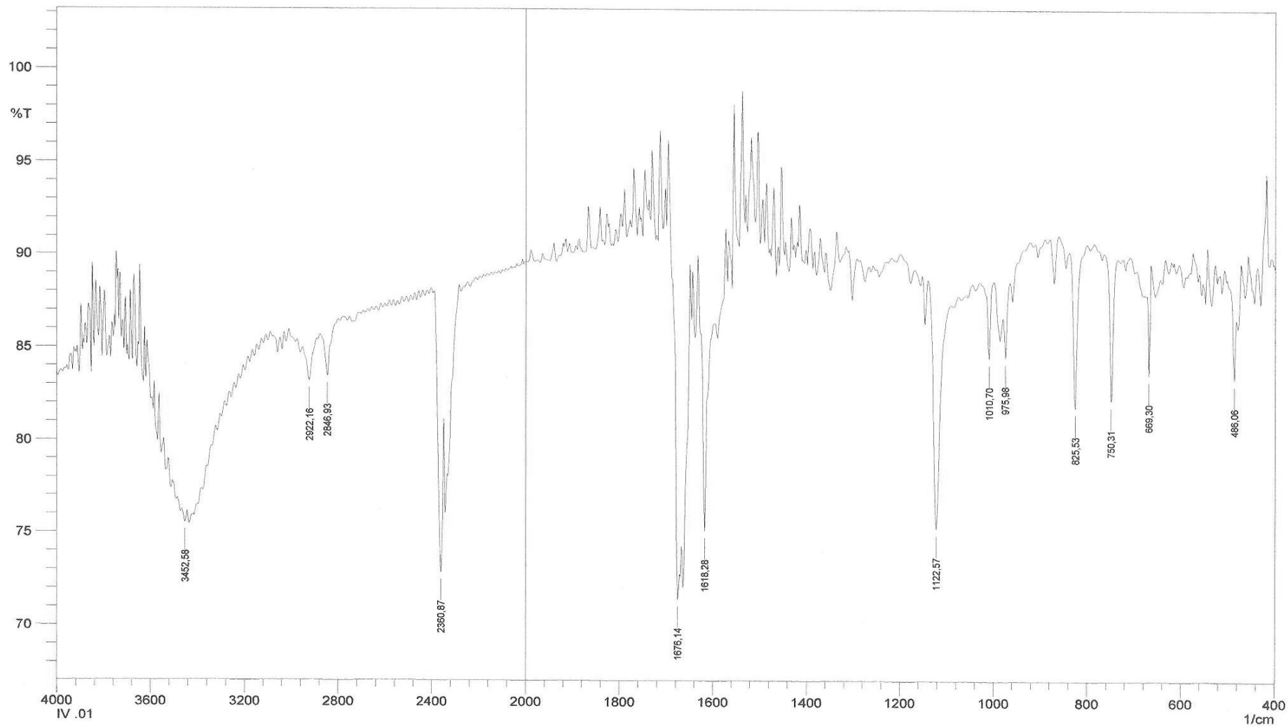
Espectro 8.1: Espectro de IV ( \text{cm}^{-1} ) de 15 .
