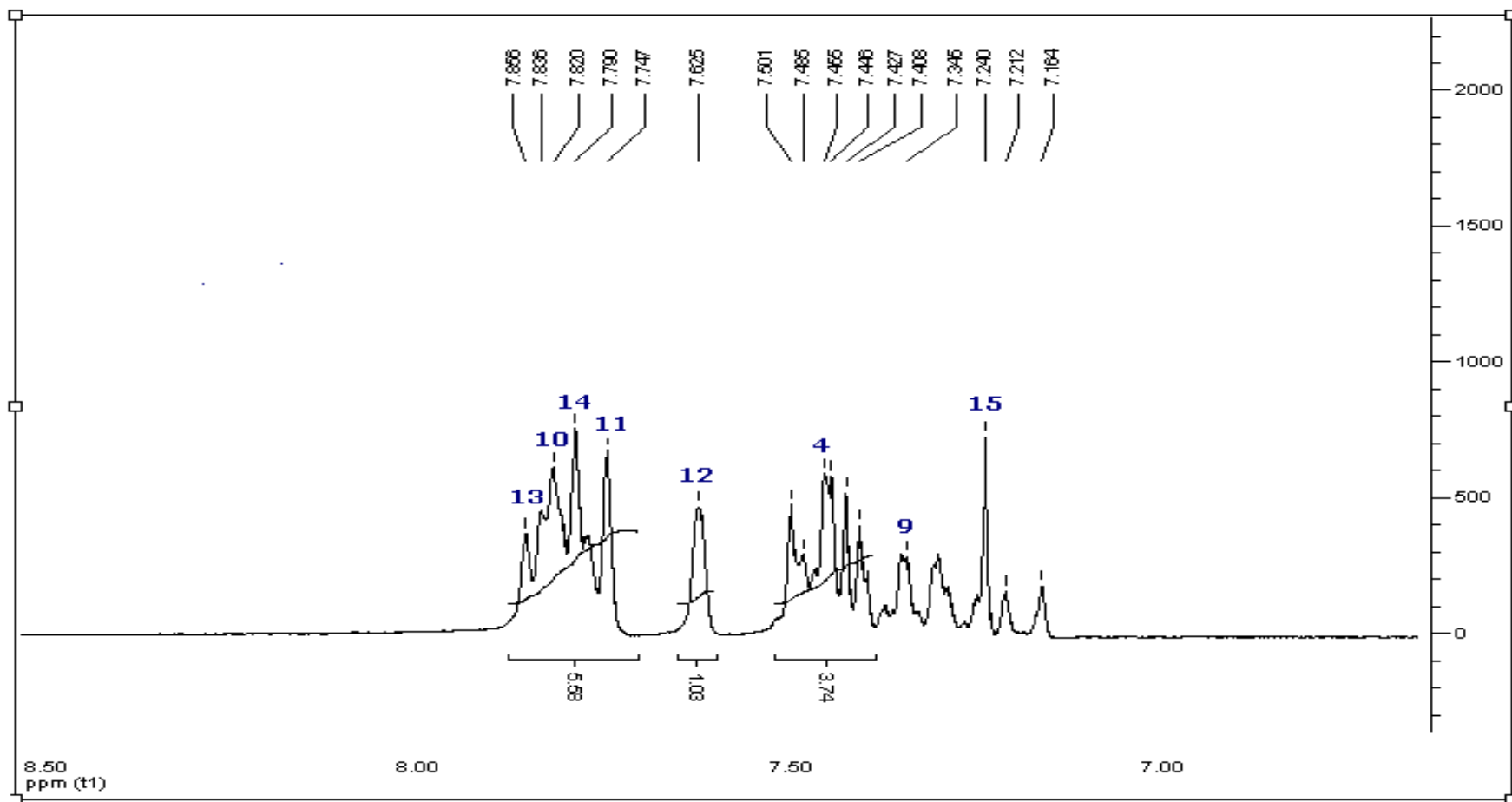
Espectro 8.10: Expansão do Espectro RMN 1 H do sorbato de 3- Naftilpropila ( 21 ) na região de 7,8 a 7,1 ppm (CDCl 3 , 200 MHz).
