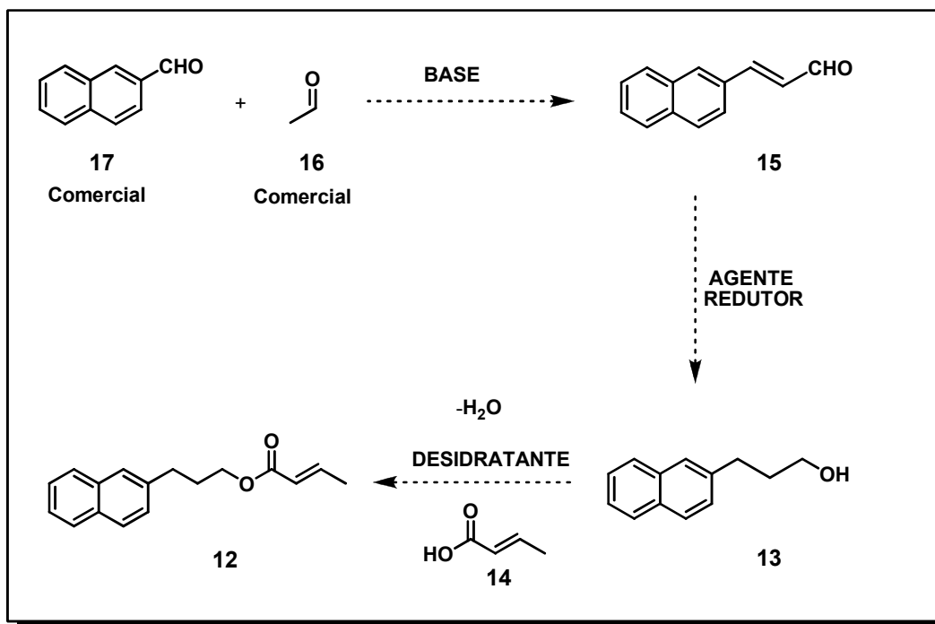
Esquema 3.2: Metodologia da síntese proposta para a obtenção do crotonato de 3-naftilpropila 12 .
