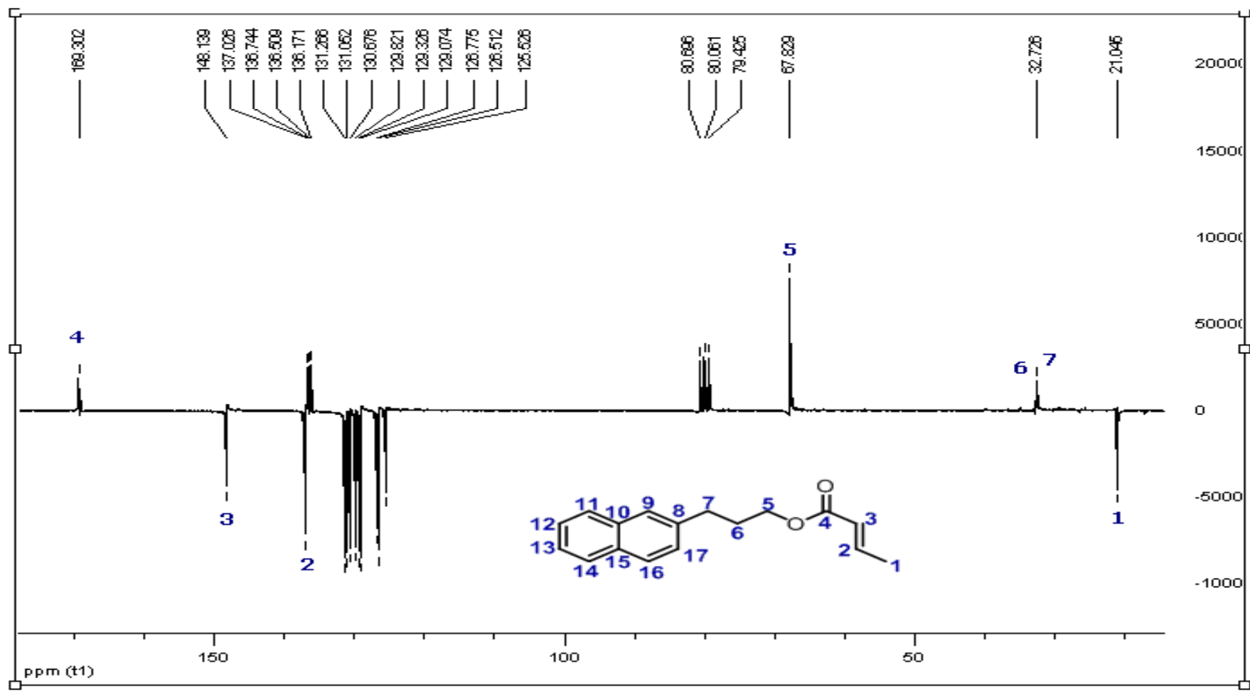
Espectro 8.7: Espectro de RMN 13 C - APT do Crotonato de 3-naftilpropila ( 12 ) (CDCl 3 , 50 MHz).
