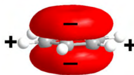
Figura 1.5: Região de blindagem (-) e desblindagem (+) anisotrópica do benzeno, adaptada de ( http://en.wikipedia.org/wiki/Cation-pi interaction ).
