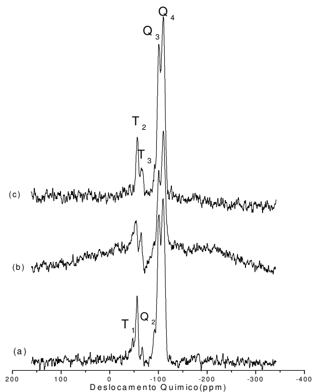
Figura 45 - Espectros de RMN de ^{29}\text{Si} das sílicas modificadas (a) Sil Cl e (b) SIL Cl AMP HETE e (c) SIL Cl PIP.
