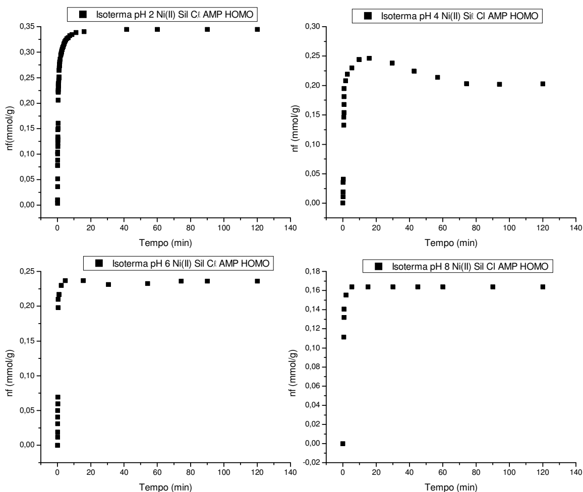
Figura 50 - Efeito do tempo e do pH na adsorção de Ni(II) na superfície SIL CL AMP HOMO.
