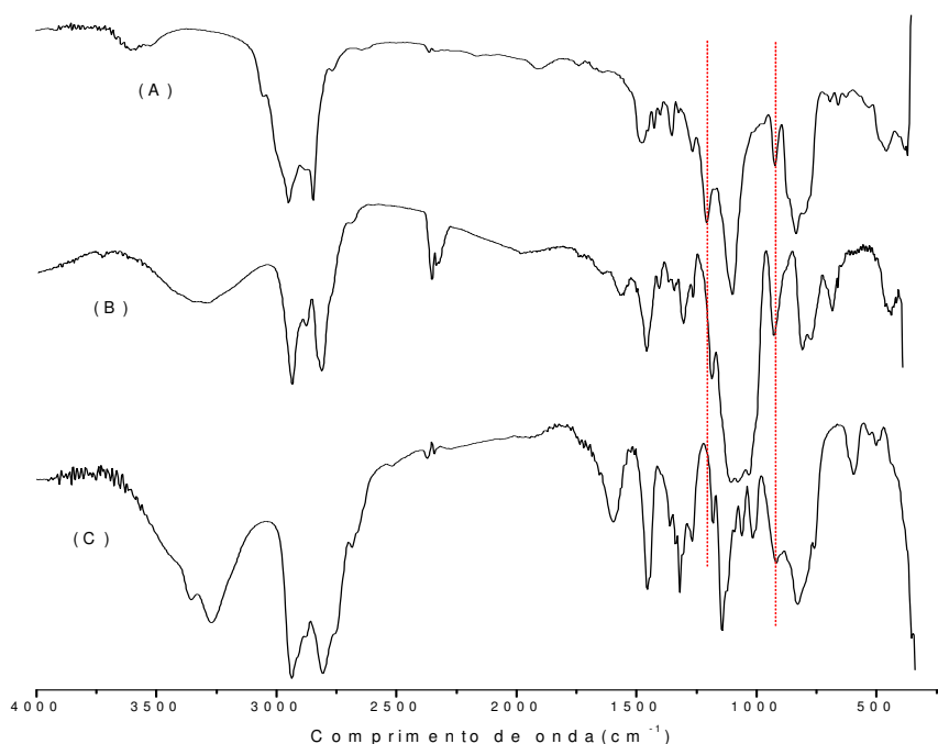
Figura 27 - Espectros na região do infravermelho para (a) 3-glicidoxipropiltrimetoxissilano, (b) sililante GLIC AMP e (c) 1-(2-aminoetil)-piperazina.
