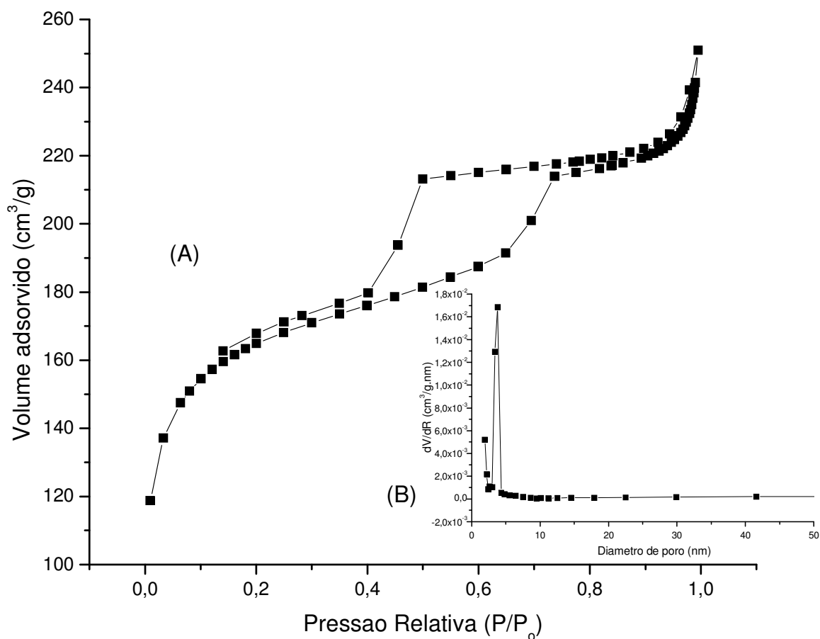
Figura 29 - (A) Isotherma de adsorção de \text{N}_2 e (B) curva de distribuição de poros na sílica Pura SBA-15 2M.
