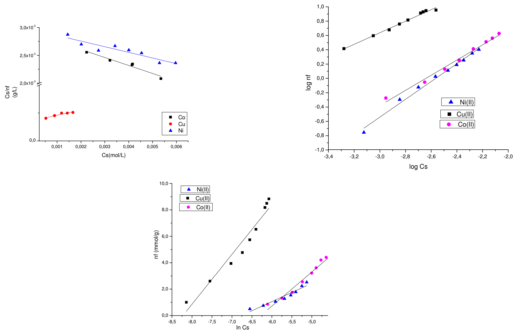
Figura 80 - Linearizações das isotermas de adsorção dos cátions de Co(II), Cu(II) e Ni(II) na superfície SIL CI AMPHOMO a 298 K aos modelos de Langmuir(A), Freundlich(B) e Temkin(C).
