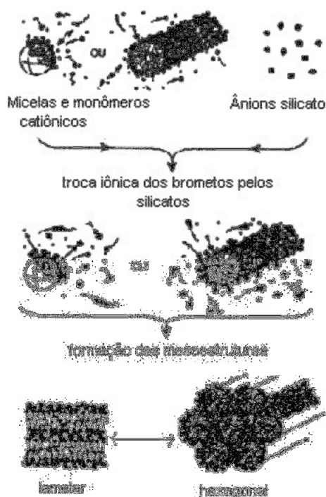
Figura 8 - Formação de um material mesoporoso através da rota cooperativa [RODRIGUES-ALVES et al, 2009].
