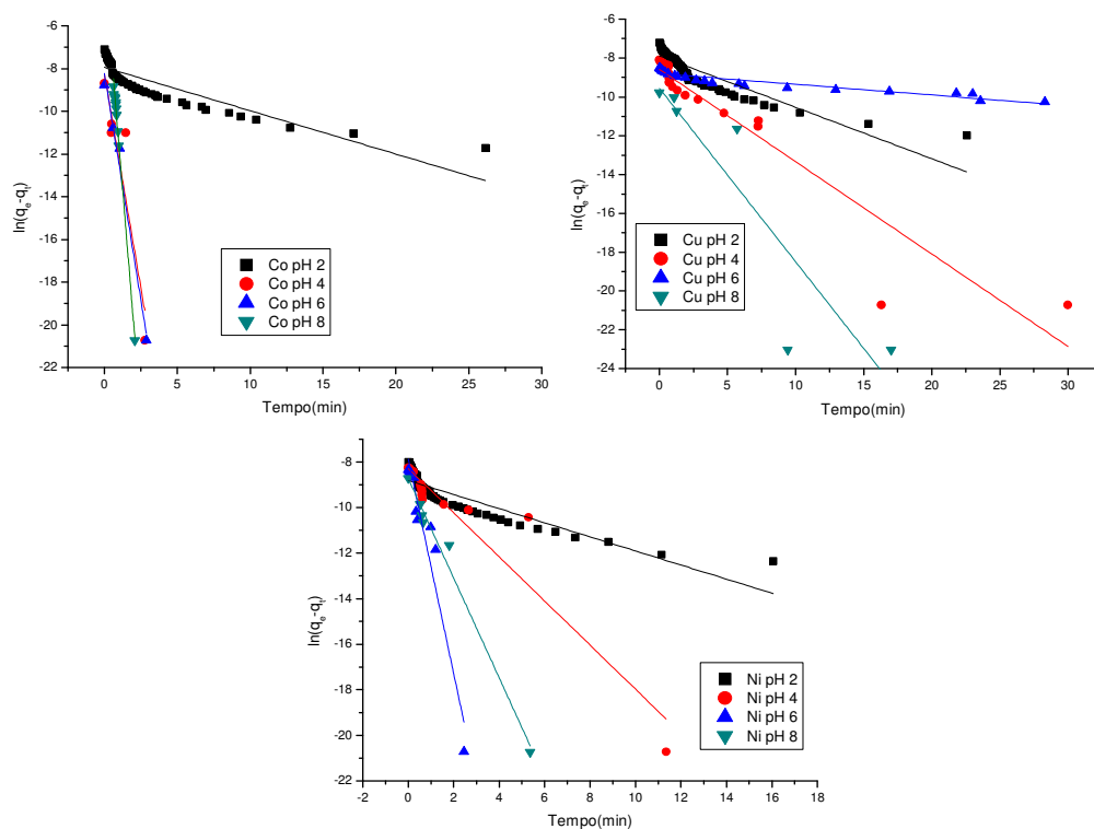
Figura 62 - Ajuste dos dados de adsorção da GLIC AMP HETE com Co(II), Cu(II) e Ni(II) a diferentes pH ao modelo de pseudo primeira ordem.
