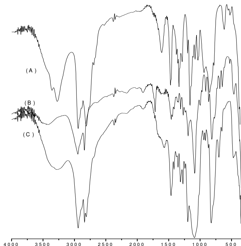
Figura 26 - Espectros de absorção na região do infravermelho da (a) 1-(2-aminoetil) piperazina, (b) 3-cloropropiltrimetoxissilano e (c) sililante CPTS AMP.
