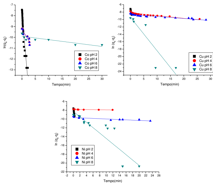
Figura 63 - Ajuste dos dados de adsorção da GLIC AMP HOMO com Co(II), Cu(II) e Ni(II) a diferentes pH ao modelo de pseudo primeira ordem.
