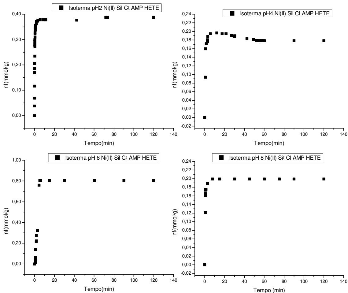
Figura 56 - Efeito do tempo e do pH na adsorção de Ni(II) na superfície SIL GLIC AMP HETE.
