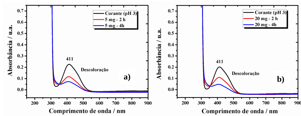
Figura 5.9. Espectros de UV-Vis das soluções do corante no pH 3, em tempos diferentes (a) 5 mg e (b) 20 mg de \text{KNbO}_3 .
