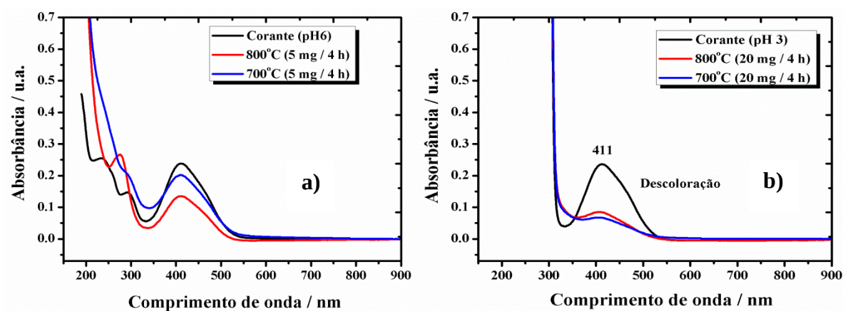
Figura 5.11. Espectros de UV-Vis das soluções do corante, em 700°C e 800°C (a) pH 6 (b) pH 3 do \text{KNbO}_3 .
