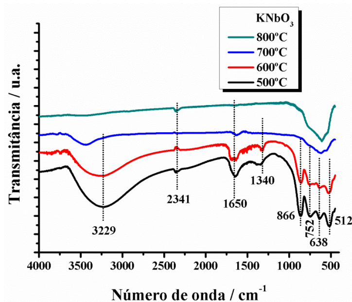
Figura 5.4. Espectros vibracionais na região do infravermelho de \text{KNbO}_3 calcinados em diferentes temperaturas.
