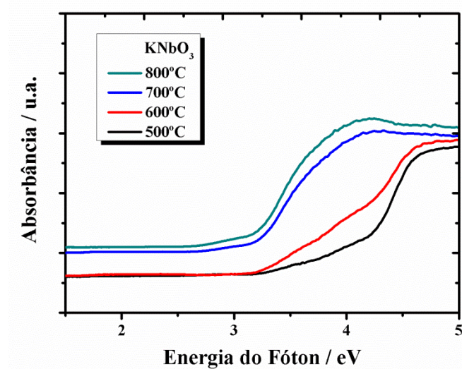
Figura 5.5. Espectros de absorbância na região do Ultravioleta-visível em elétron-volt do \text{KNbO}_3 , calcinados a 500°C, 600°C, 700°C e 800°C.
