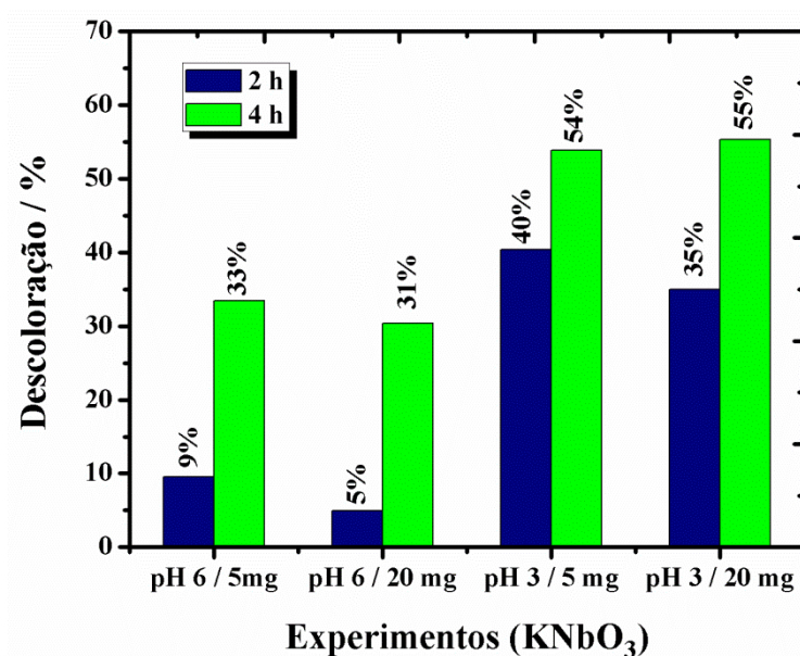
Figura 5.10. Resultados de descoloração referente à banda em 411 nm do grupo azo ( -\text{N}=\text{N}- ).
