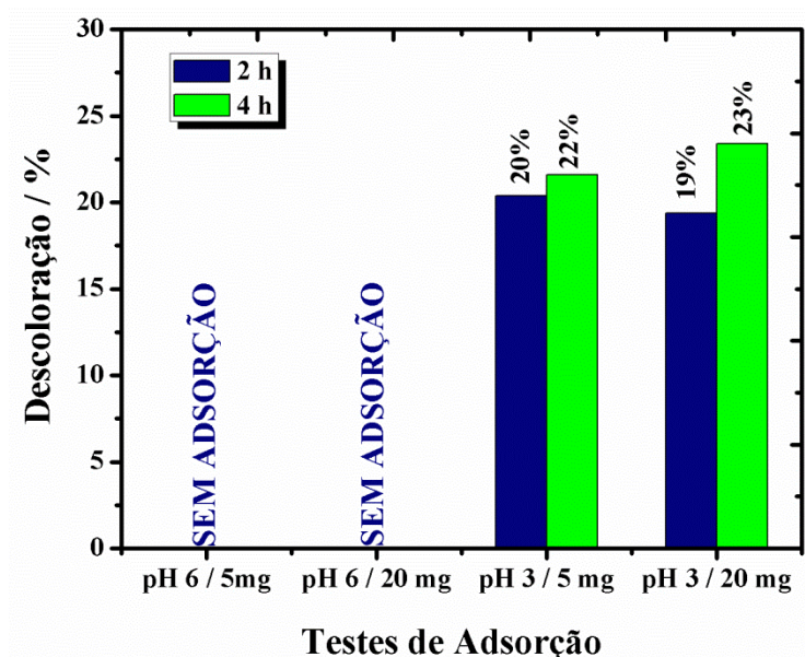
Figura 5.7. Testes de adsorção realizado nas amostras de \text{KNbO}_3 .
