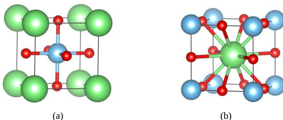
Figura 3.1. Representação esquemática da estrutura perovskita (a) cátion B em sítio octaédrico e (b) cátion A em sítio dodecaédrico. Legenda: as bolinhas em verde, azul e vermelho correspondem ao átomo A, B e O respectivamente. (Fonte: Adaptado de JOHNSON e LEMMENS, 2008).
