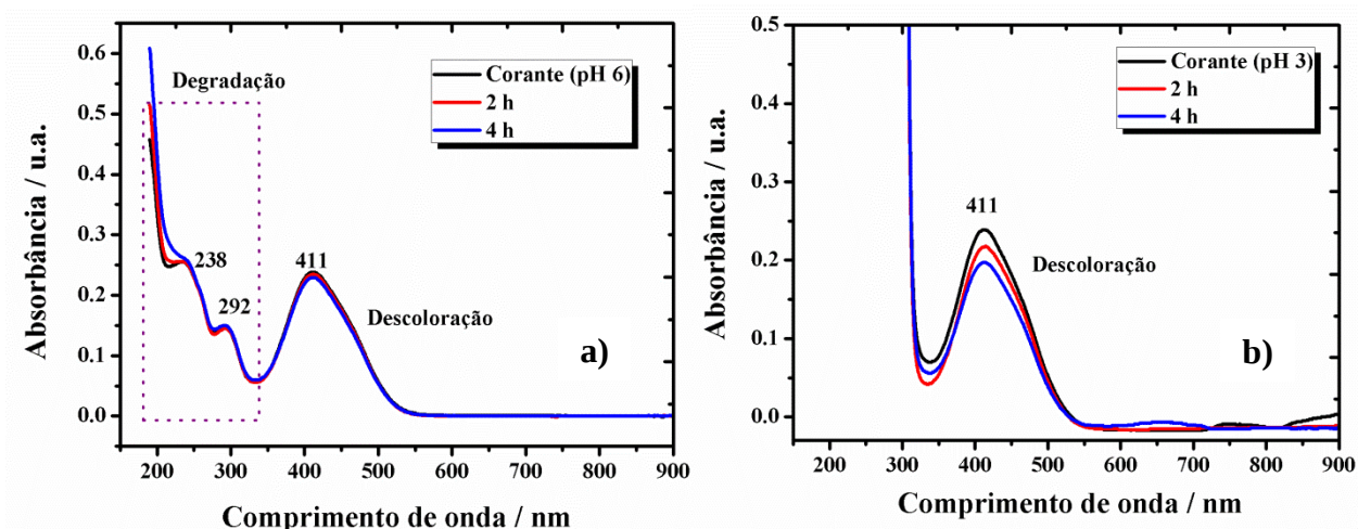
Figura 5.6. Espectros de UV-Vis das soluções do corante, em tempos diferentes (a) pH 6 e (b) pH 3 para o processo de fotólise direta.
