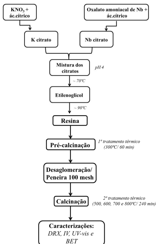
Figura 4.1. Fluxograma da rota de síntese do \text{KNbO}_3 .
