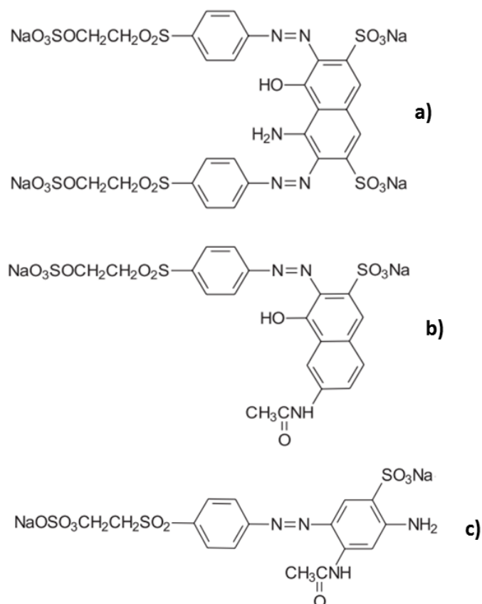
Figura 3.4. Representação das estruturas dos corantes: (a) preto remazol; (b) alaranjado remazol 3R e (c) amarelo ouro remazol RNL (CATANHO et al. , 2006).
