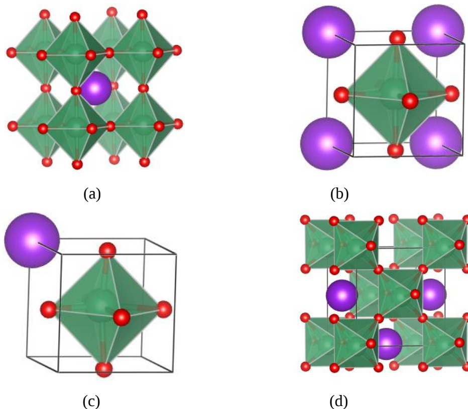
Figura 3.2. Representação gráfica das estruturas perovskitas do KNbO 3 (a) em arranjo cúbico, (b) tetragonal, (c) romboédrico e (d) ortorrômbico. Legenda: as bolinhas em roxo, verde e vermelho correspondem ao átomo K, Nb e O respectivamente. (Fonte: Adaptado de HEWAT, 1973).
