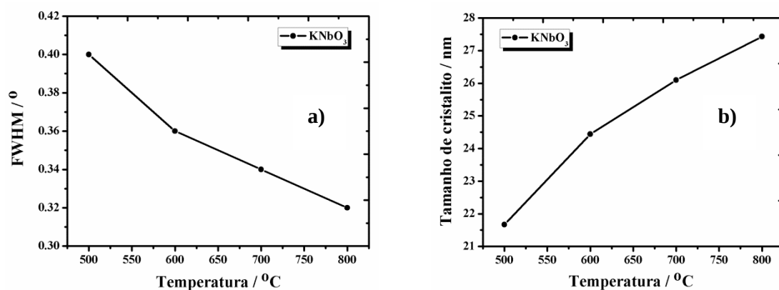
Figura 5.3. Representação gráfica: Valores de FWHM (a) e tamanho médio de cristalitos (b) das amostras de KNbO 3 calcinadas em 500°C, 600°C, 700°C e 800°C.
