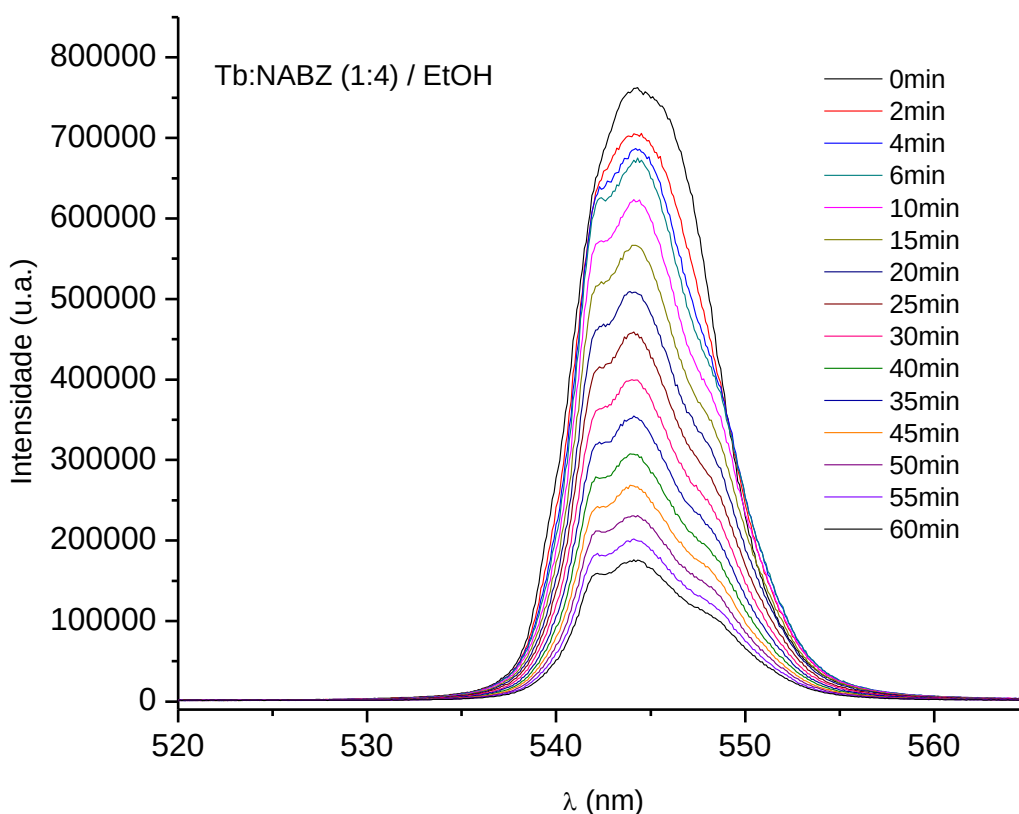
Figura 4.32 – Espectros de emissão da reação \text{Tb}:\text{NABZ} (1:4) no intervalo de 520 a 566 nm, registrados a temperatura ambiente, durante 1 hora.
