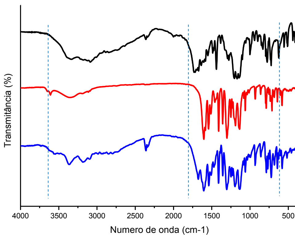
Figura 27. Espectros de absorção na região do Infravermelho: (a) NTF2AP, (b) Eu(TTA) 3 (H 2 O) 2 e (c) Eu(TTA) 3 (NTF2AP) 2 .
