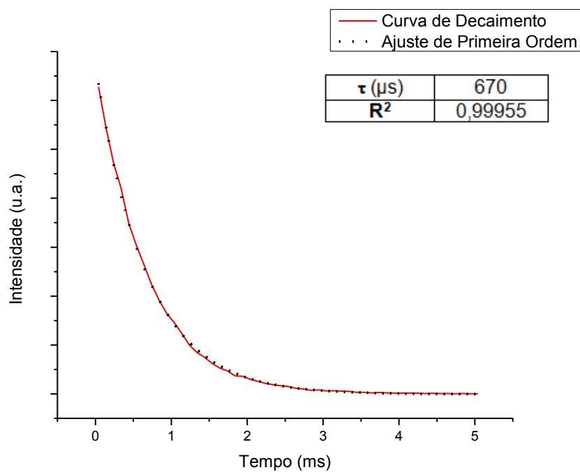
Figura 50. Curvas de decaimento de luminescência do [\text{Eu}(\text{TTA})_3(\text{NTF}_2\text{AP})_2] , registradas a temperatura ambiente.
