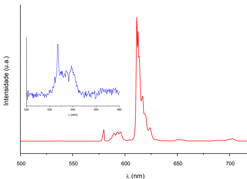
Figura 44. Espectro de emissão do (\text{Et}_3\text{NH})[\text{Eu}(\text{BZAC})_4] a temperatura de nitrogênio líquido, com excitação em 370 nm.
