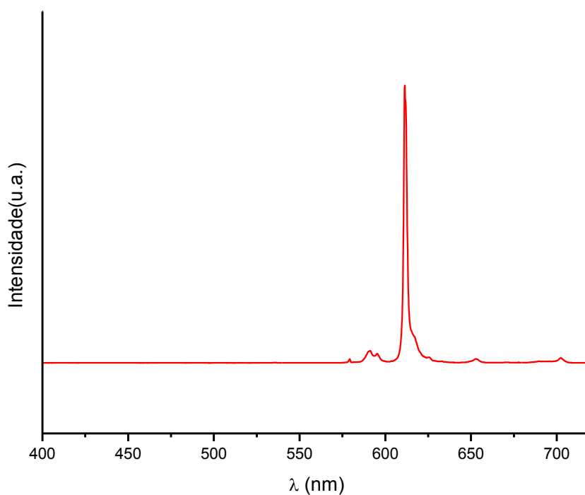
Figura 38. Espectro de emissão do \text{Eu}(\text{TTA})_3(\text{NTF2AP})_2 a temperatura ambiente, com excitação em 370 nm.
