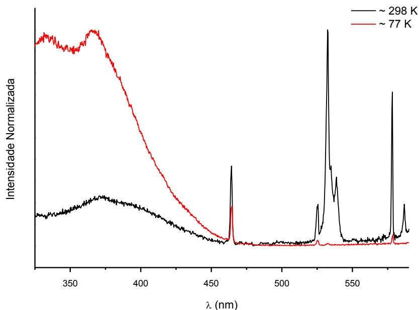
Figura 28. Espectros de excitação do \text{Eu}(\text{BZAC})_3(\text{H}_2\text{O})_2 a temperatura ambiente e de nitrogênio líquido, monitorada em 612 nm.
