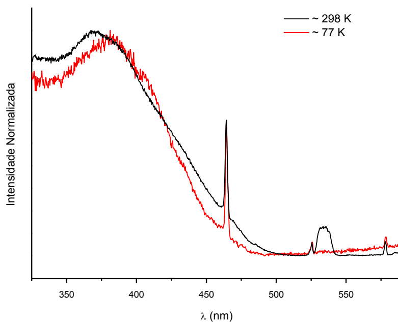
Figura 29. Espectro de excitação do \text{Eu}(\text{TTA})_3(\text{H}_2\text{O})_2 a temperatura ambiente e de nitrogênio líquido, monitorada em 612 nm.
