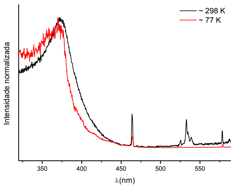
Figura 30. Espectro de excitação do \text{Eu(BZAC)}_3(\text{NAC2AP}) a temperatura ambiente e de nitrogênio líquido, monitorada em 612 nm.
