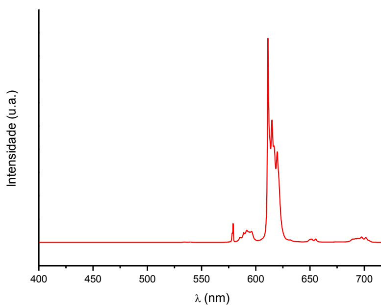
Figura 37. Espectro de emissão do \text{Eu}(\text{TTA})_3(\text{H}_2\text{O})_2 a temperatura ambiente, com excitação em 370 nm.
