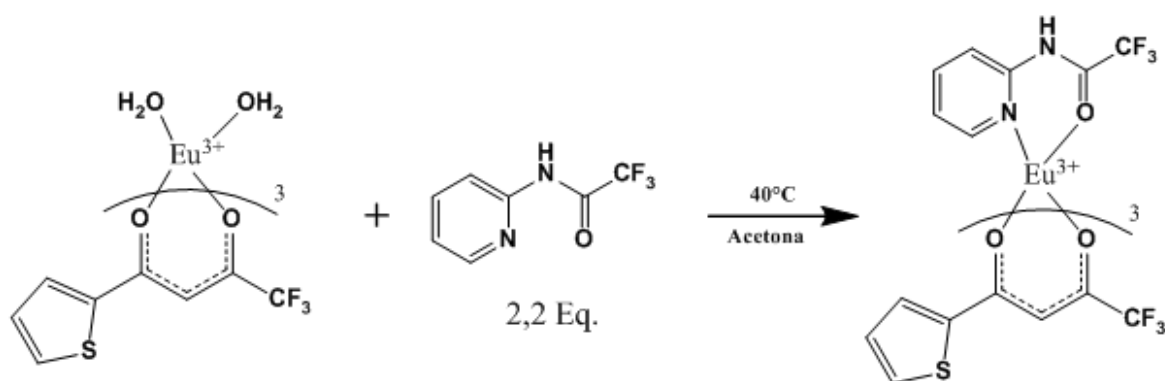
Figura 25. Esquema de síntese proposta para o complexo contendo o ligante N-(trifluoroacetil)-2-aminopiridina.
