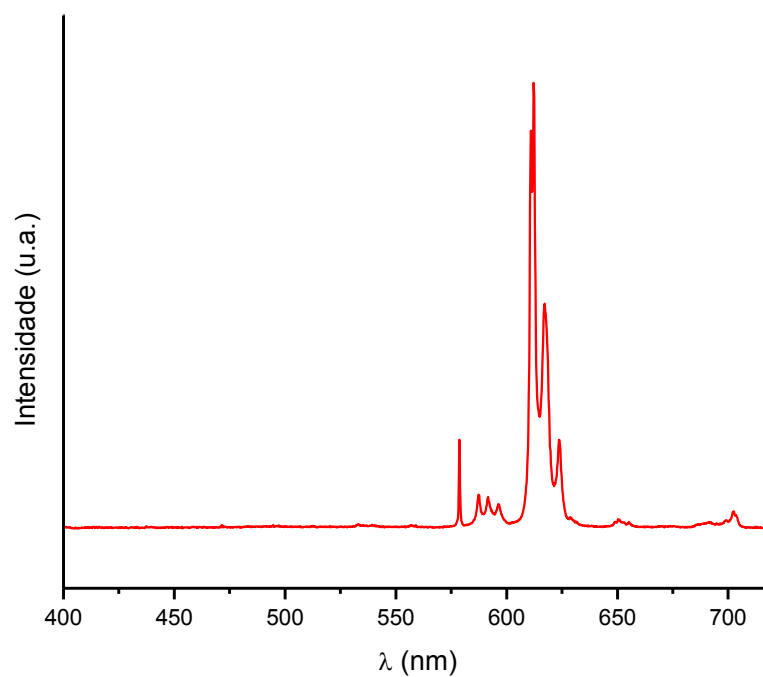
Figura 34. Espectro de emissão do \text{Eu}(\text{BZAC})_3(\text{H}_2\text{O})_2 a temperatura ambiente, com excitação em 370 nm.
