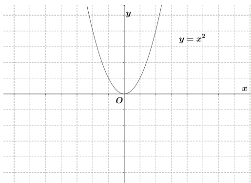
Figura 3.4: Gráfico da função quadrática y = x^2 no plano cartesiano Oxy .
