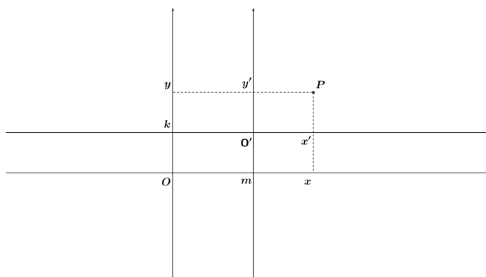
Figura 3.1: Translação de eixos
