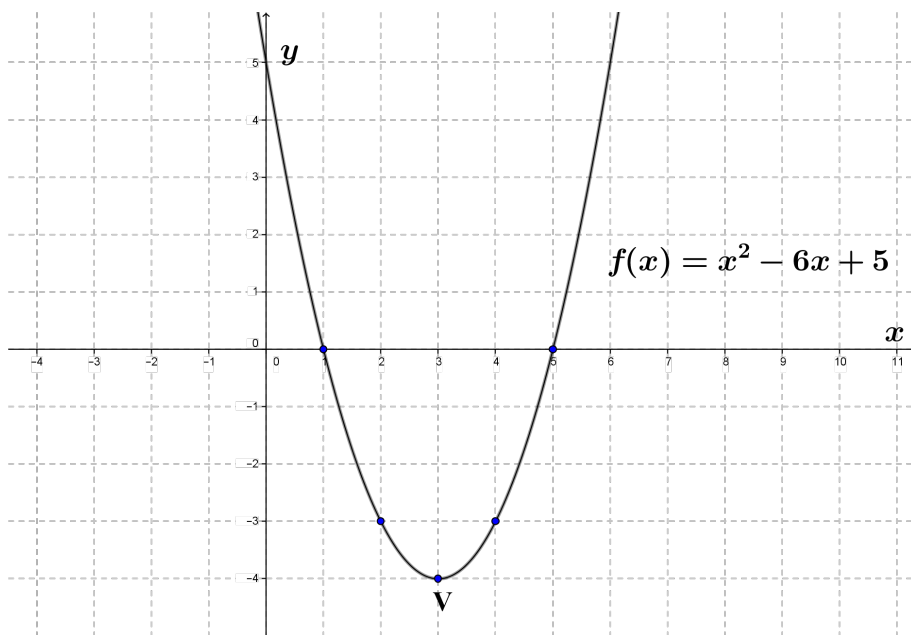
Figura 1.3: Gráfico da função quadrática f(x) = x^2 - 6x + 5 .
