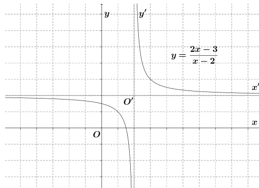
Figura 3.3: Gráfico da função hipérbole y = \frac{1}{x} transladado duas unidades para cima e duas para a direita.
