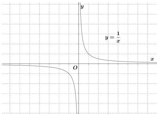
Figura 3.2: Gráfico da função hipérbole y = \frac{1}{x} no plano cartesiano Oxy .
