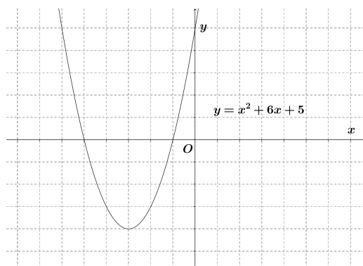
Figura 3.8: Gráfico da função quadrática y = x^2 + 6x + 5 no plano cartesiano Oxy .
