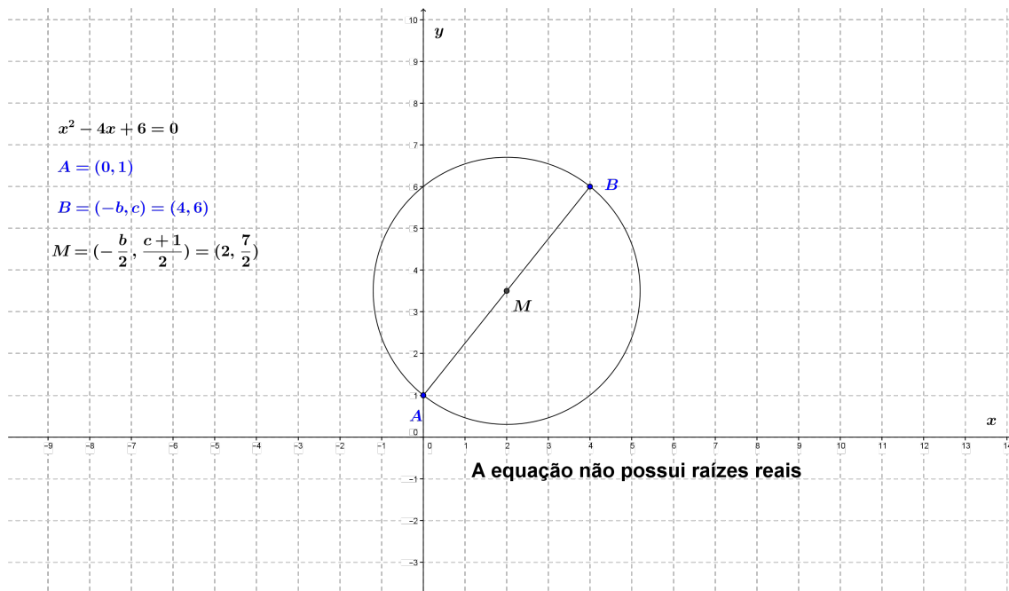
Figura 2.9: Solução geométrica da equação x^2 - 4x + 6 = 0 .
