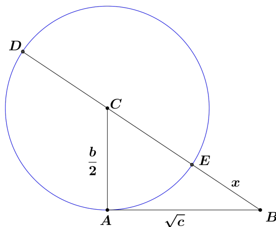
Figura 2.3: Construção de Descartes ( x^2 + bx = c ).
