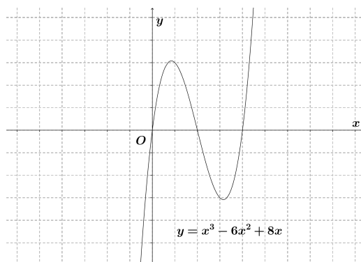
Figura 3.6: Gráfico da função cúbica y = x^3 - 6x^2 + 8x no plano cartesiano Oxy .
