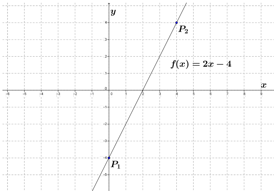
Figura 1.2: Gráfico da função afim f(x) = 2x - 4 .
