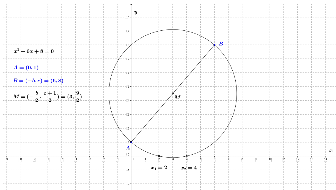
Figura 2.7: Solução geométrica da equação x^2 - 6x + 8 = 0 .
