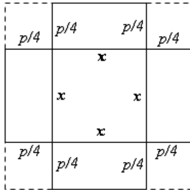
Figura 2.2: Construção de Al-Khwarizmi.
