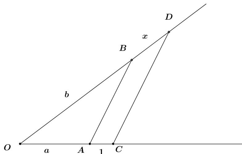
Figura 2.1: Solução geométrica da equação do 1º grau.
