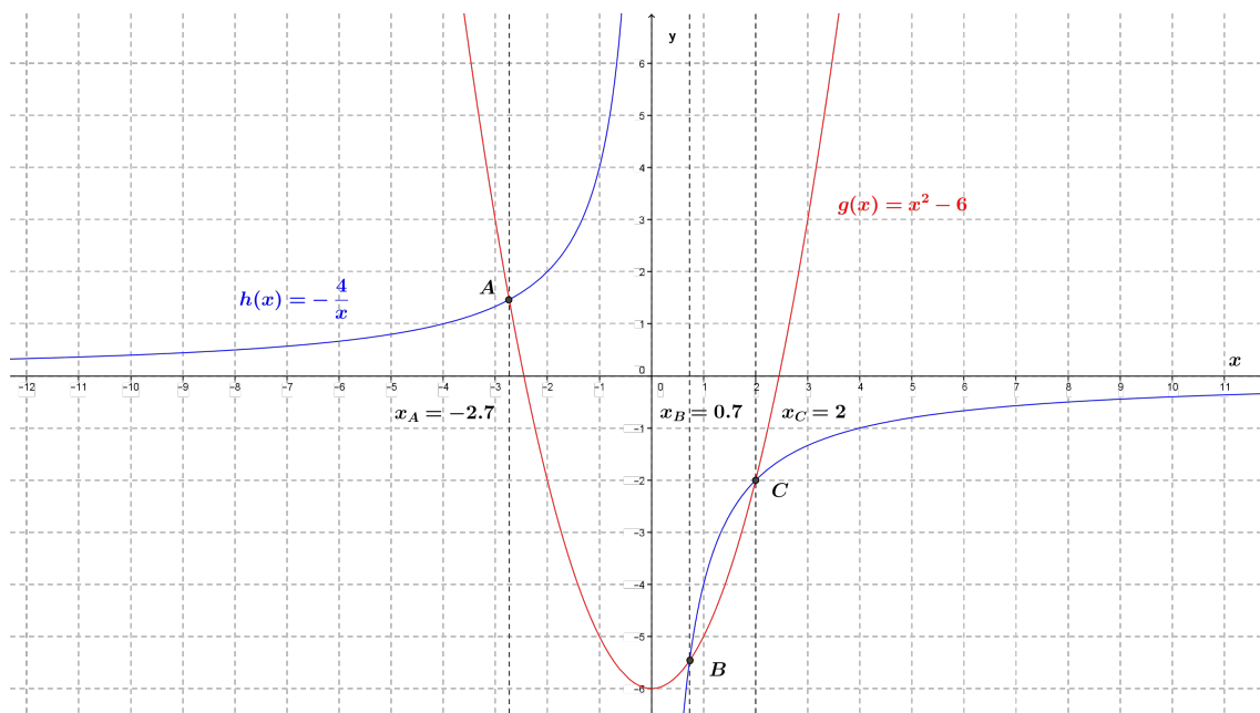
Figura 2.13: Solução geométrica da equação x^3 - 6x + 4 = 0 .
