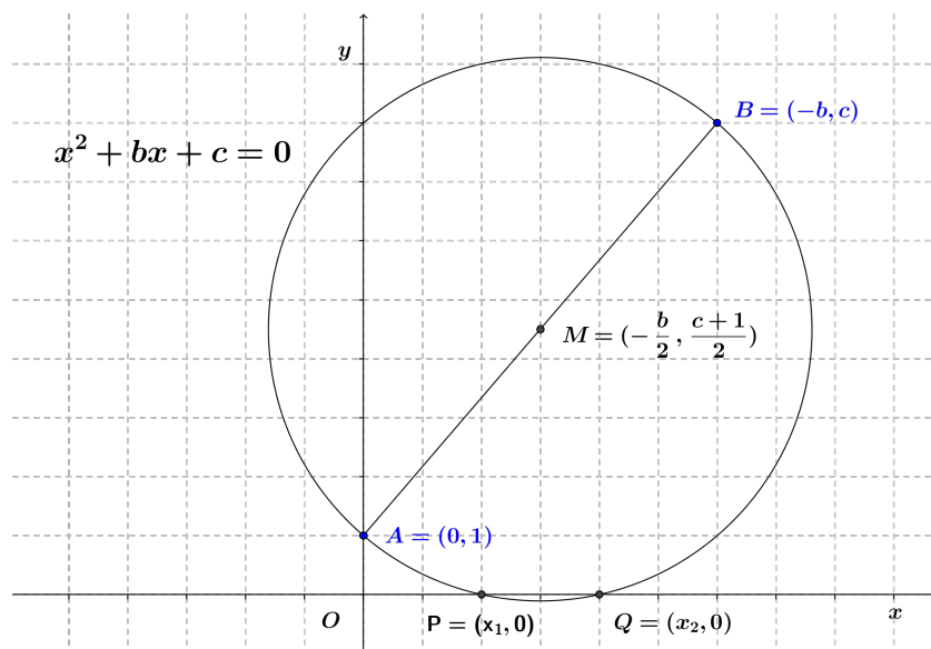
Figura 2.6: Construção de Thomas Carlyle.
