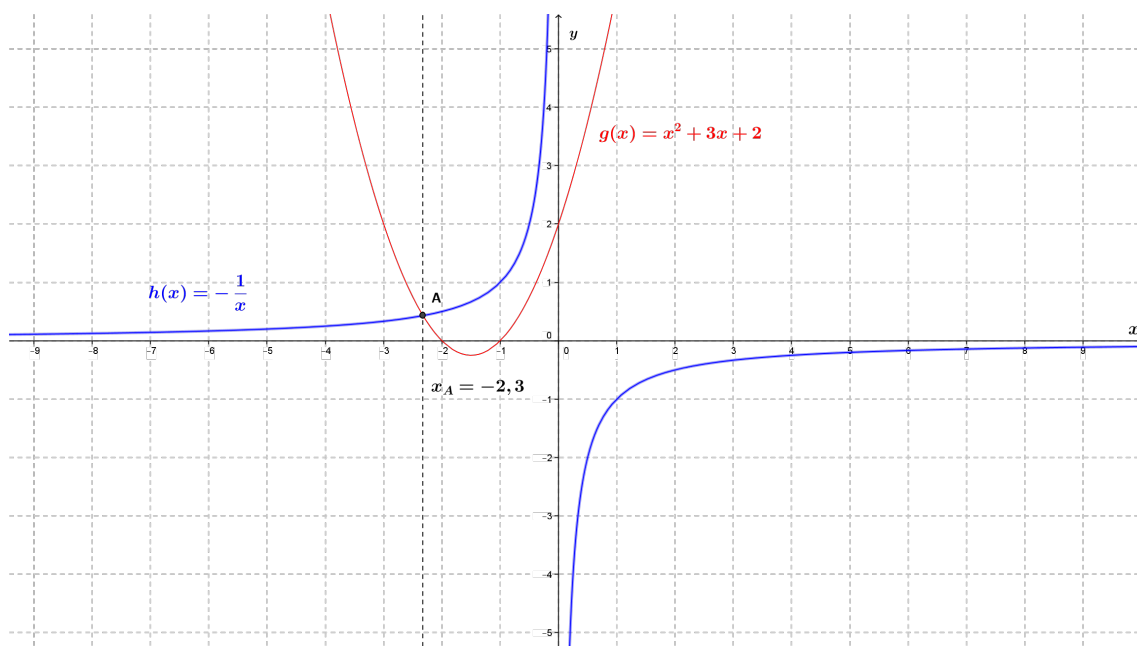
Figura 2.11: Solução geométrica da equação x^3 + 3x^2 + 2x + 1 = 0 .
