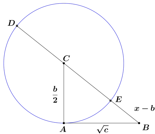
Figura 2.4: Construção de Descartes ( x^2 = bx + c ).
