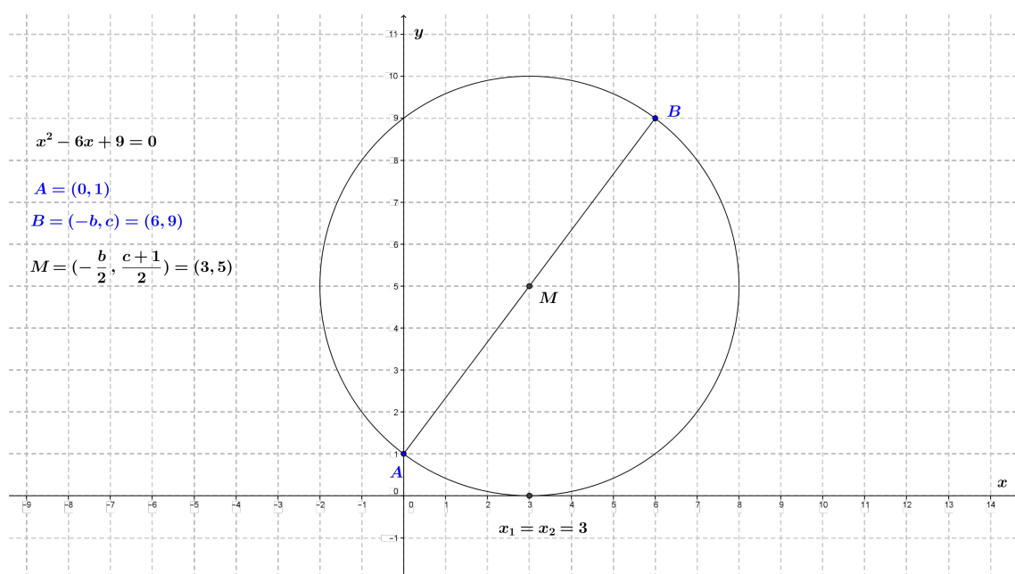
Figura 2.8: Solução geométrica da equação x^2 - 6x + 9 = 0 .
