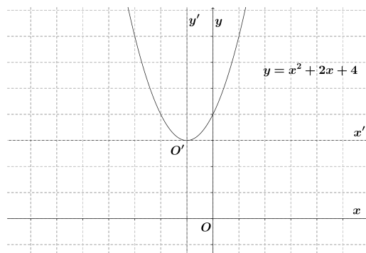
Figura 3.5: Gráfico da função quadrática y = x^2 transladado três unidades para cima e uma para a esquerda.
