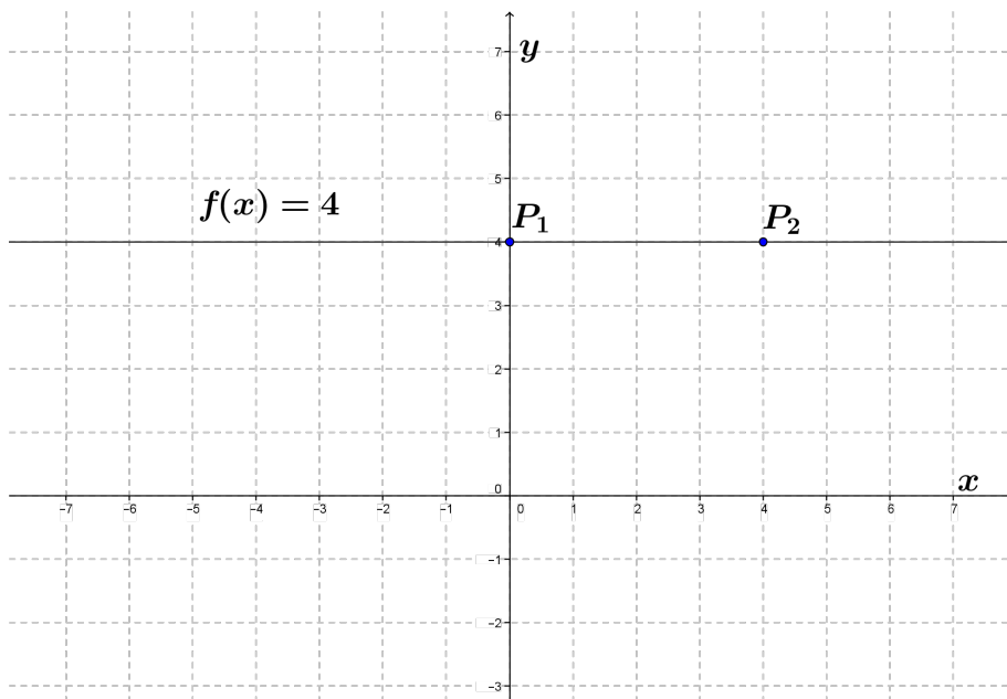
Figura 1.1: Gráfico da função constante f(x) = 4 .
