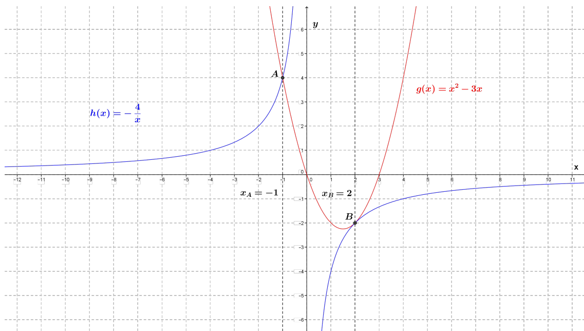
Figura 2.12: Solução geométrica da equação x^3 - 3x^2 + 4 = 0 .
