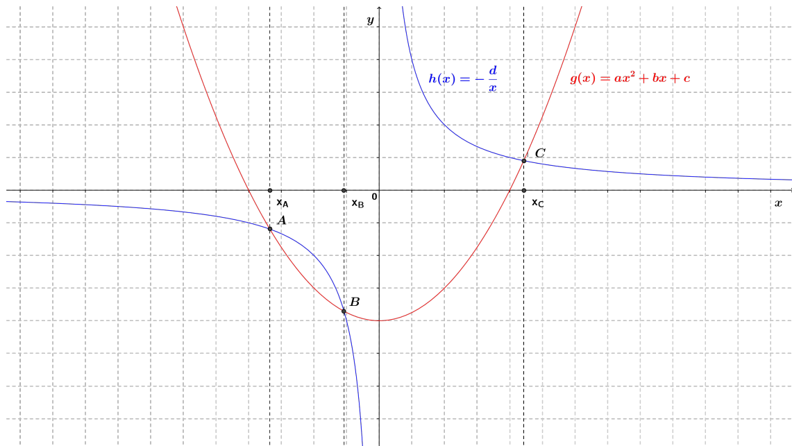
Figura 2.10: Solução geométrica da equação do 3º grau.
