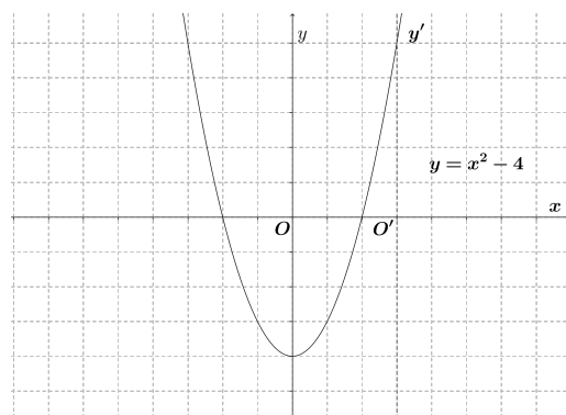
Figura 3.9: Gráfico da função quadrática y = x^2 + 6x + 5 transladado três unidades para a direita.
