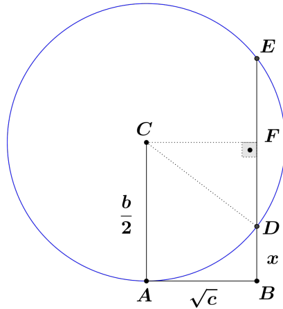
Figura 2.5: Construção de Descartes ( x^2 + c = bx ).
