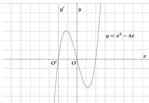
Figura 3.7: Gráfico da função cúbica y = x^3 - 6x^2 + 8x transladado duas unidades para a esquerda.
