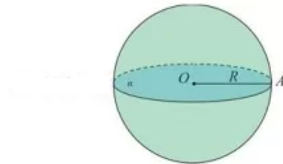
Figura 3.3: Círculo Máximo
