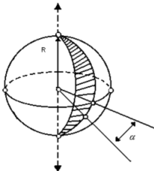
Figura 3.6: Fuso Esférico
