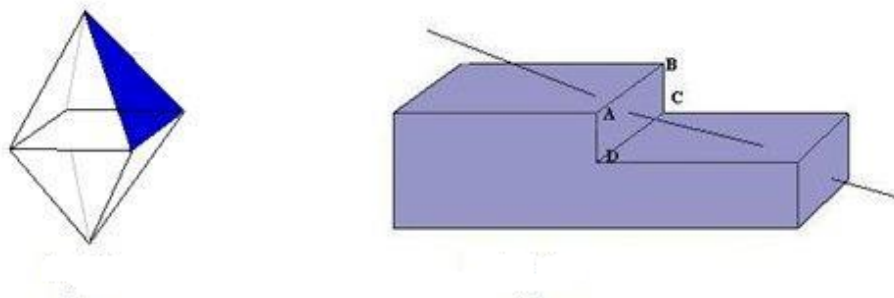
Figura 2.3: Poliedro convexo e não convexo
