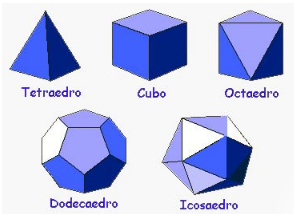
Figura 2.6: Poliedros de Platão
