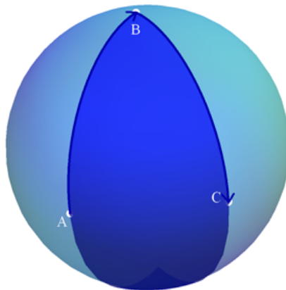
Figura 3.4: ângulo esférico
