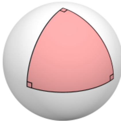
Figura 3.5: Triângulo esférico
