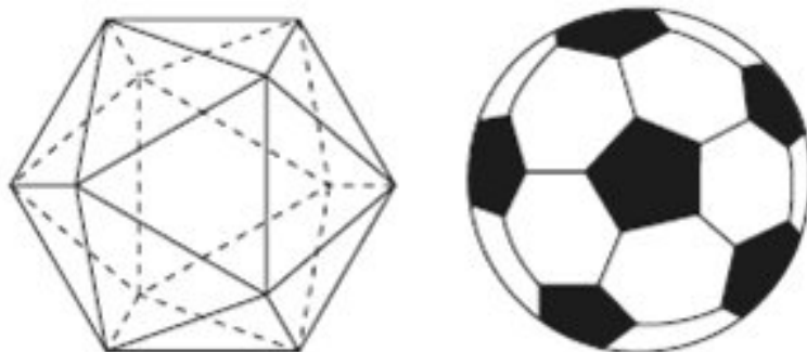
Figura 2.4: Poliedro e a bola de 1970
