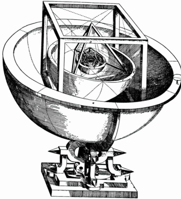
Figura 2.5: Modelo de Kepler para os planetas
