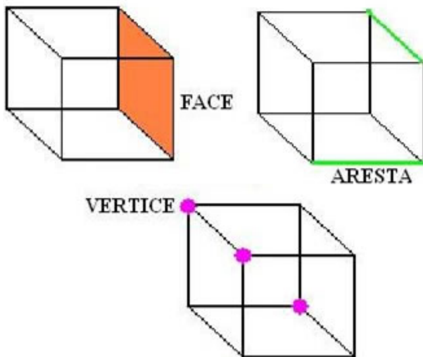
Figura 2.2: Elementos de um poliedro
