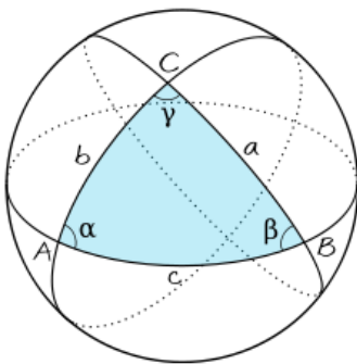
Figura 3.7: Triângulo Esférico
