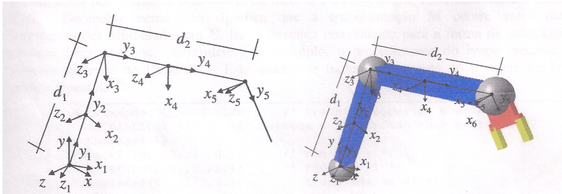
Figura 2.12: Eixos locais do braço mecânico
