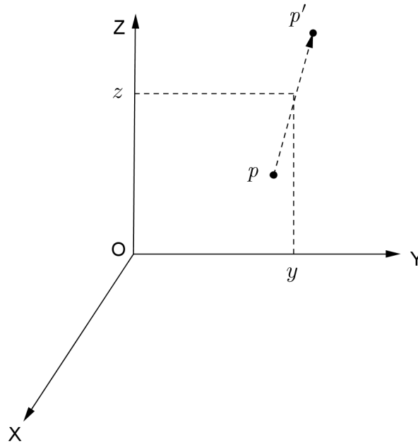
Figura 2.4: Transformação de reflexão em relação ao plano yOz
