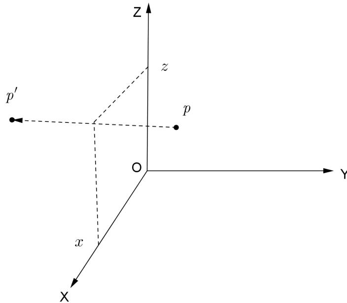
Figura 2.3: Transformação de reflexão em relação ao plano xOz
