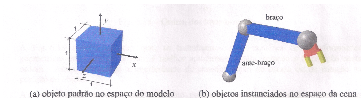
Figura 2.11: Instanciação de objetos num braço mecânico simples
