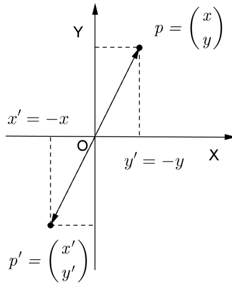
Figura 1.9: Transformação de espelhamento em relação a origem
