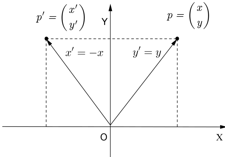
Figura 1.8: Transformação de espelhamento em relação ao eixo y
