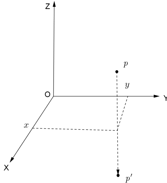
Figura 2.2: Transformação de reflexão em relação ao plano xOy
