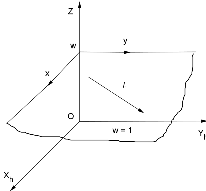
Figura 1.17: Imersão do \mathbb{R}^2 no sistema homogêneo x_h, y_h e w
