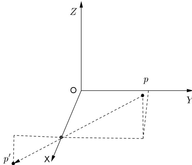
Figura 2.5: Transformação de reflexão em relação ao eixo x
