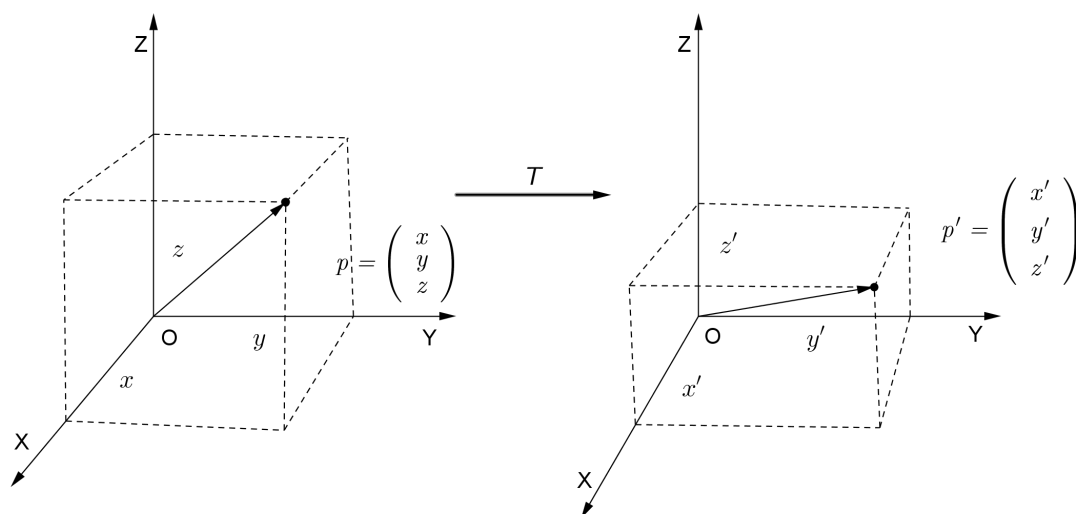
Figura 2.1: Transformação de \mathbf{p} em \mathbf{p}' no espaço
