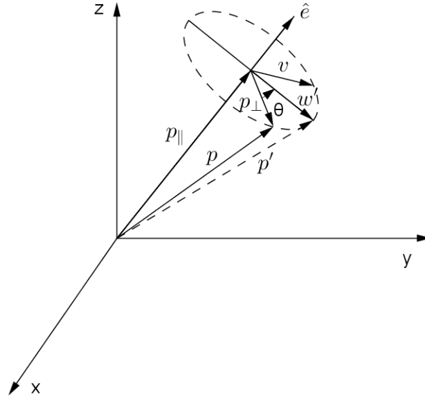
Figura 2.9: Rotação em torno de um eixo qualquer
