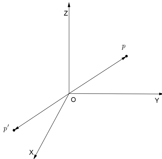
Figura 2.6: Transformação de reflexão no espaço em relação a origem
