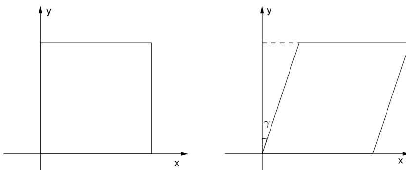
Figura 1.15: Transformação de cisalhamento em x
