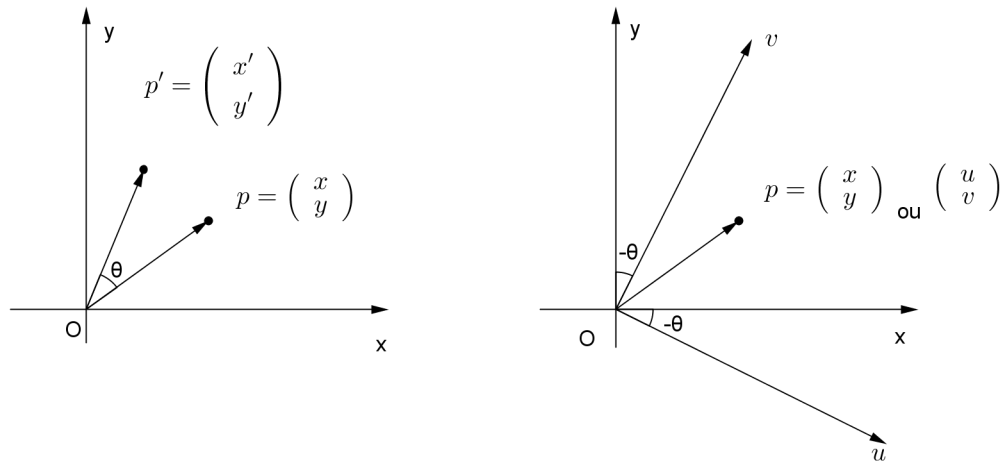
Figura 1.14: Transformação versus mudança de base
