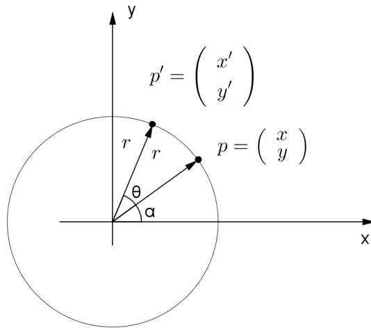
Figura 1.12: Transformação de rotação no \mathbb{R}^2
