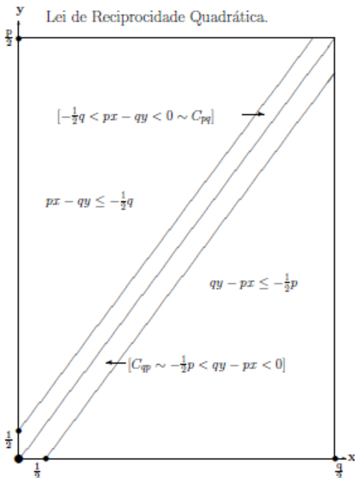
Figura 2.2: O Retângulo R
