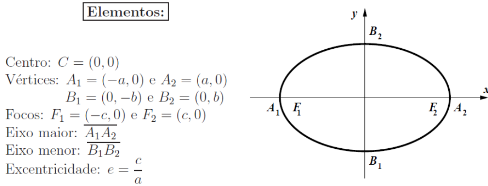
Figura 3.10: Elipse e seus elementos.
