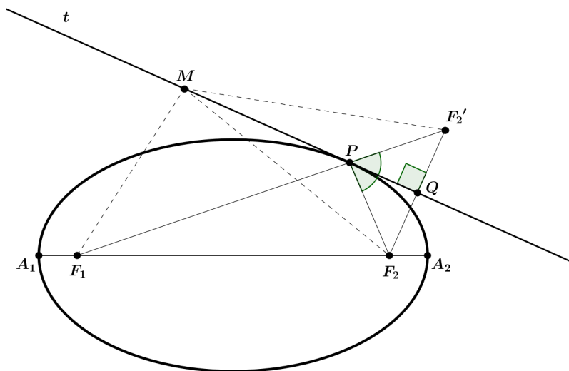
Figura 3.14: Reta tangente à cônica no ponto P .
