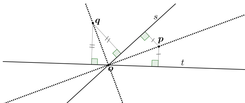
Figura 3.1: Conjunto equidistante a duas retas concorrentes.
