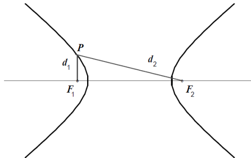
Figura 1.16: Hipérbole com seus focos F_1 e F_2 .
