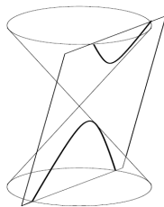
Figura 1.14: Hipérbole.
