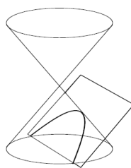
Figura 1.12: Parábola.
