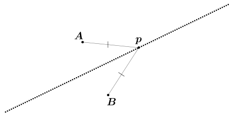
Figura 3.2: Conjunto equidistante a dois pontos.
