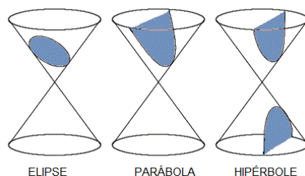
Figura 1: Cônicas
