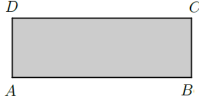
Figura 2.10: Paralelogramo ABCD .
