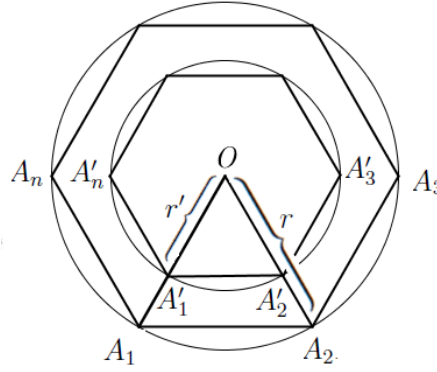
Figura 2.18: Polígono semelhantes.
