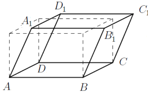
Figura 2.24: Paralelogramo oblíquo.
