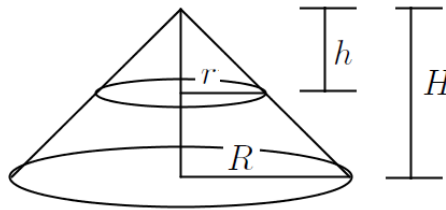
Figura 4.13: Cone.
