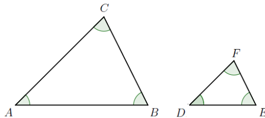
Figura 2.15: Triângulos semelhantes.
