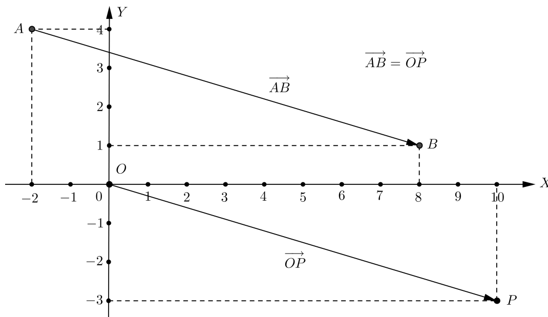
Figura 4.3: Seguintos equipolentes
