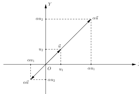
Figura 4.5: Produto \alpha\vec{u} em coordenadas.
