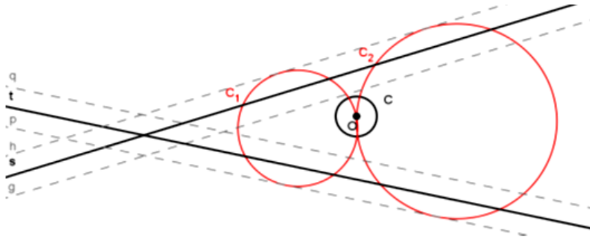
Figura 3.9: Circunferências auxiliares C_1 e C_2
