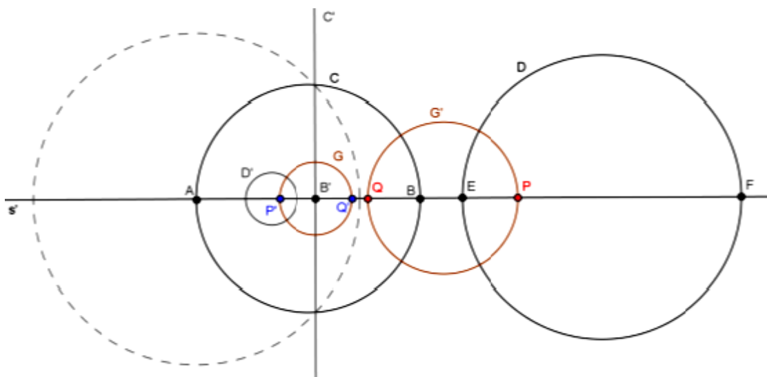
Figura 3.16: Descobrimos P' e Q'
