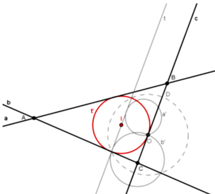
Figura 3.2: Circunferência inscrita no triângulo ABC
