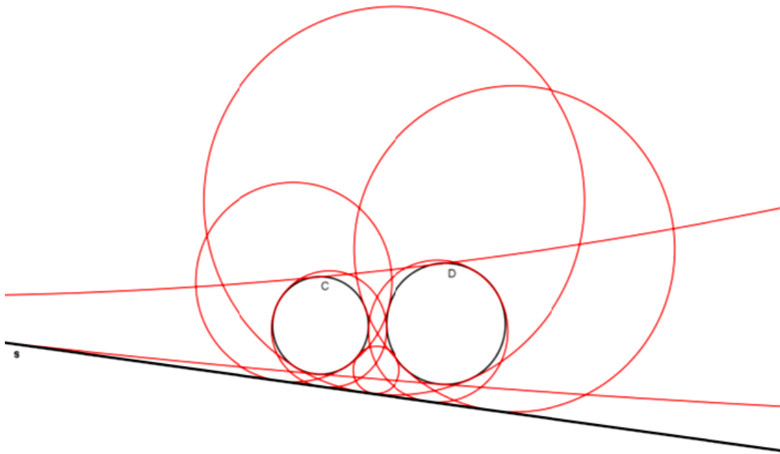
Figura 3.21: Solução do caso RCC
