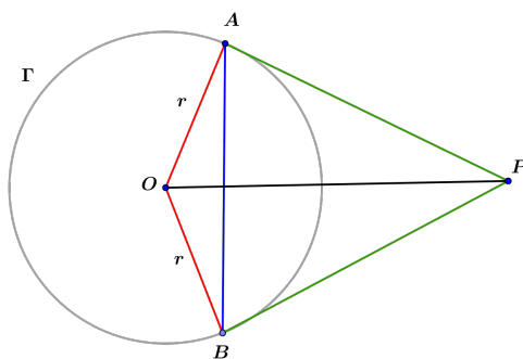
Figura 1.5: Retas tangentes
