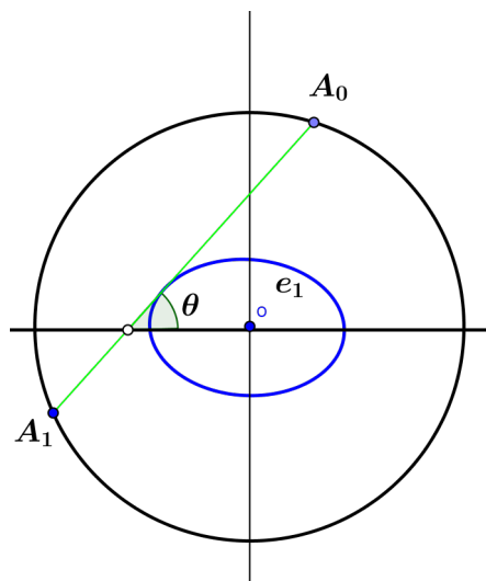
Figura 2.3: Quando A_0A_1 é tangente a e_1 ?
