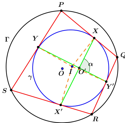
Figura 1.12: Quadrilátero Bicêntrico
