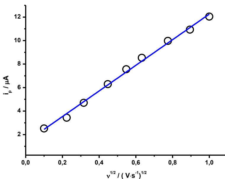
Figura 68 - Relação entre i_p vs. v^{1/2} relativo ao processo a'/a'' do \text{Ni}^{\text{II}} (melofen).
