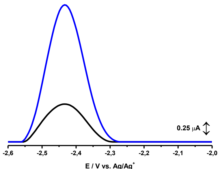
Figura 26 - Voltamogramas de pulso diferencial referente à redução do H_2Cy_2melen antes (preto) e após a adição de um equivalente ácido (azul).
