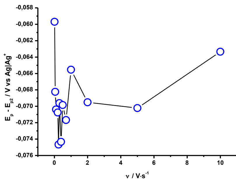
Figura 55 - Comportamento do parâmetro E_p - E_{p1/2} em função de v relativo ao processo B do H_2Cy_2melofen .
