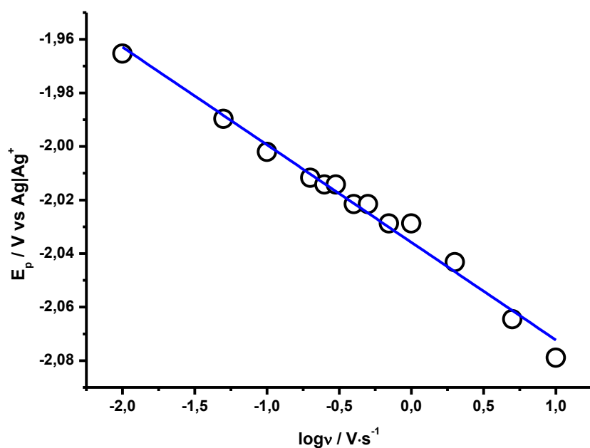
Figura 56 - Relação entre E_p e o logaritmo de v relativo ao processo B do H_2Cy_2melofen .
