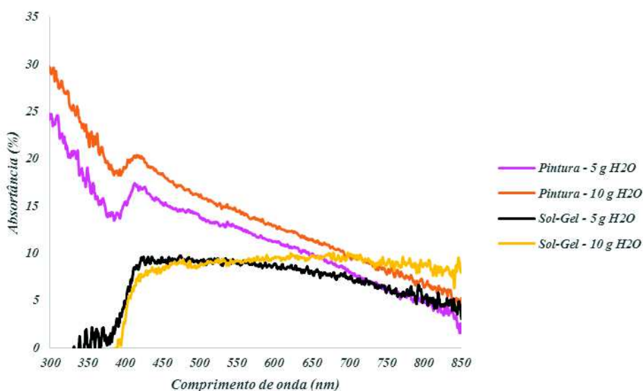
Figura 87. Espectroscopia de Absorptância na faixa do UV-Vis e infravermelho próximo do filme a base de CBC.10.250 depositada em Substrato de Aço Inoxidável.
