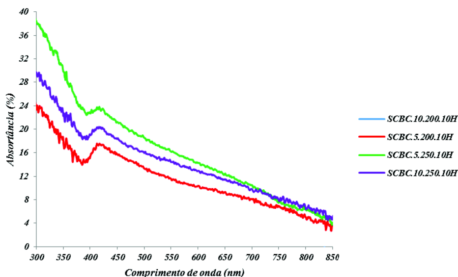
Figura 69. Espectroscopia de Absortância na faixa do UV-Vis e infravermelho próximo do filme depositado pela Técnica de Pintura, utilizando 10 g de H 2 O, em Substrato de Aço Inoxidável.
