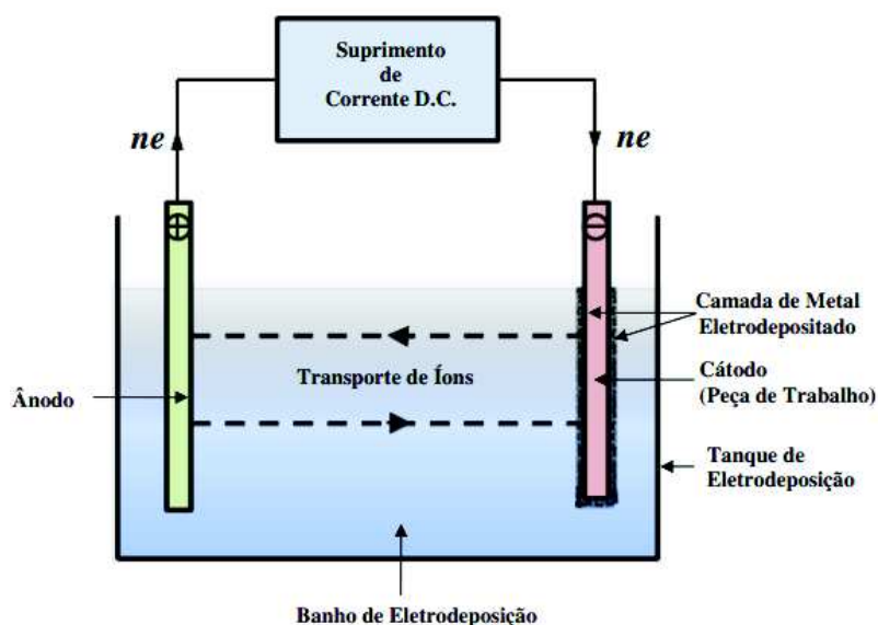
Figura 14. Princípio da Eletrodeposição
