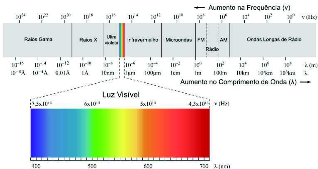
Figura 1. Espectro Eletromagnético.
