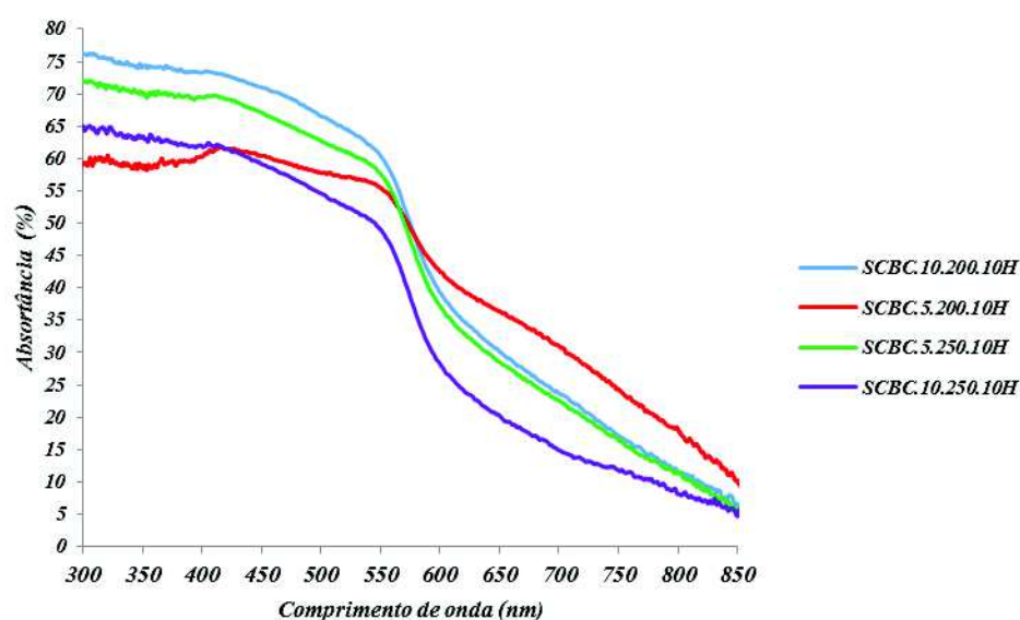
Figura 70. Espectroscopia de Absorância na faixa do UV-Vis e infravermelho próximo do filme depositada pela Técnica de Pintura, utilizando 10 g de H 2 O, em Substrato de Cobre.
