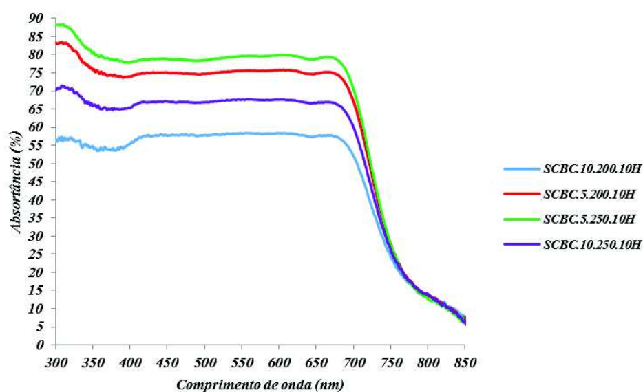
Figura 71. Espectroscopia de Absorância na faixa do UV-Vis e infravermelho próximo do filme depositada pela Técnica de Pintura, utilizando 10 g de H 2 O, em Substrato de Vidro.
